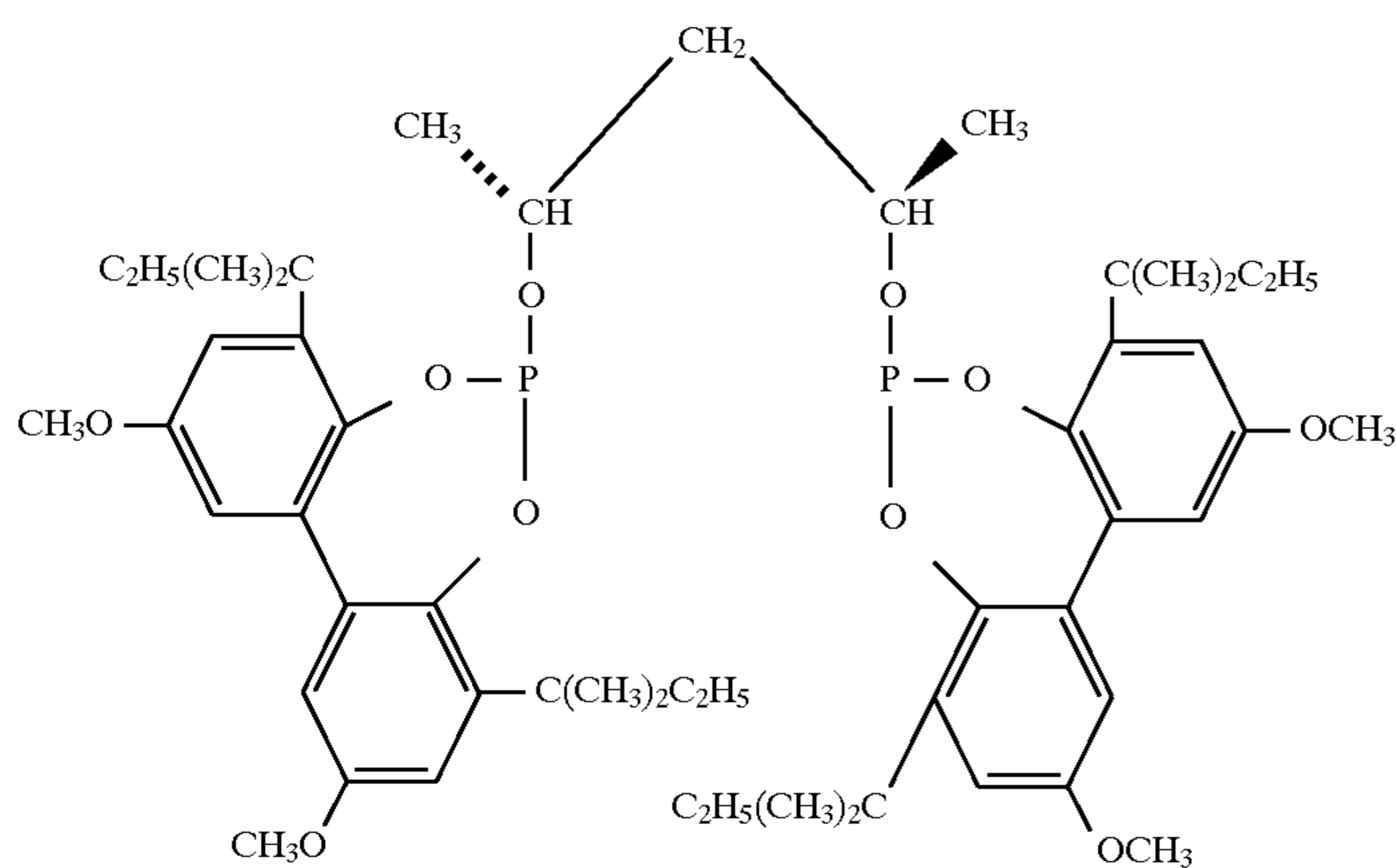
Ligand I
