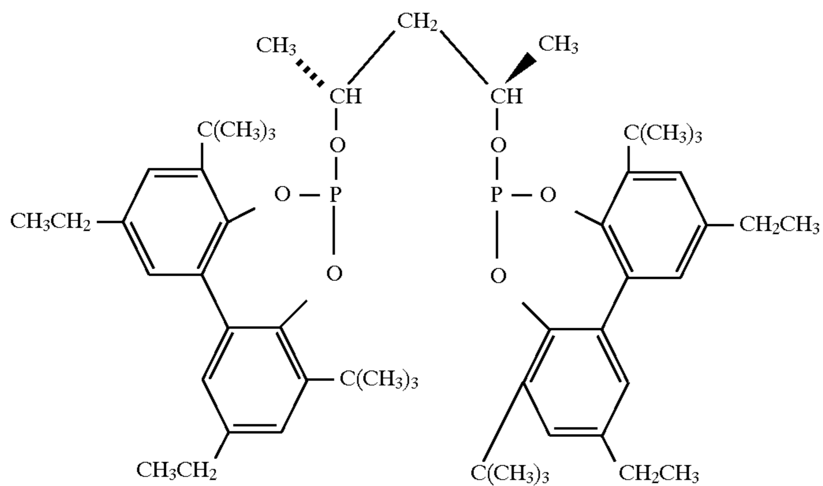
Ligand L
