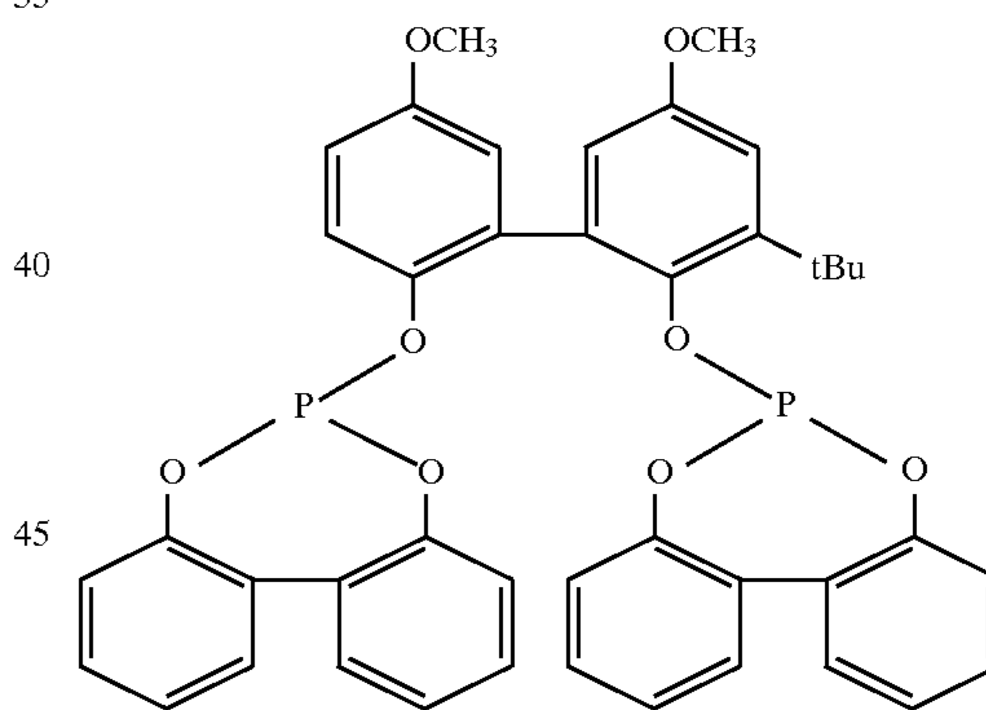
Ligand W
