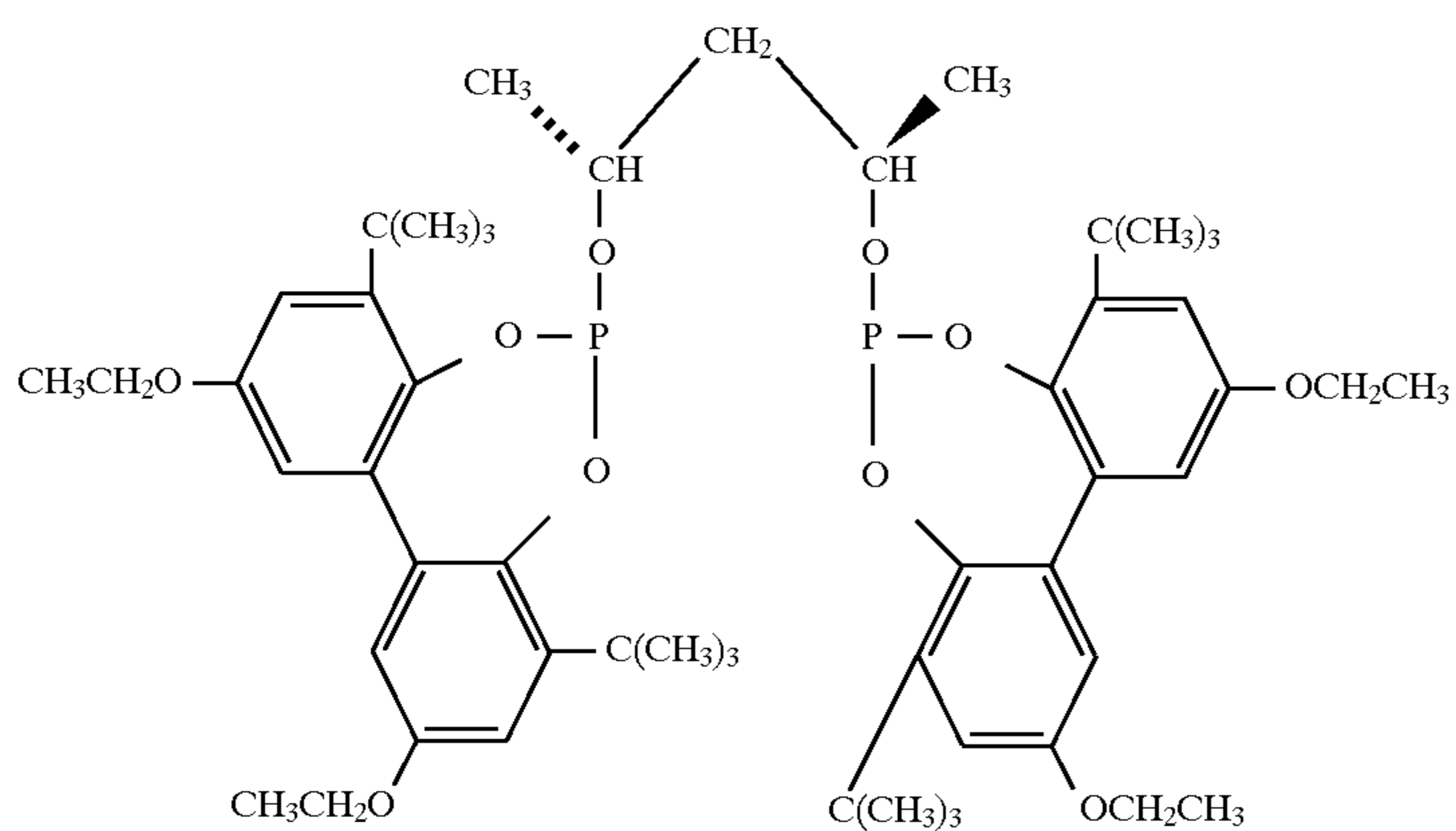
Ligand K
