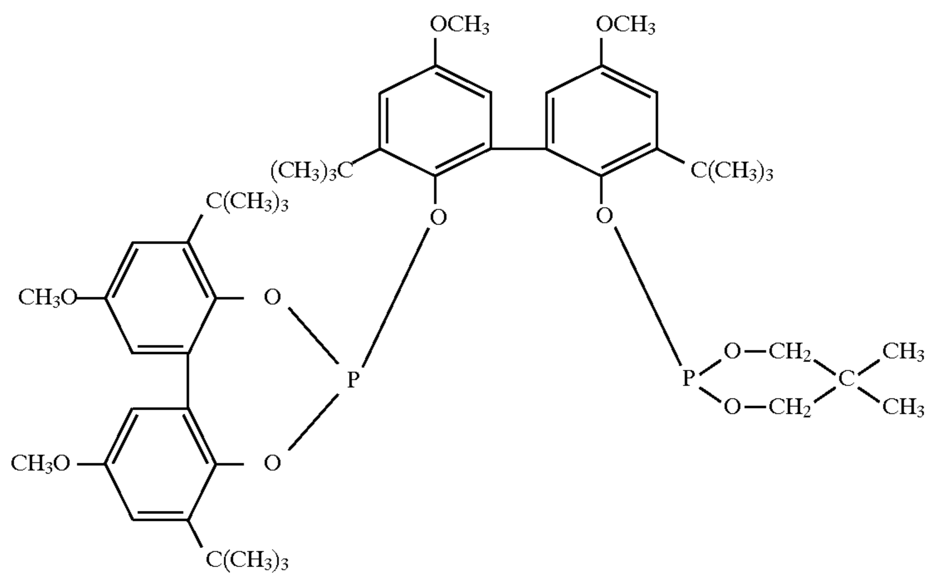
Ligand P
