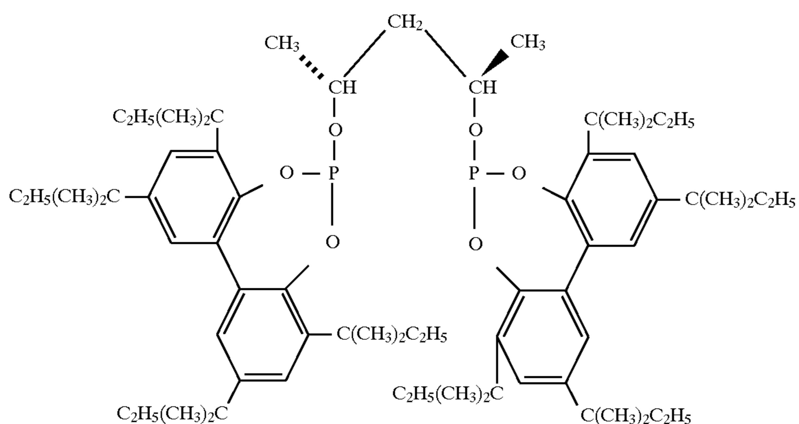
Ligand G
