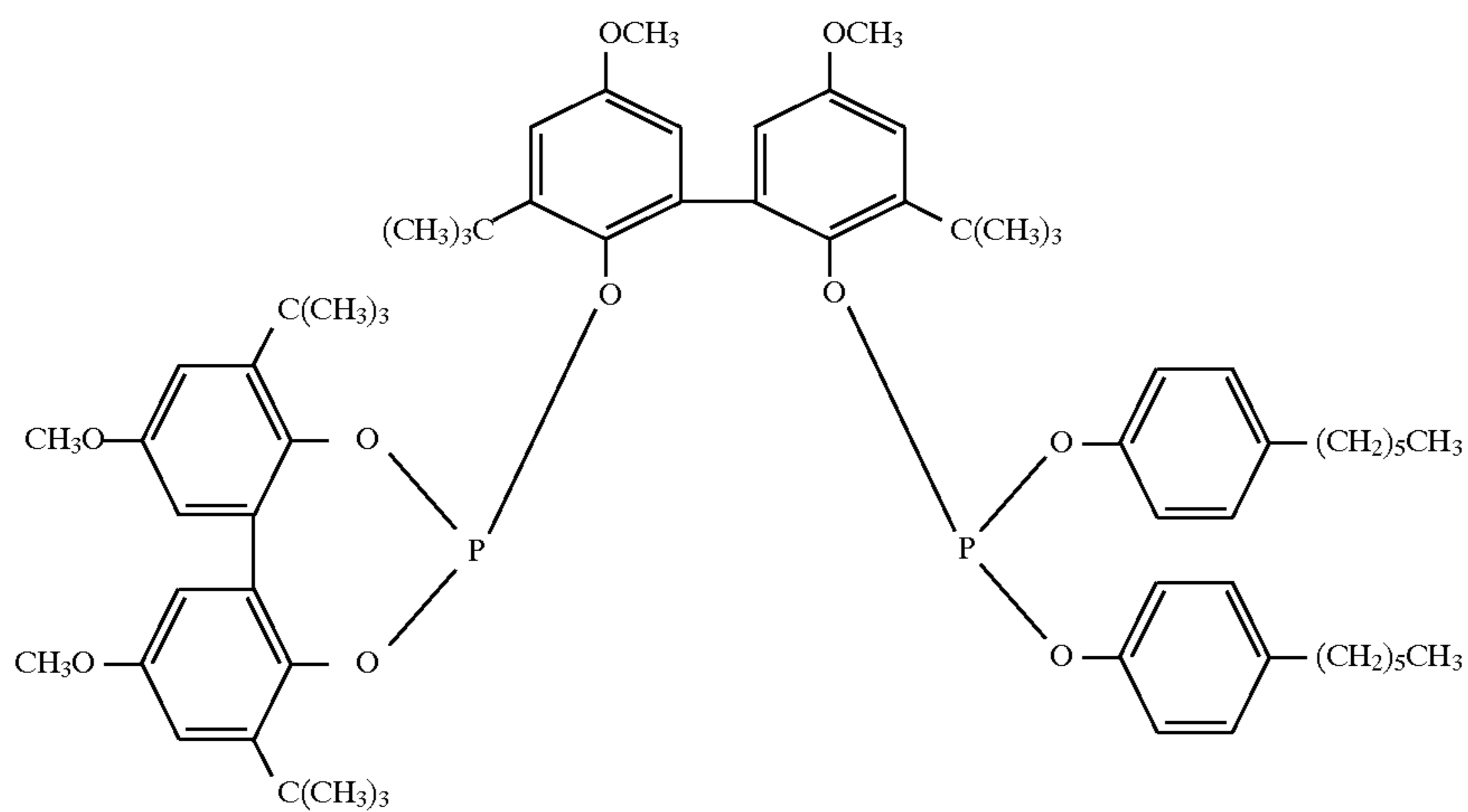
Ligand Q
