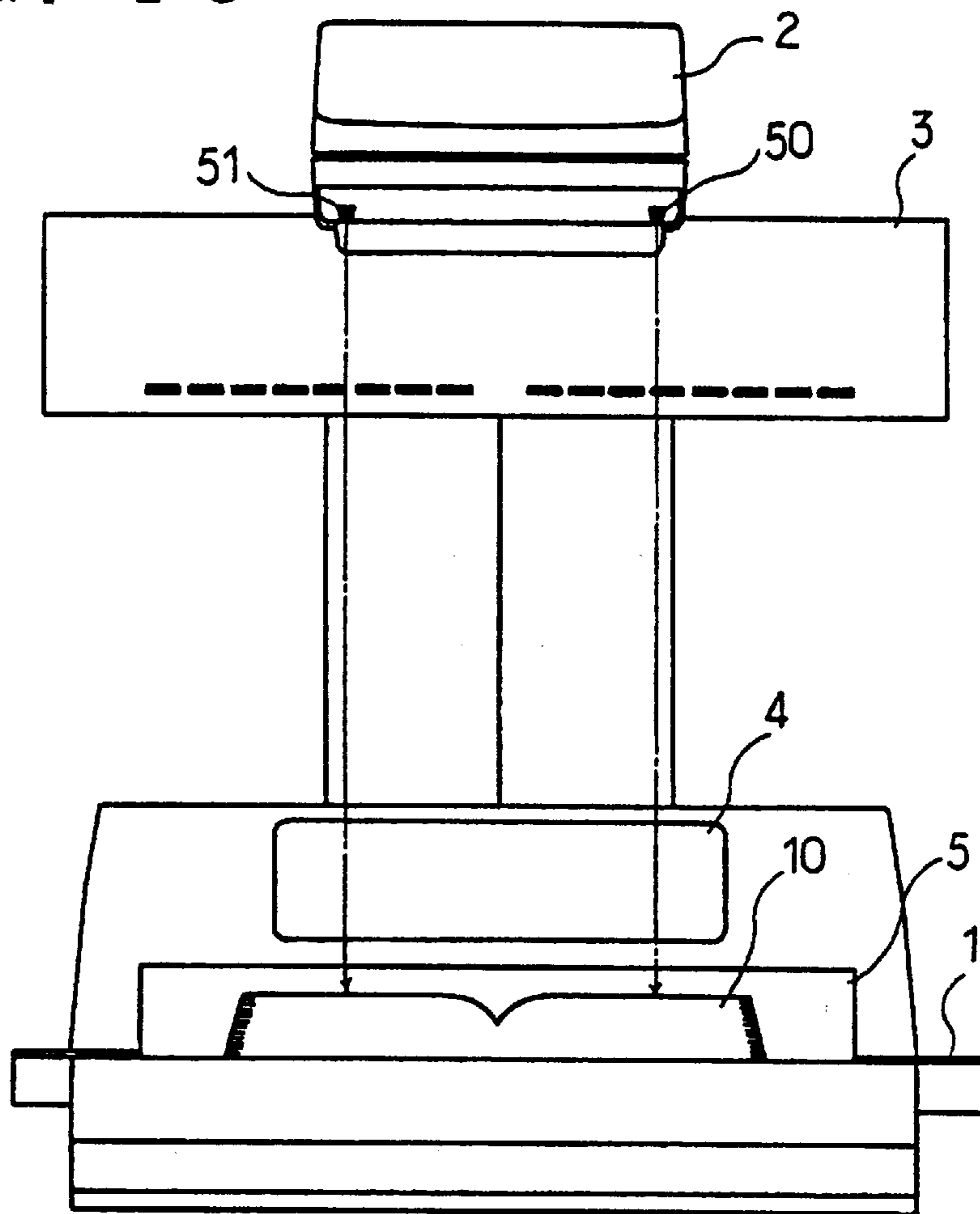
FIG. 15
