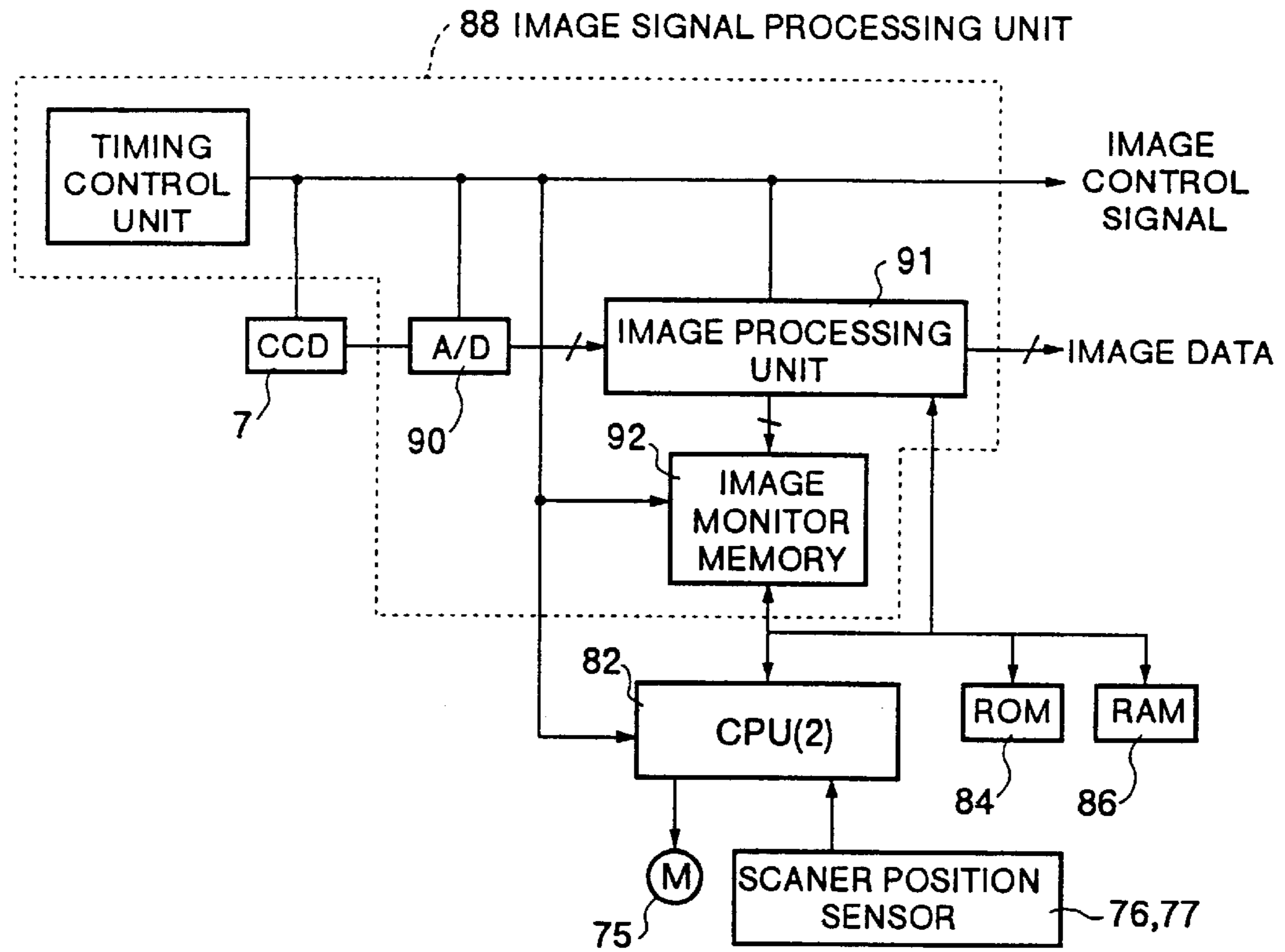
FIG. 31
