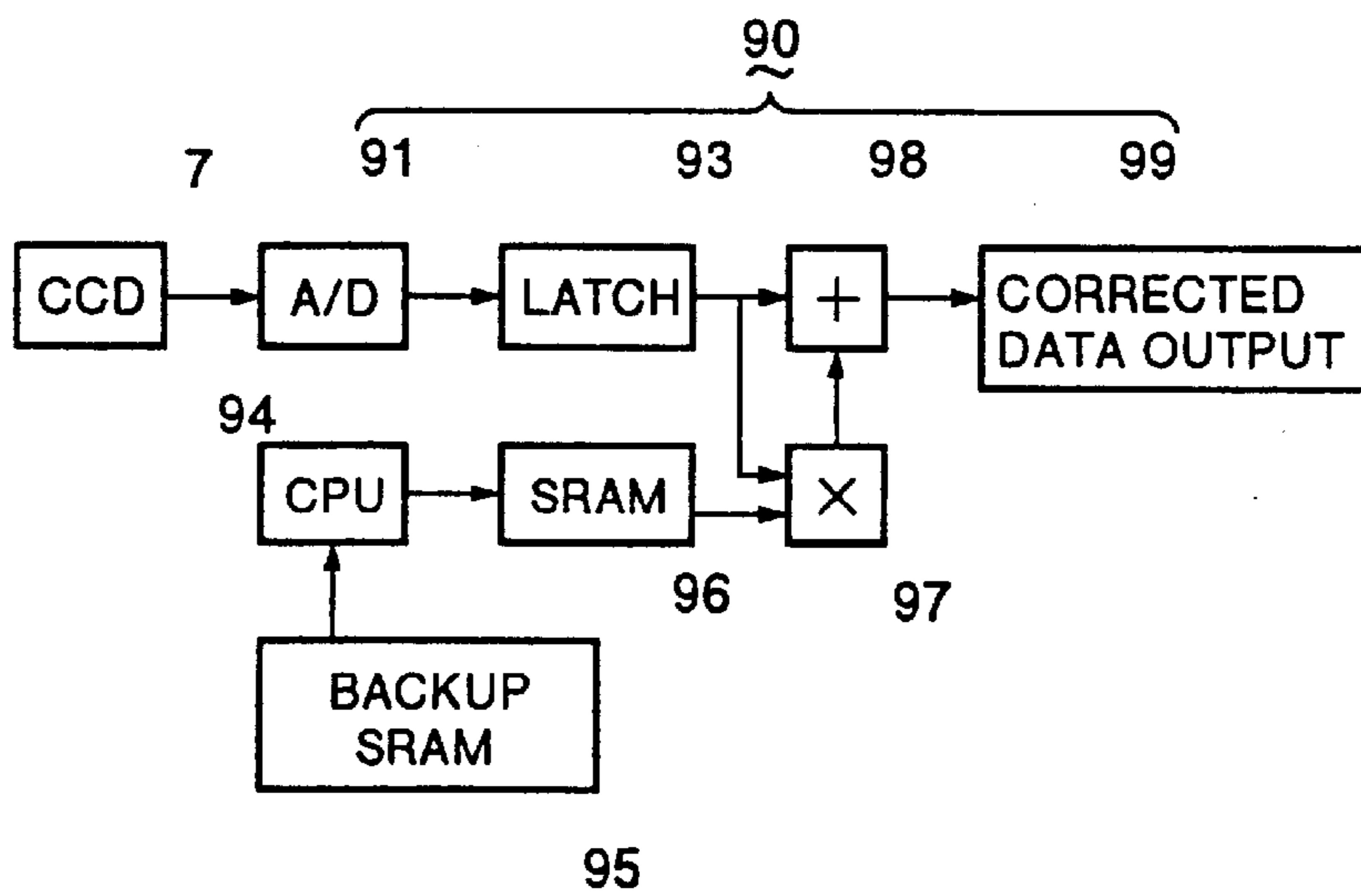
FIG. 39
