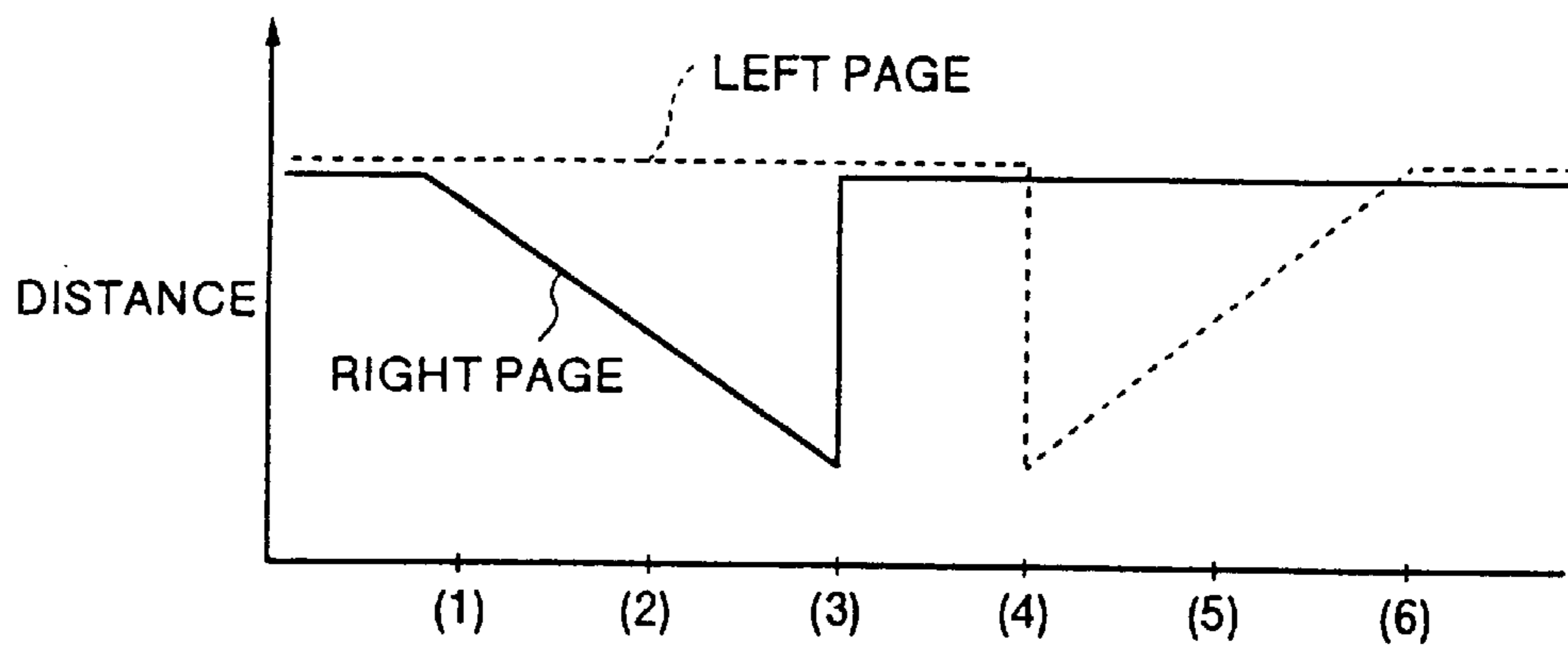
FIG. 18 (b)
