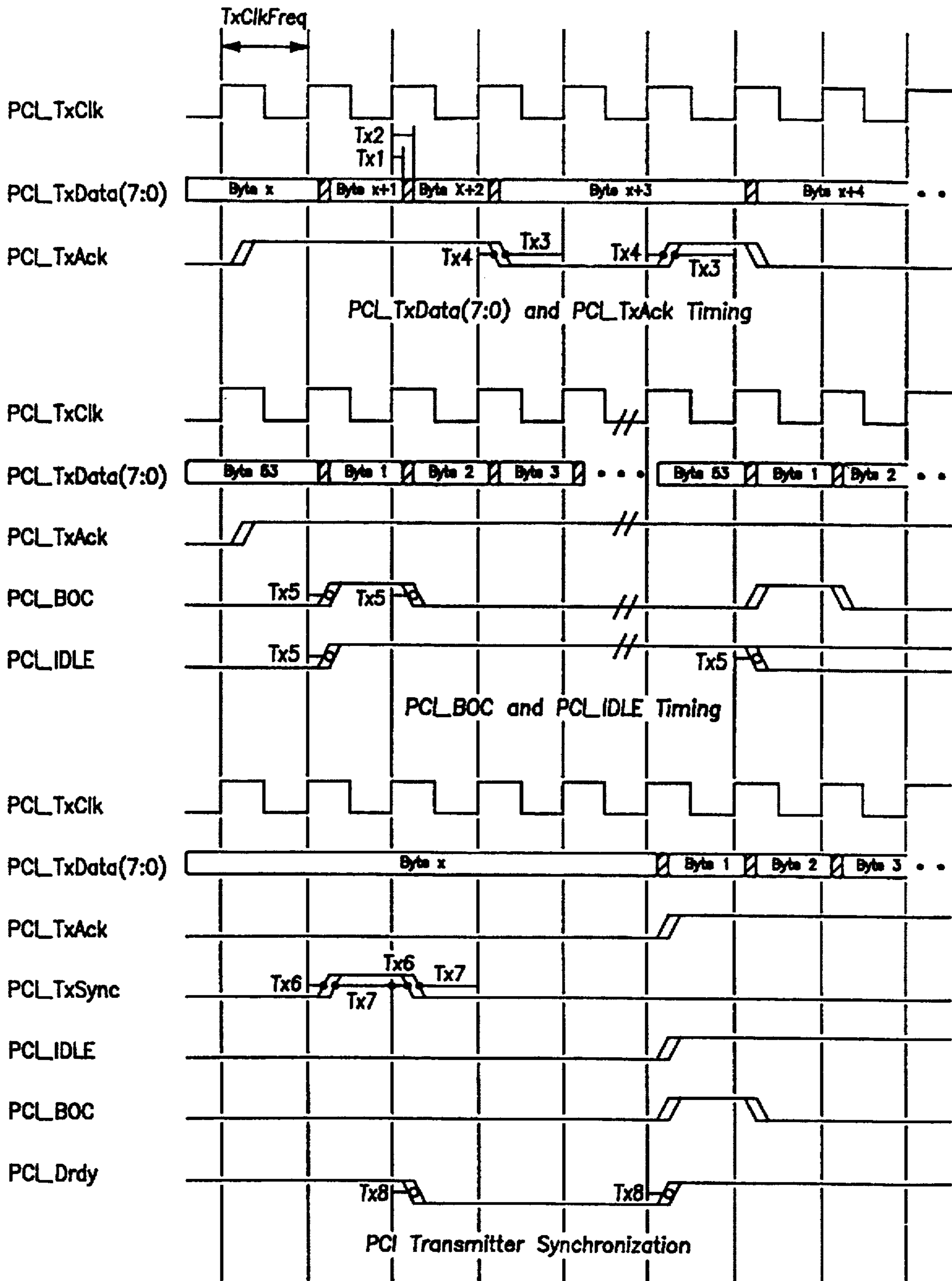
PCI SYNCHRONIZATION FIG. 28C
