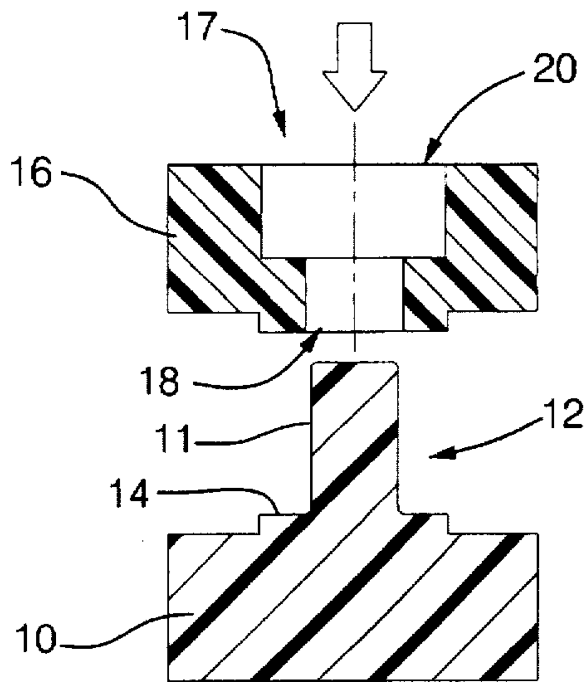
PRIOR ART FIG. 1A
