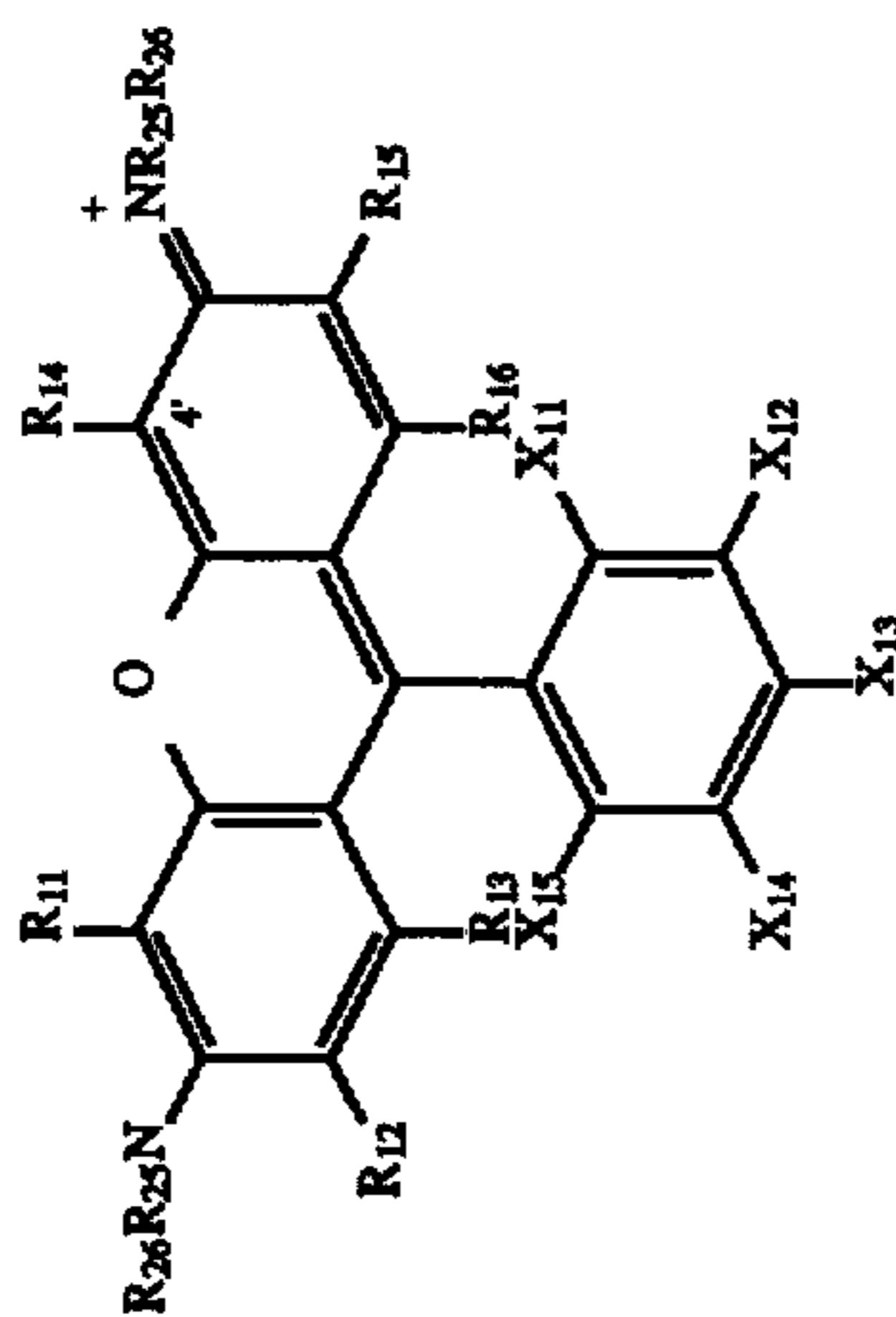
RHODAMINE
