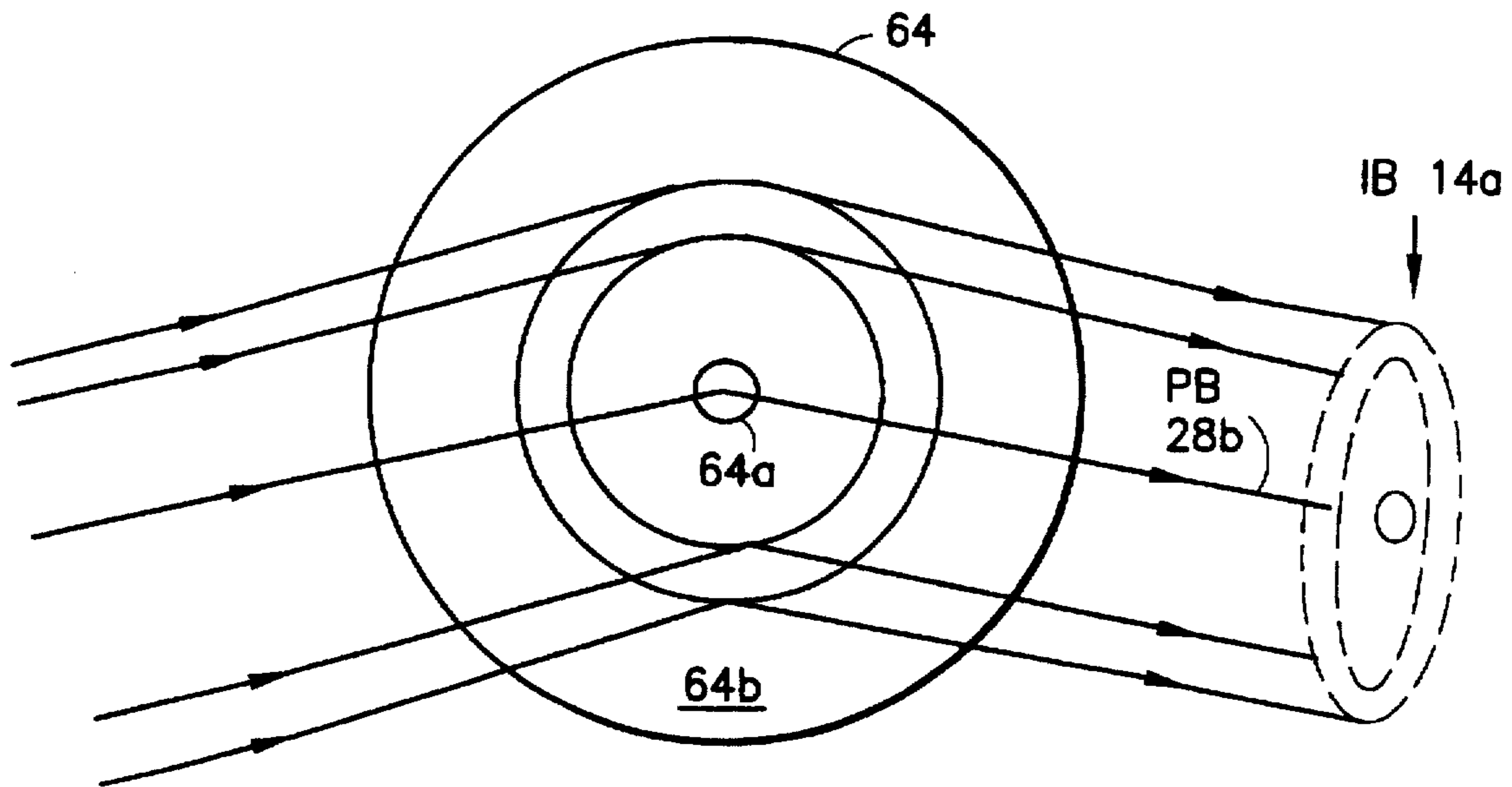
FIG. 8a
