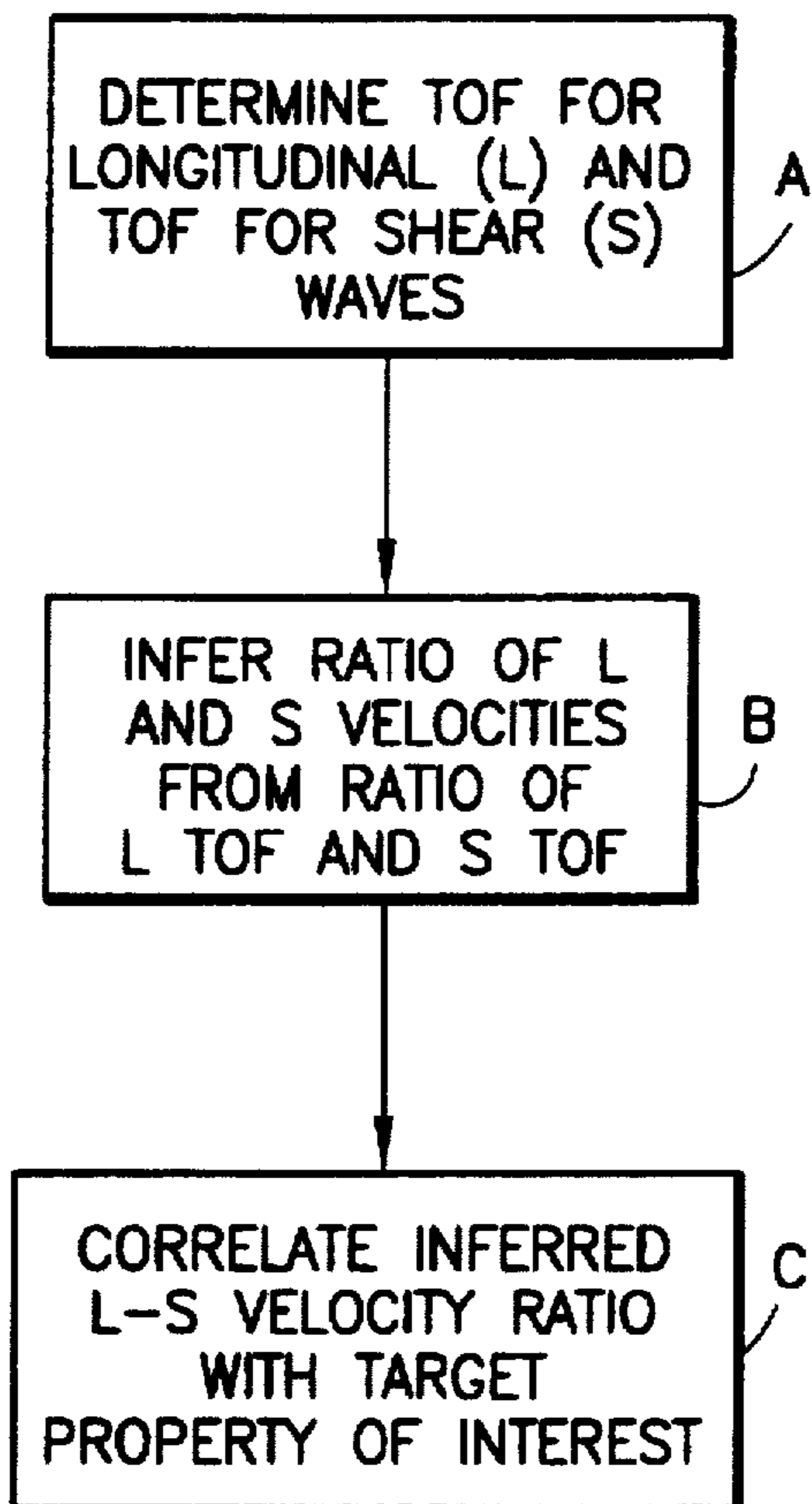
FIG. 17
