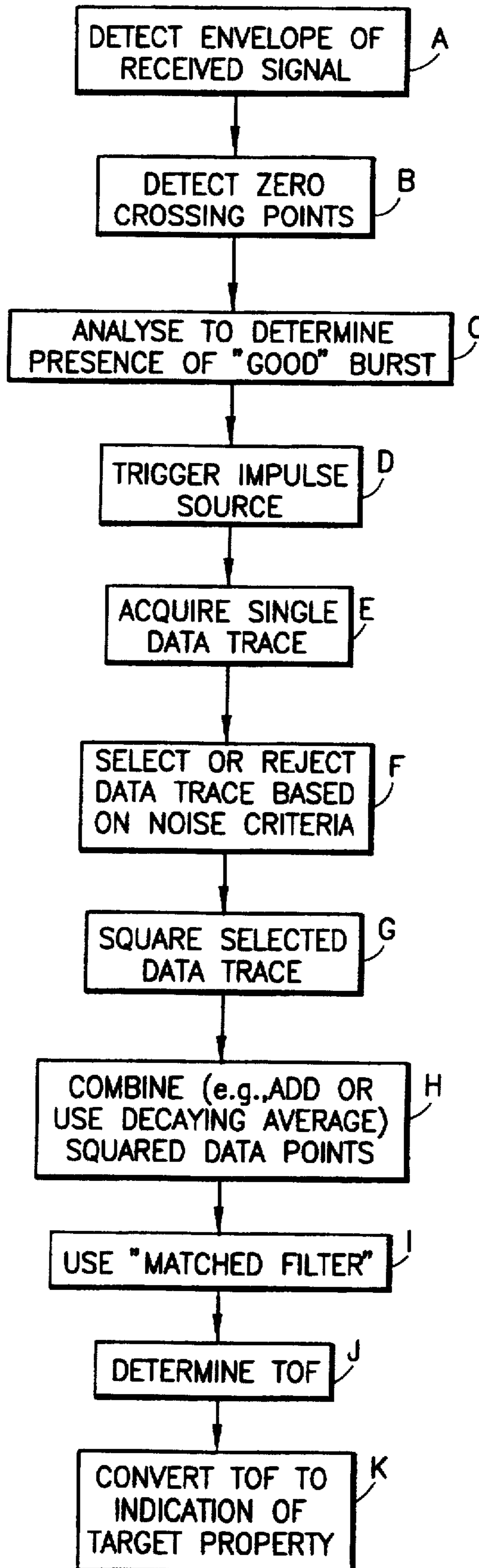
FIG. 14
