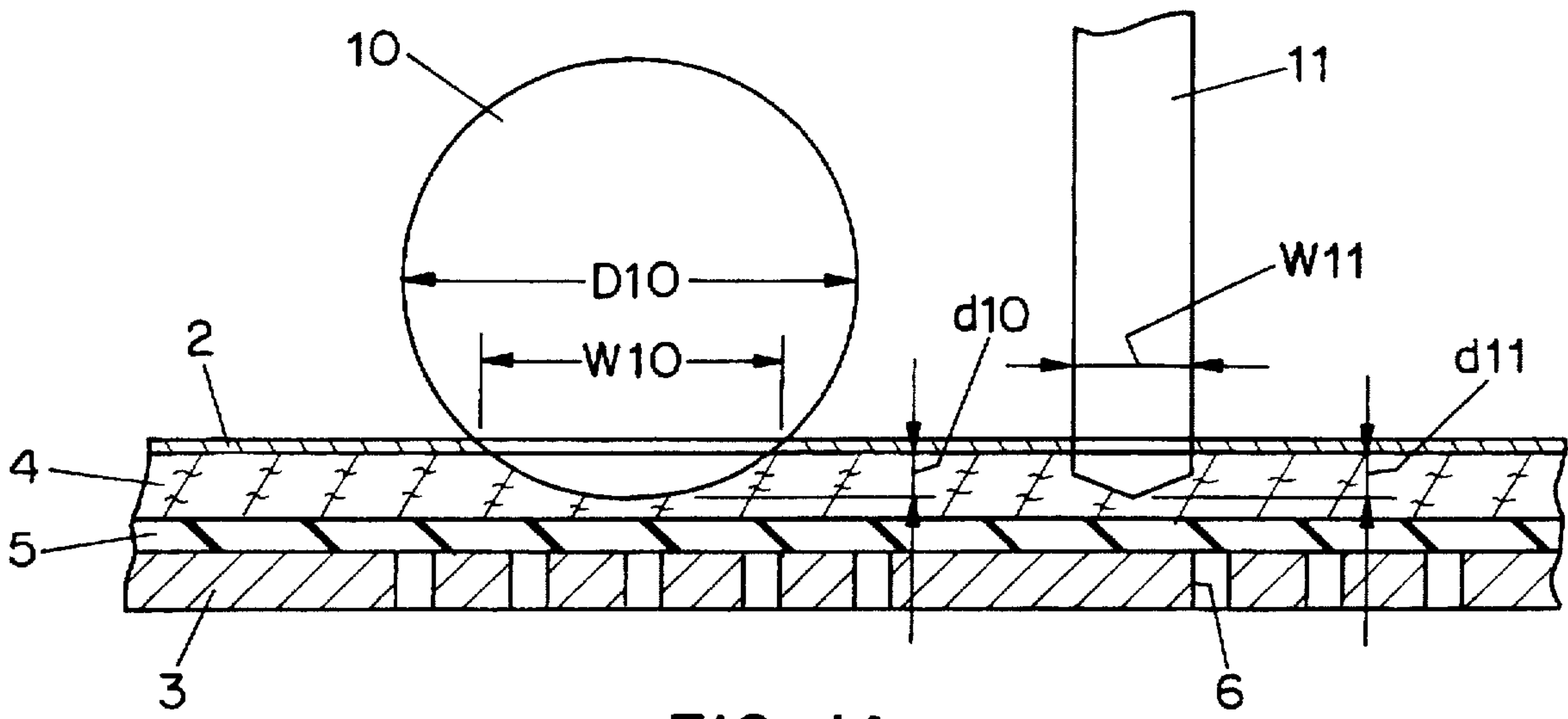
FIG. 1A
