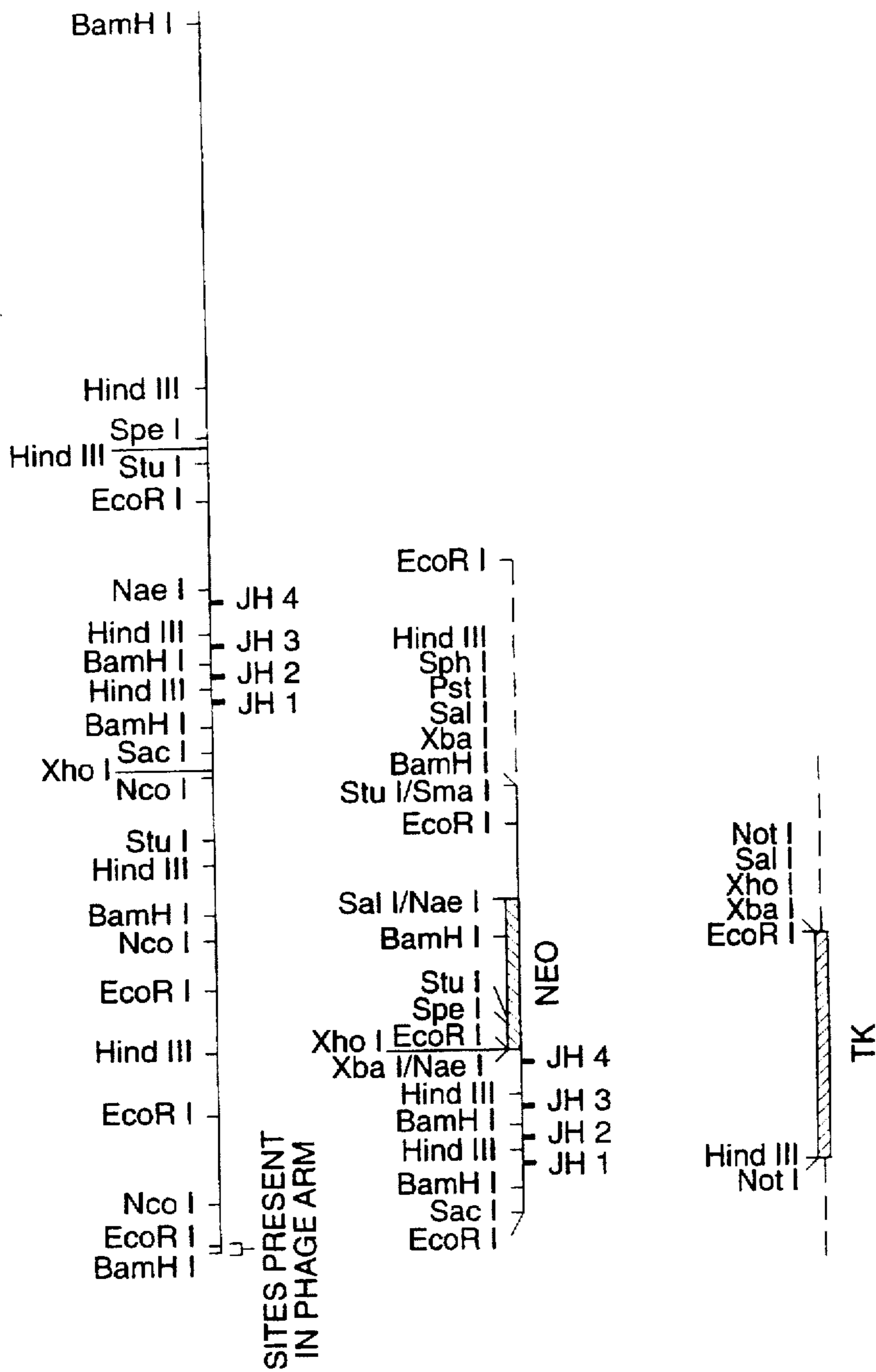
A) GENOMIC J H LOCUS
