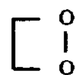
1, 2-dioxetane
