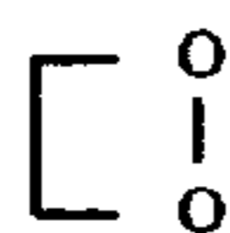
1, 2-dioxetane
