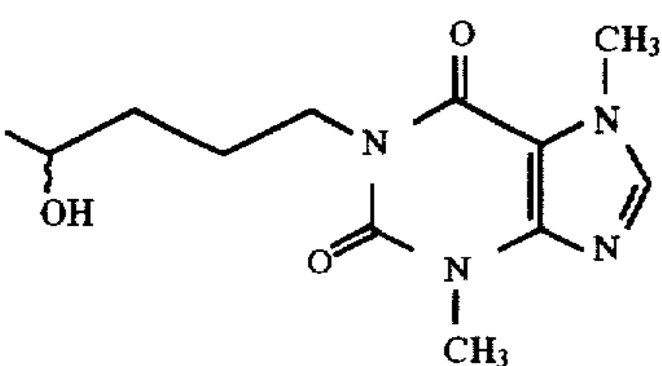
1542 1-(4-Hydroxypentyl)-3,7-dimethylxanthine
