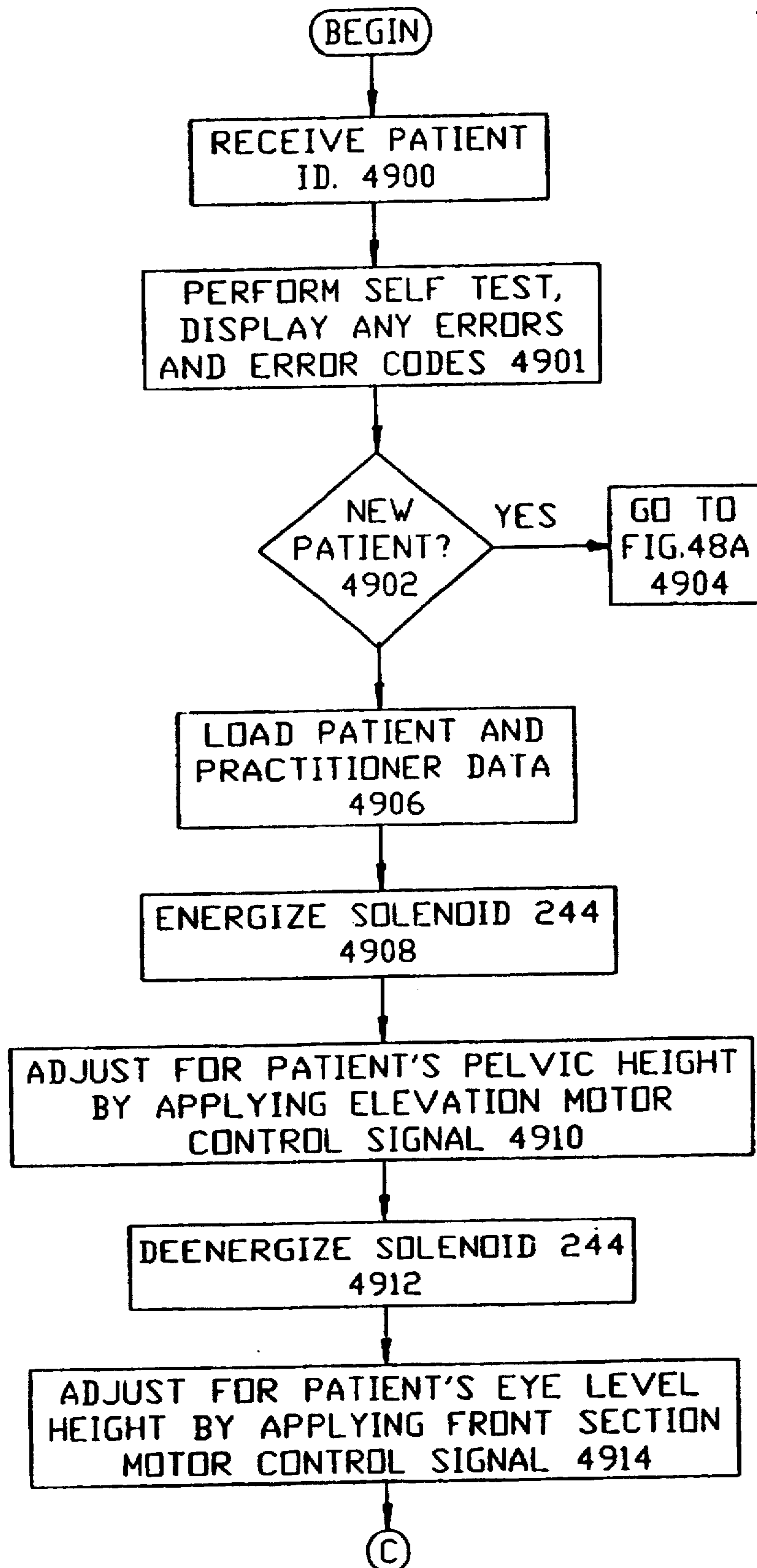
FIG. 49A
