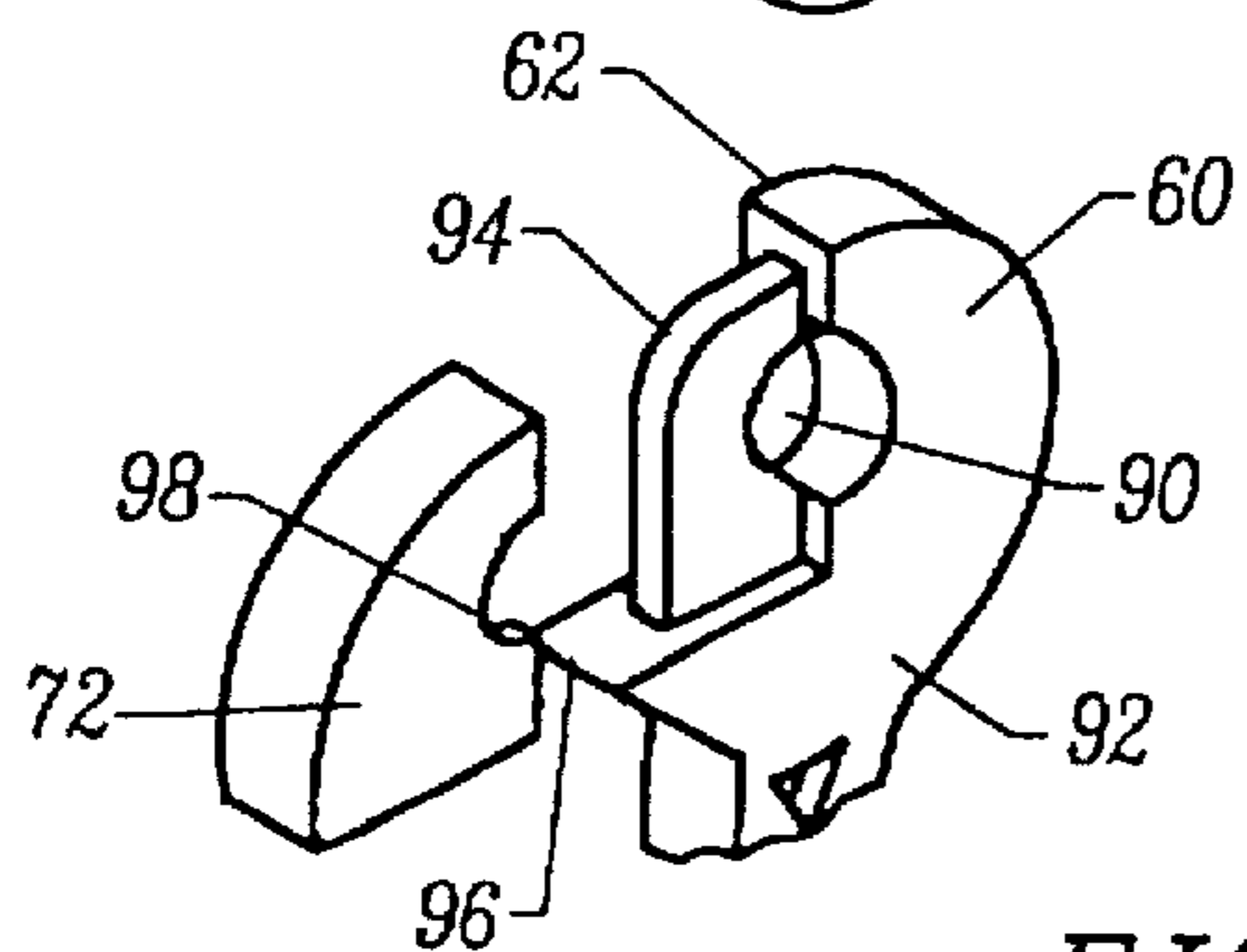
FIG. 3C
