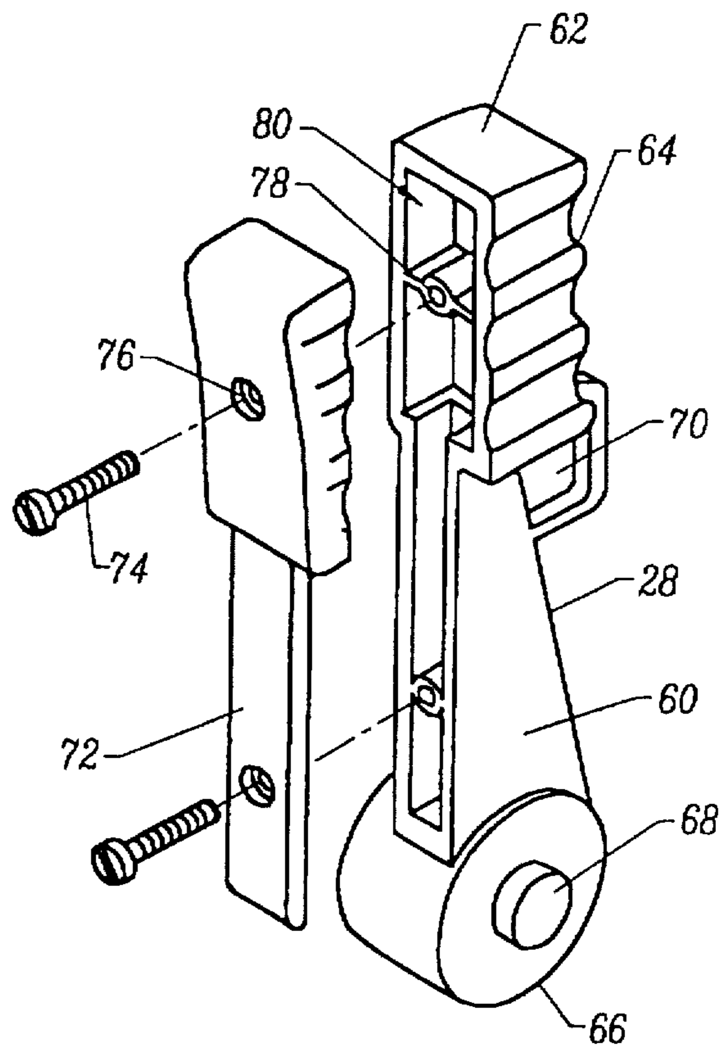
FIG. 3A
