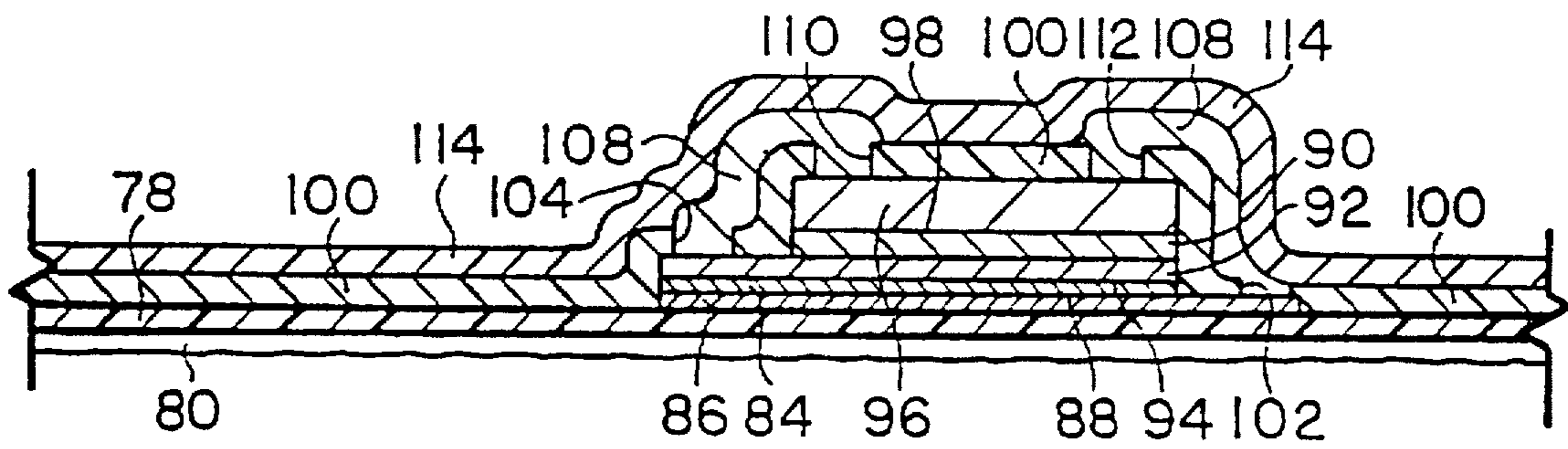
FIG. 6E
