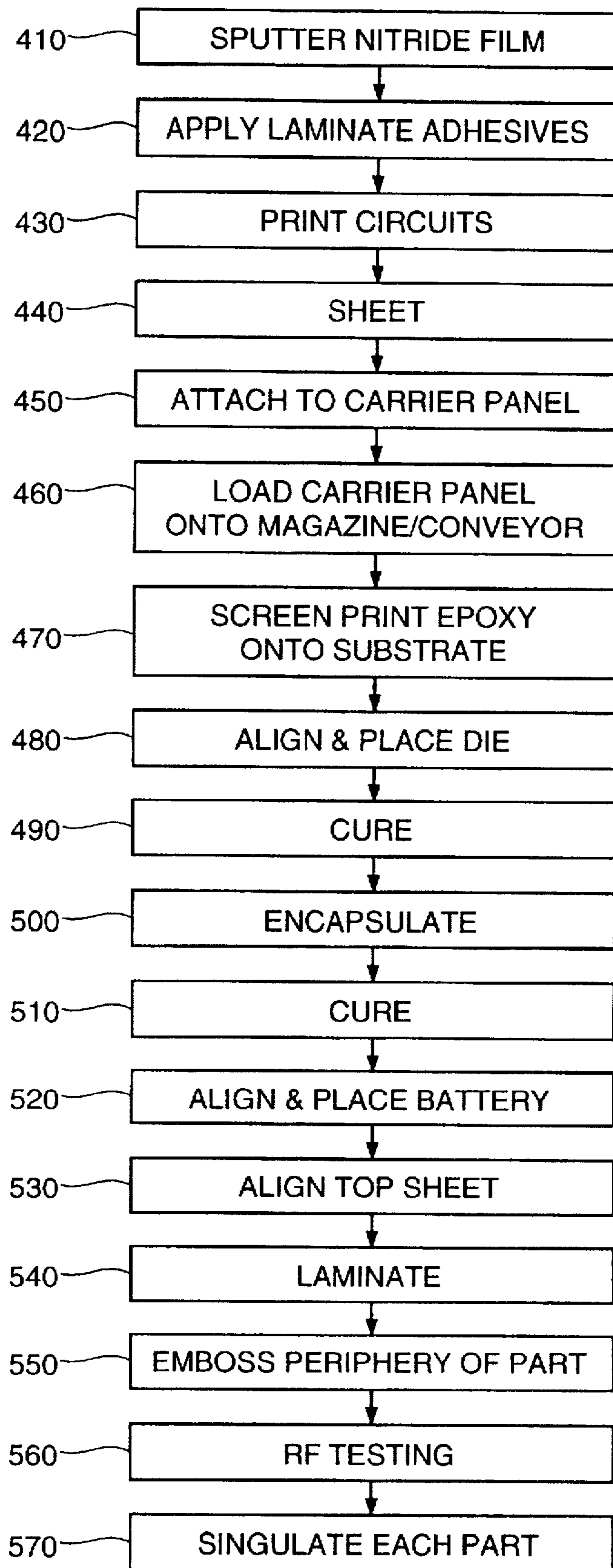
FIG. 13A
