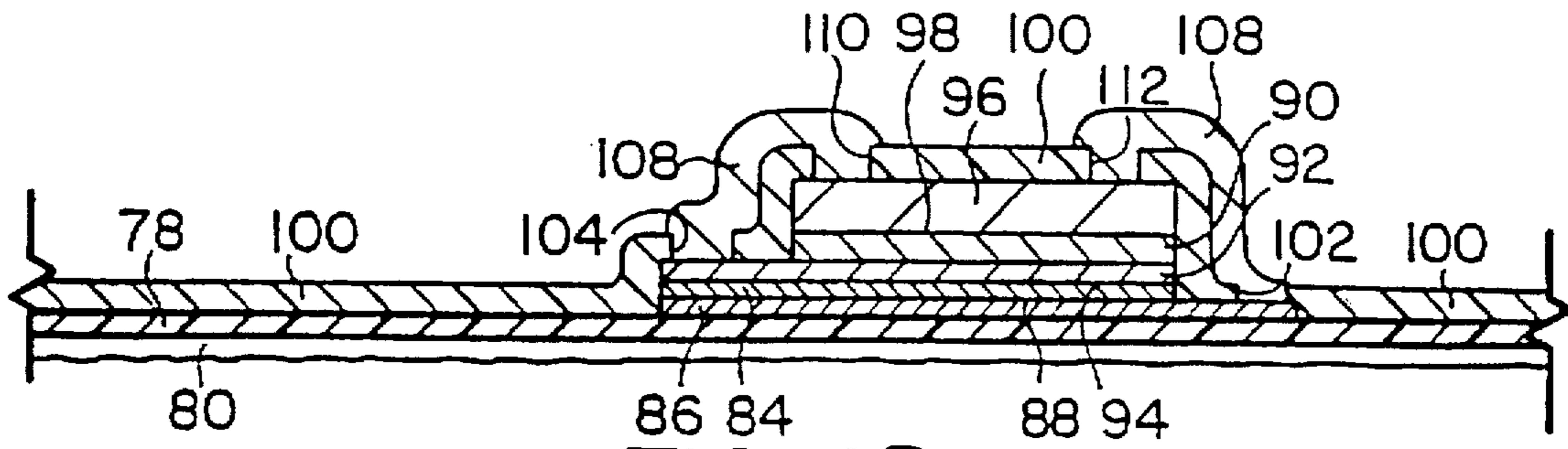
FIG. 6D
