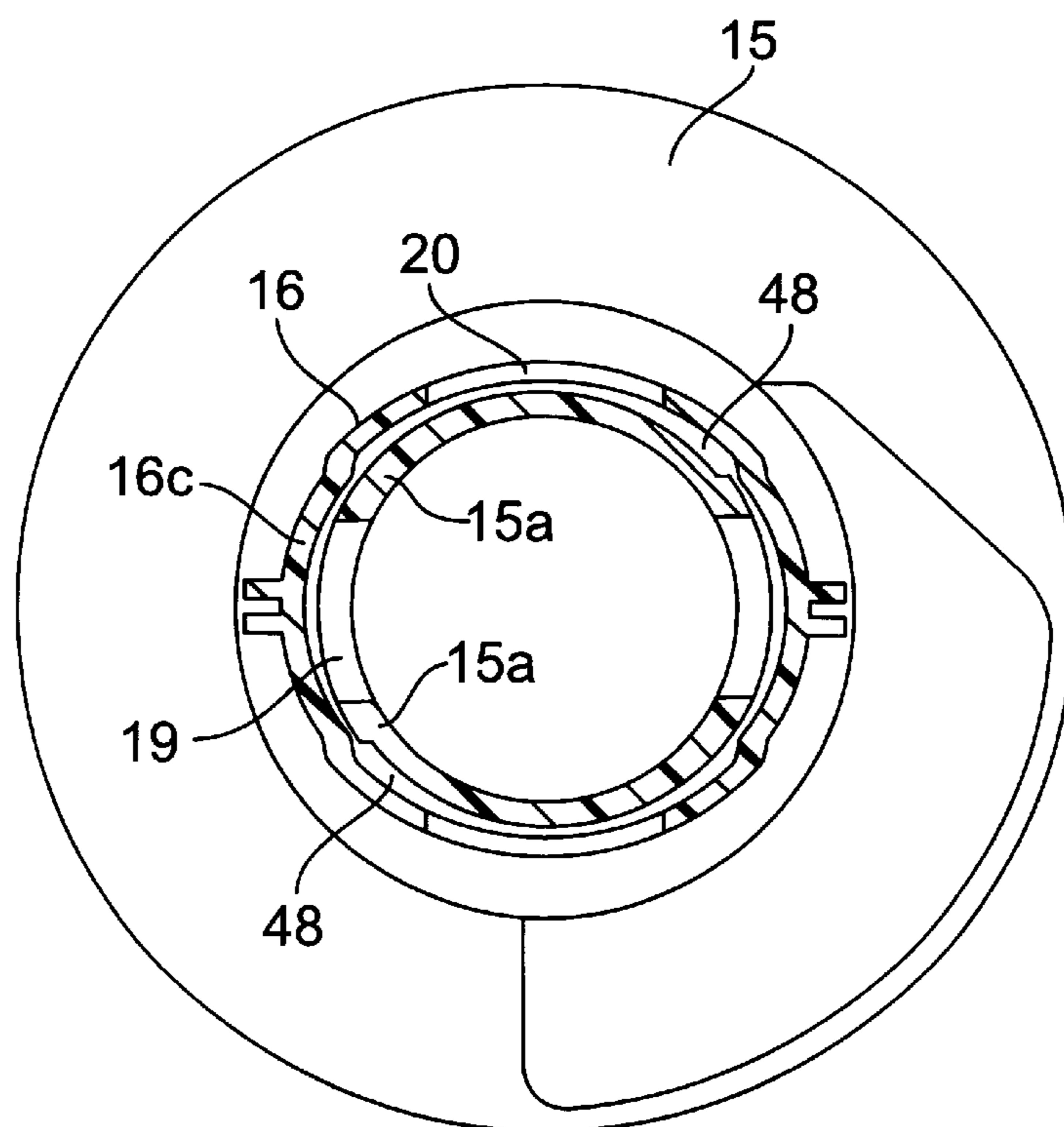
FIG. 9
