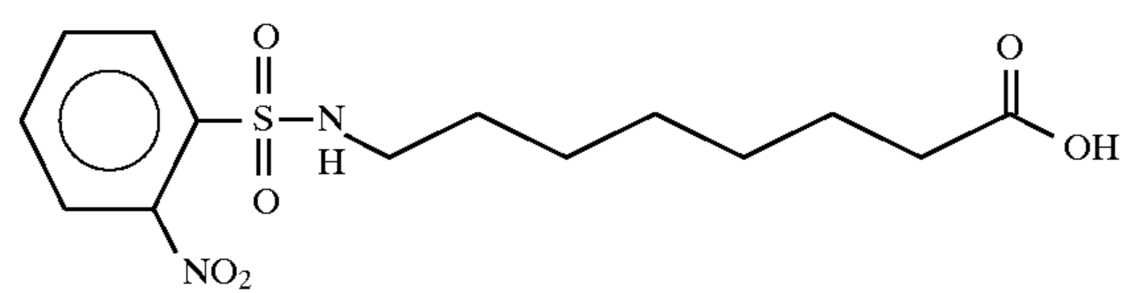
8-(2-nitrobenzenesulfonyl)aminocaprylic acid
