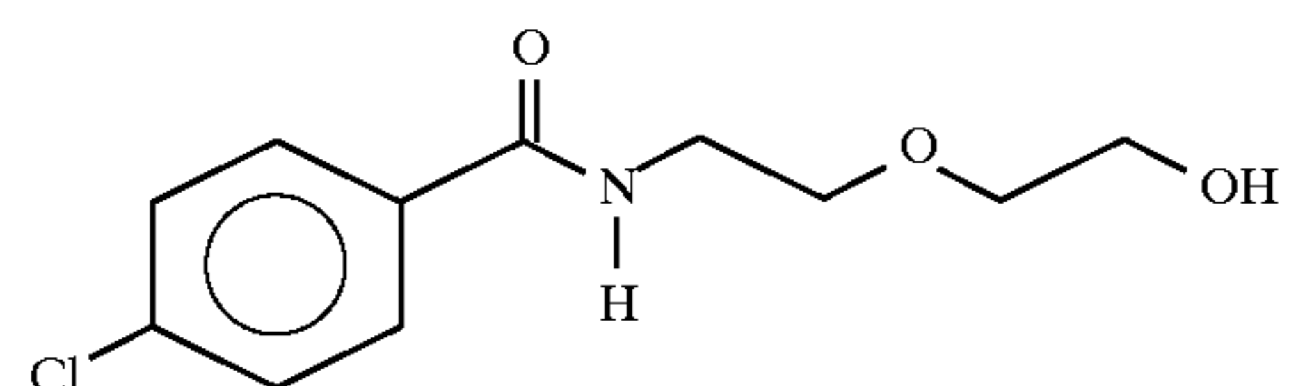
2-[2-N-(4-chlorobenzoyl)aminoethoxy]ethanol
