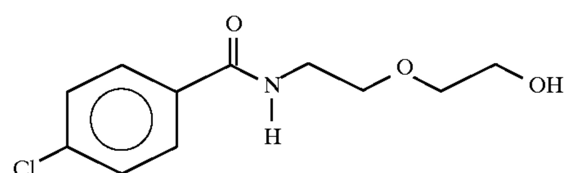
2-[2-N-(4-chlorobenzoyl)aminoethoxy]ethanol
