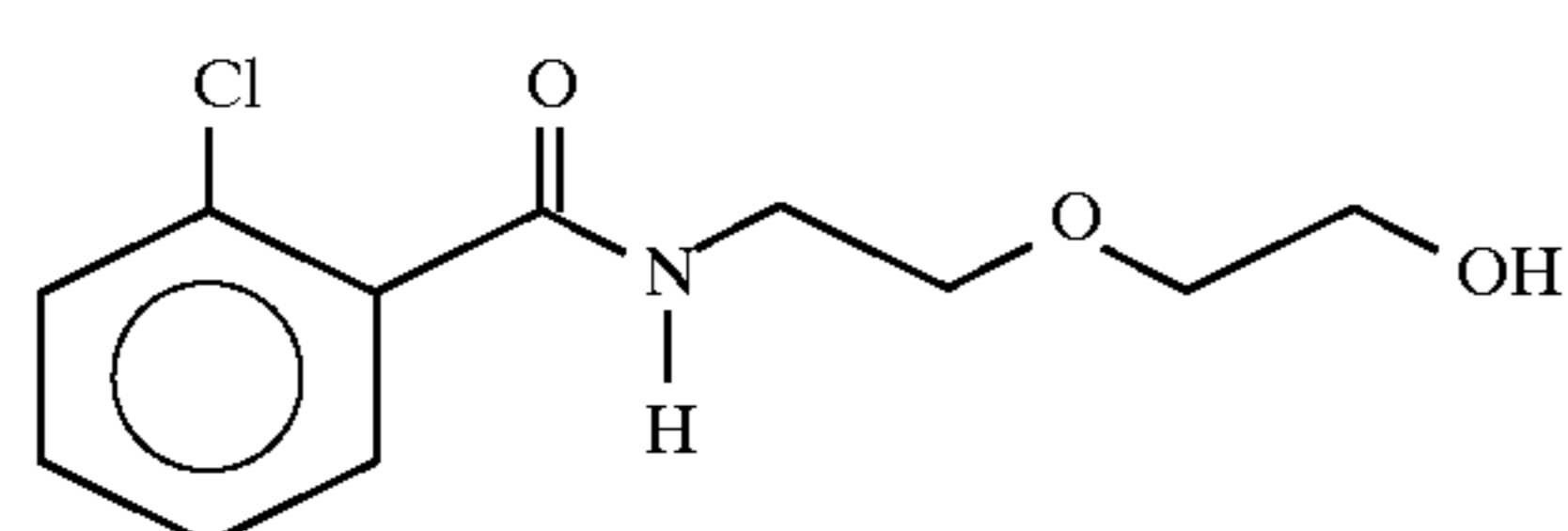
2-[2-N-(2-chlorobenzoyl)aminoethoxy]ethanol
