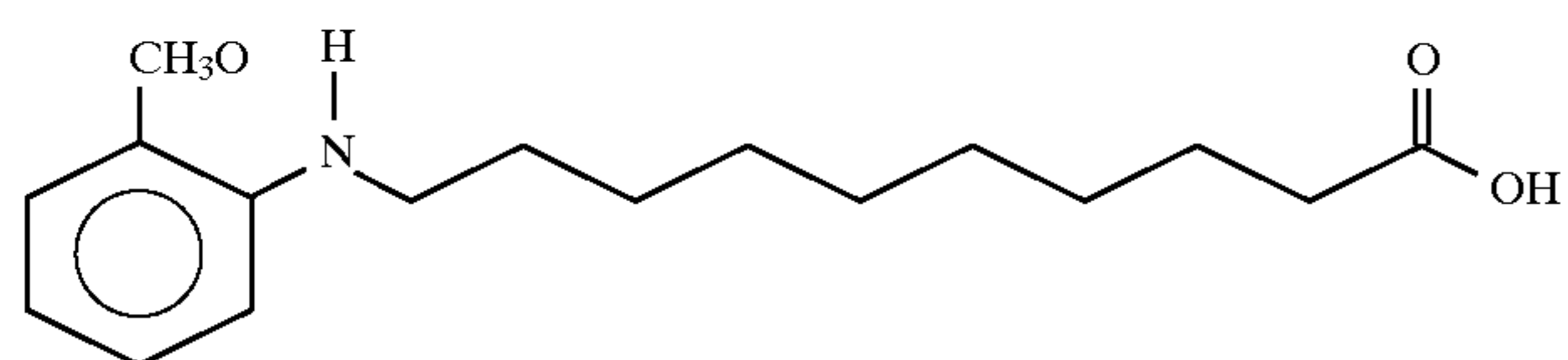
2-ethoxybenzenenaminodecanoic acid
