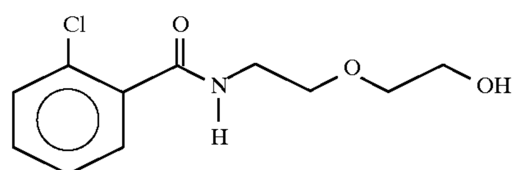
2-[2-N-(2-chlorobenzoyl)aminoethoxy]ethanol
