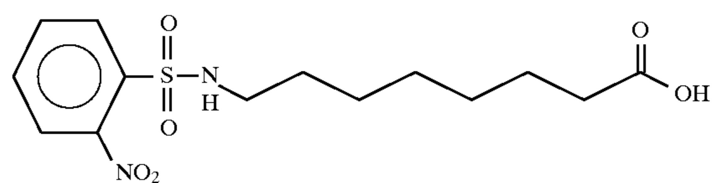
8-(2-nitrobenzenesulfonyl)aminocaprylic acid
