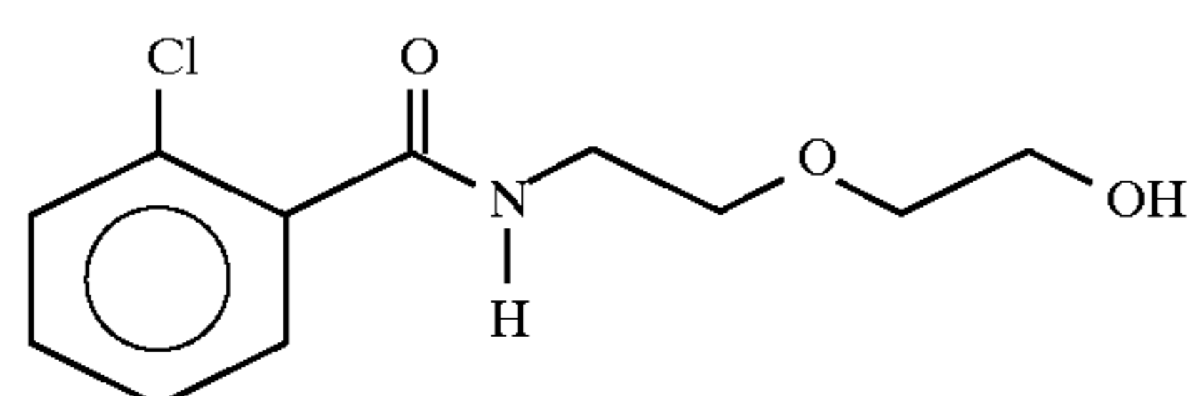
2-[2-N-(2-chlorobenzoyl)aminoethoxy]ethanol
