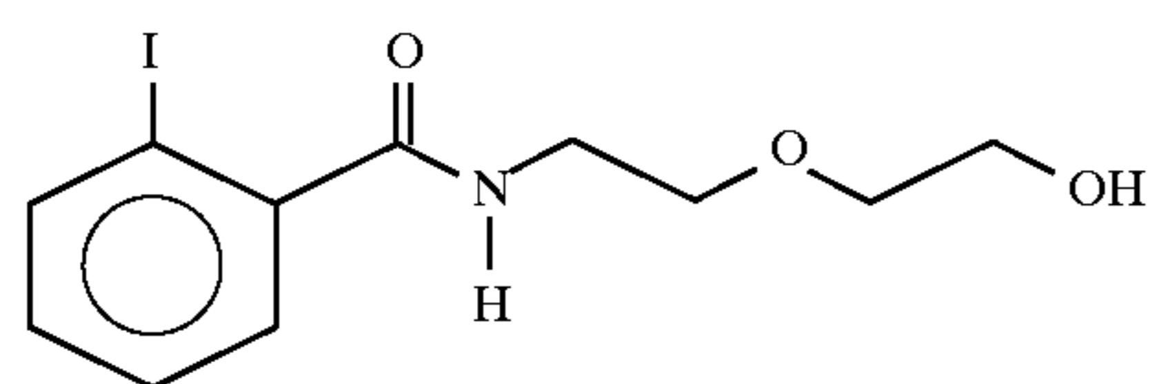
2-[N-(2-iodobenzoyl)aminoethoxy]ethanol
