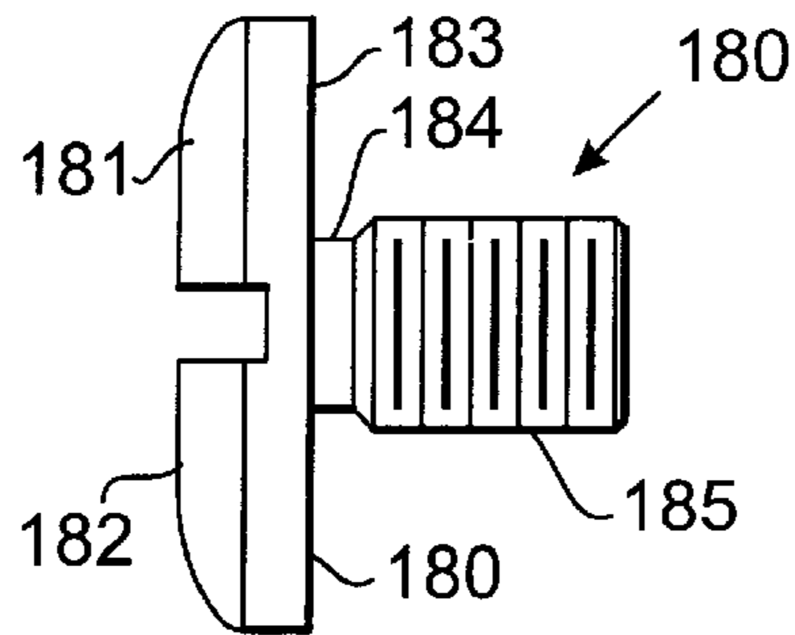
Fig. 38
