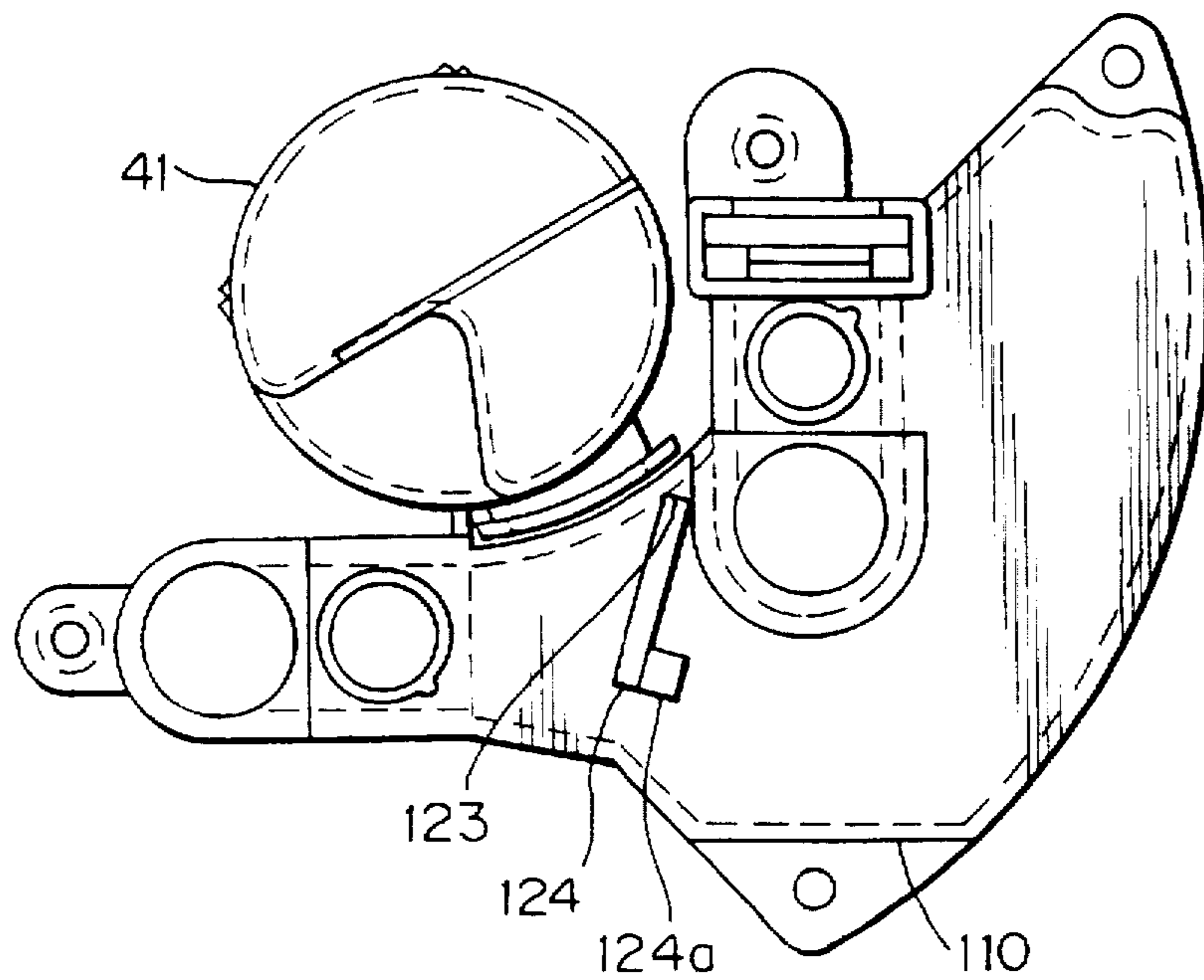
Fig. 11B
