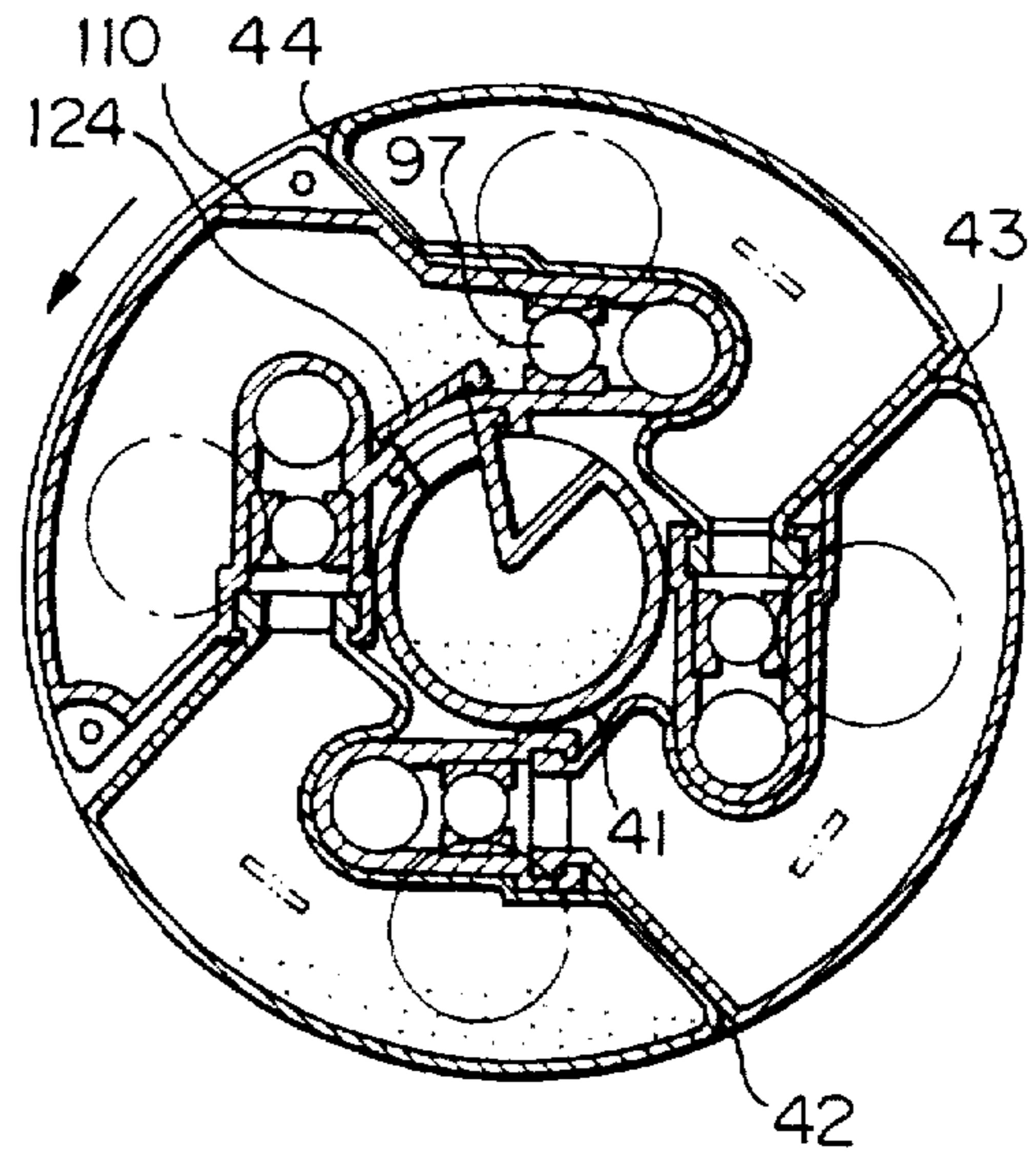
Fig. 15D
