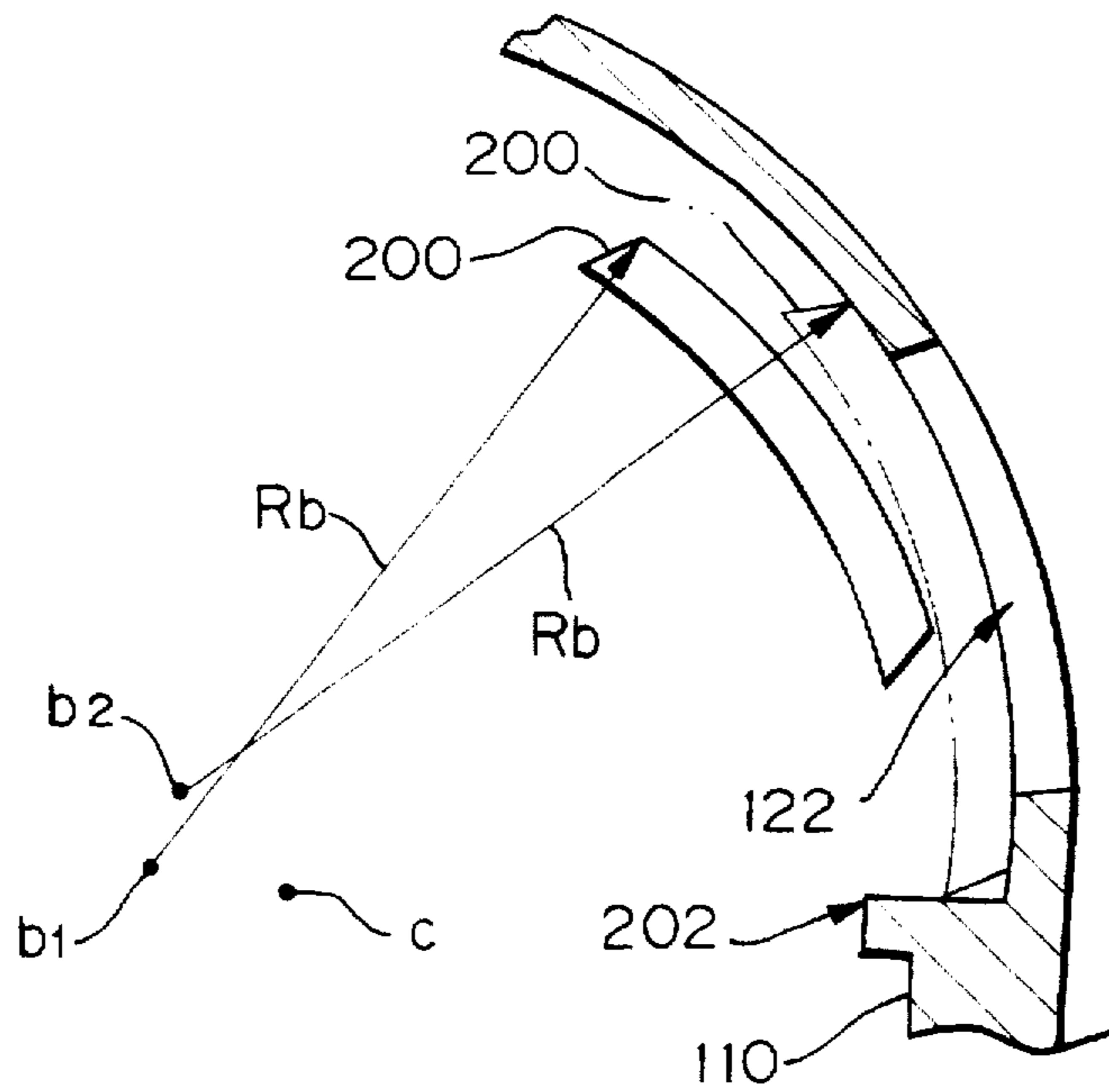
Fig. 14C
