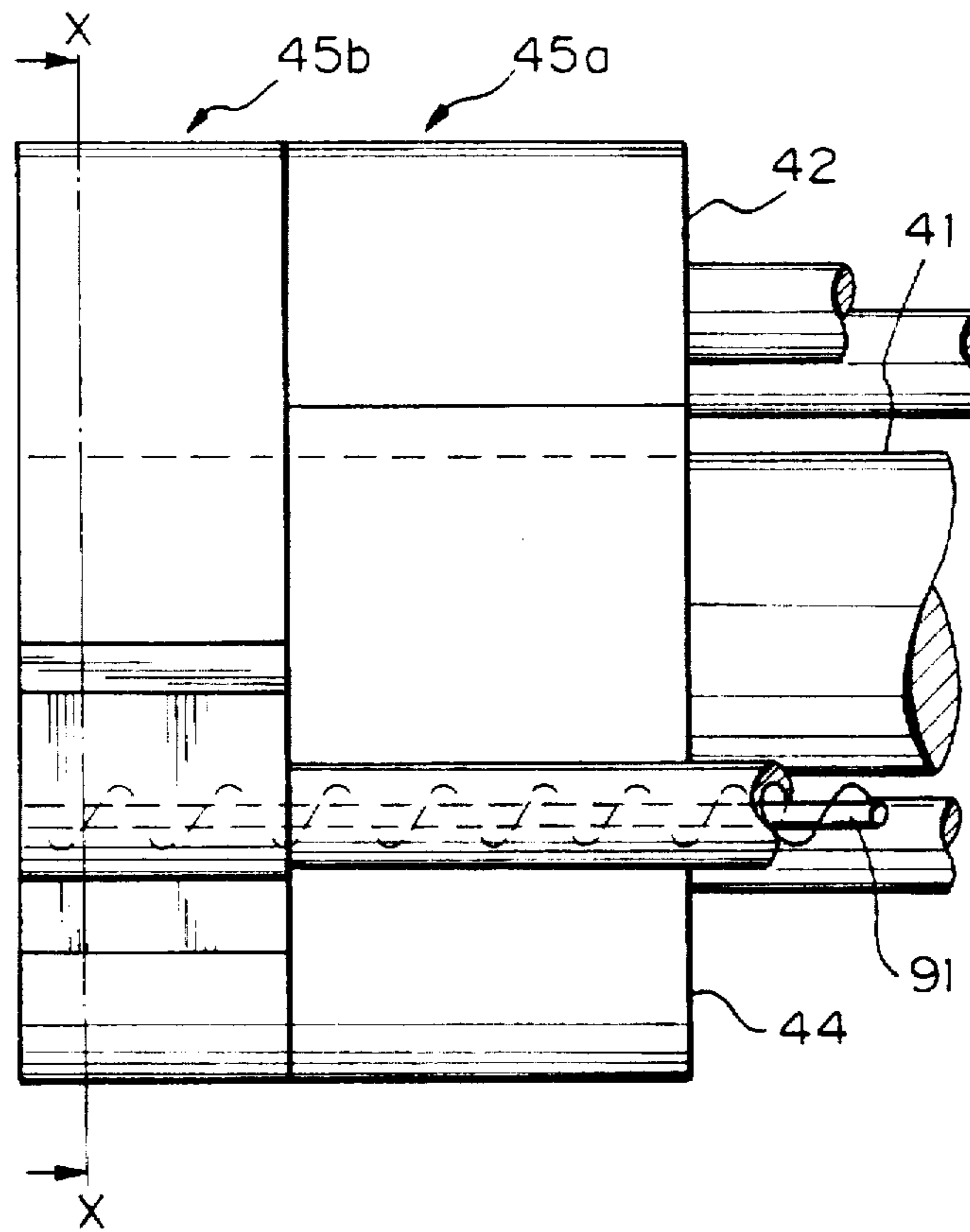
Fig. 12B
