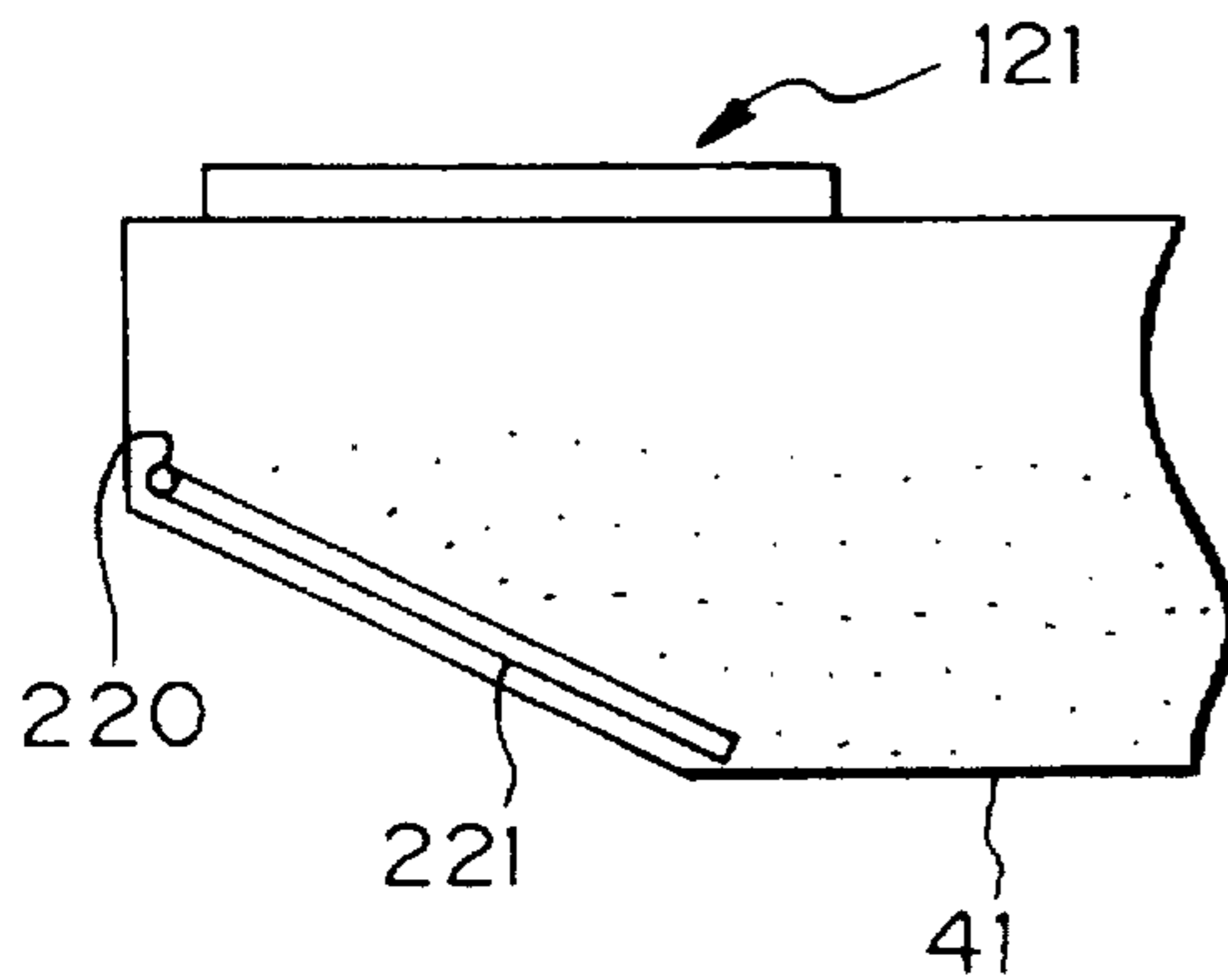
Fig. 17A
