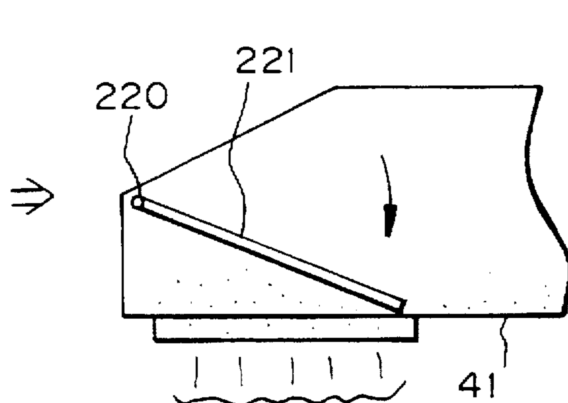
Fig. 17B
