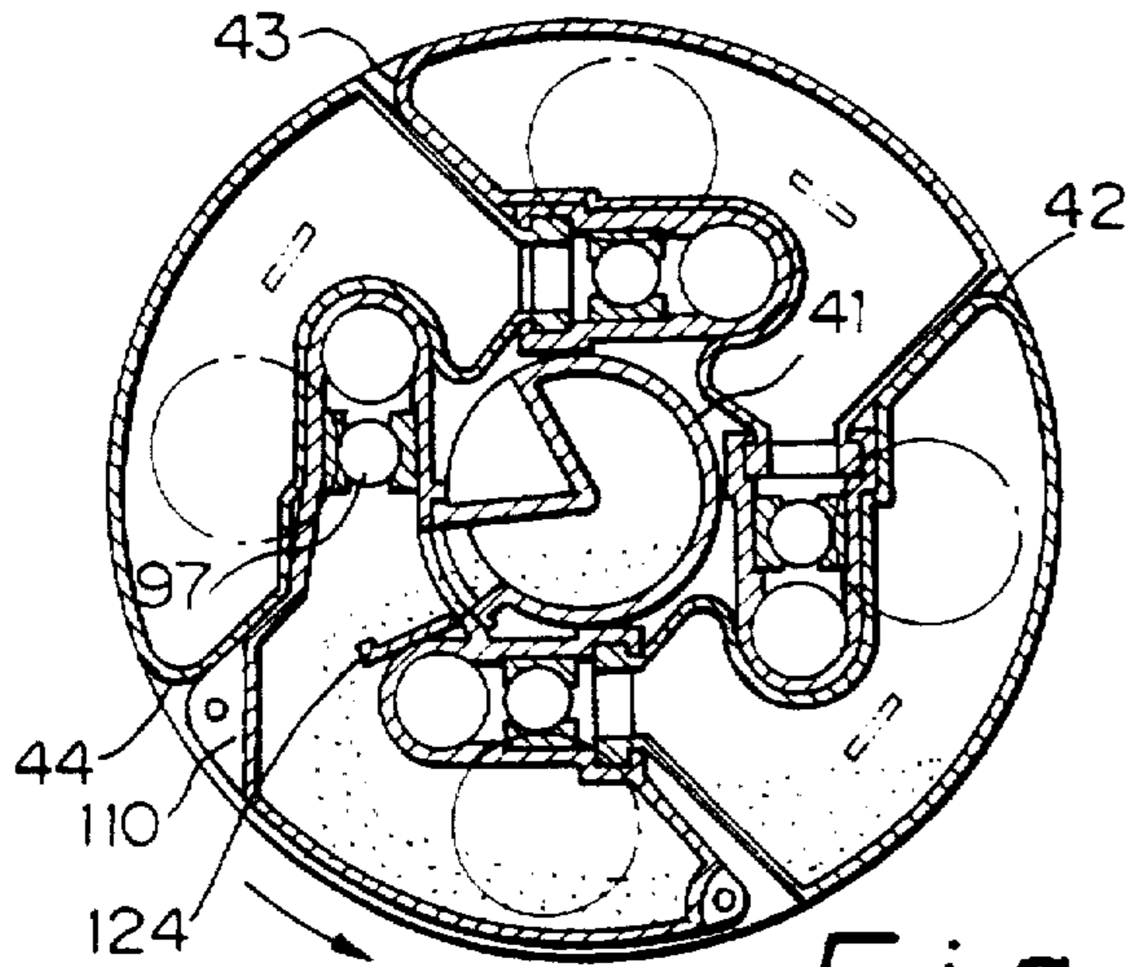
Fig. 15C
