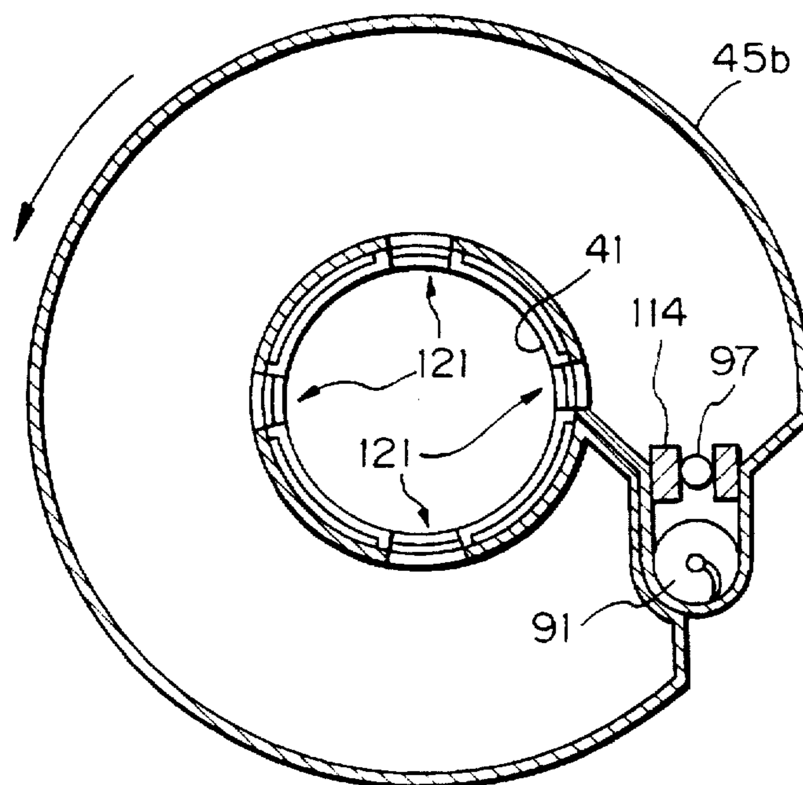
Fig. 12B
