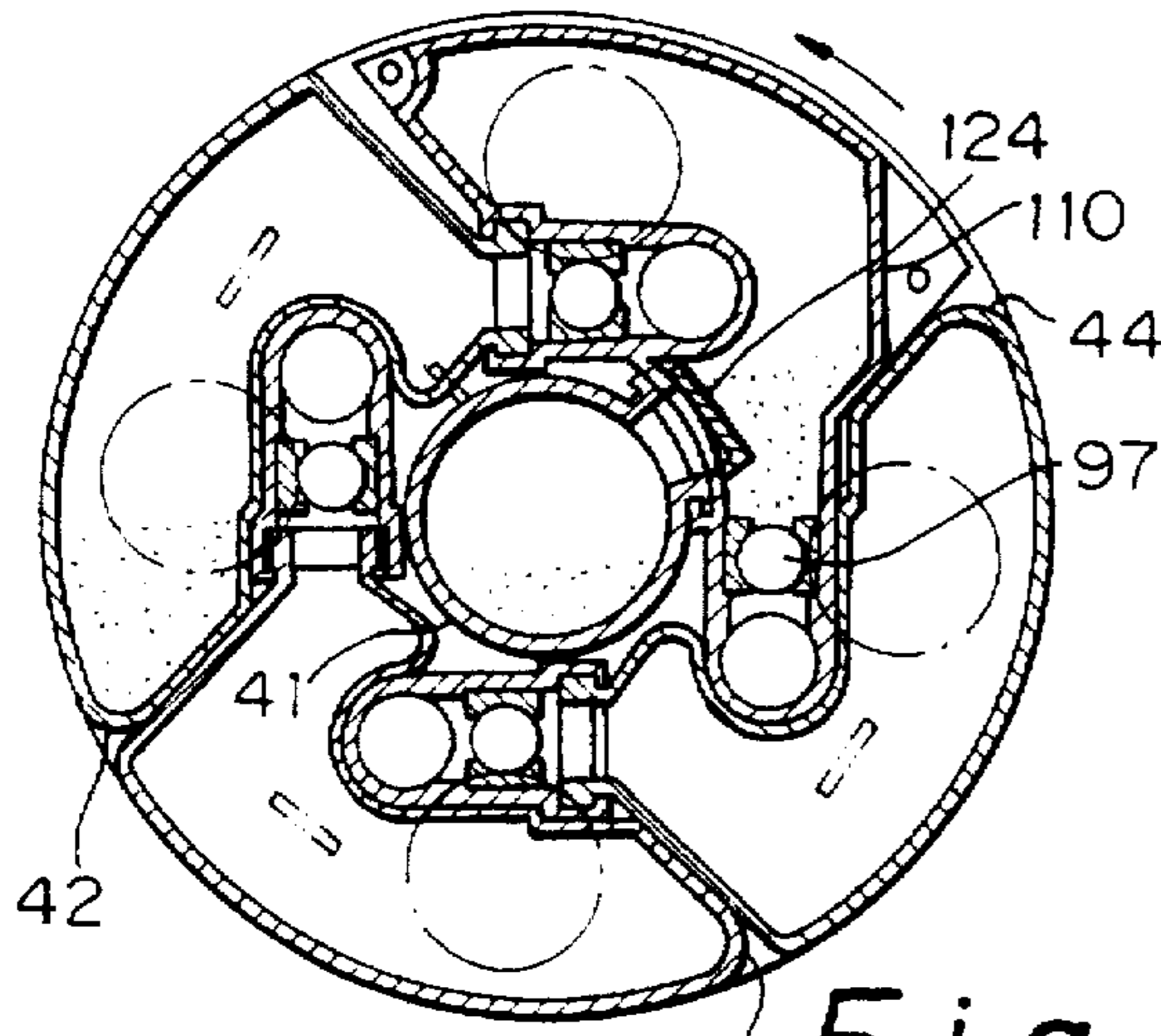
Fig. 10A
