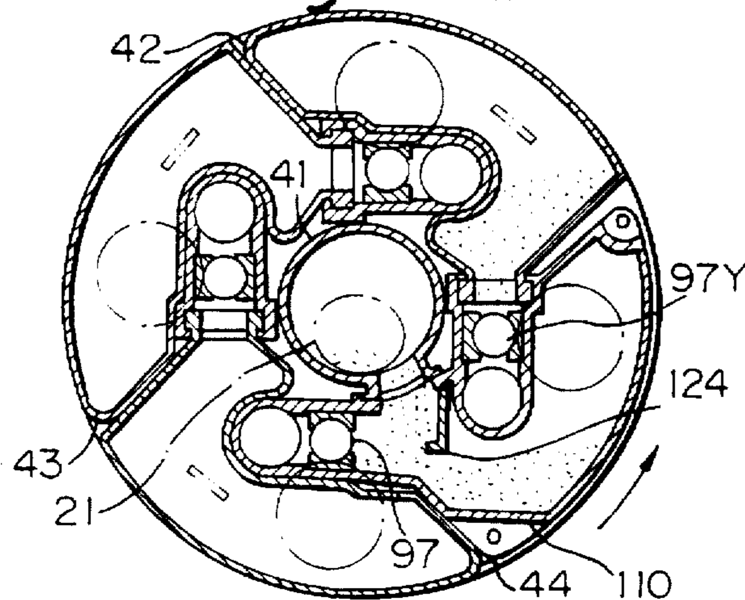
Fig. 15E
