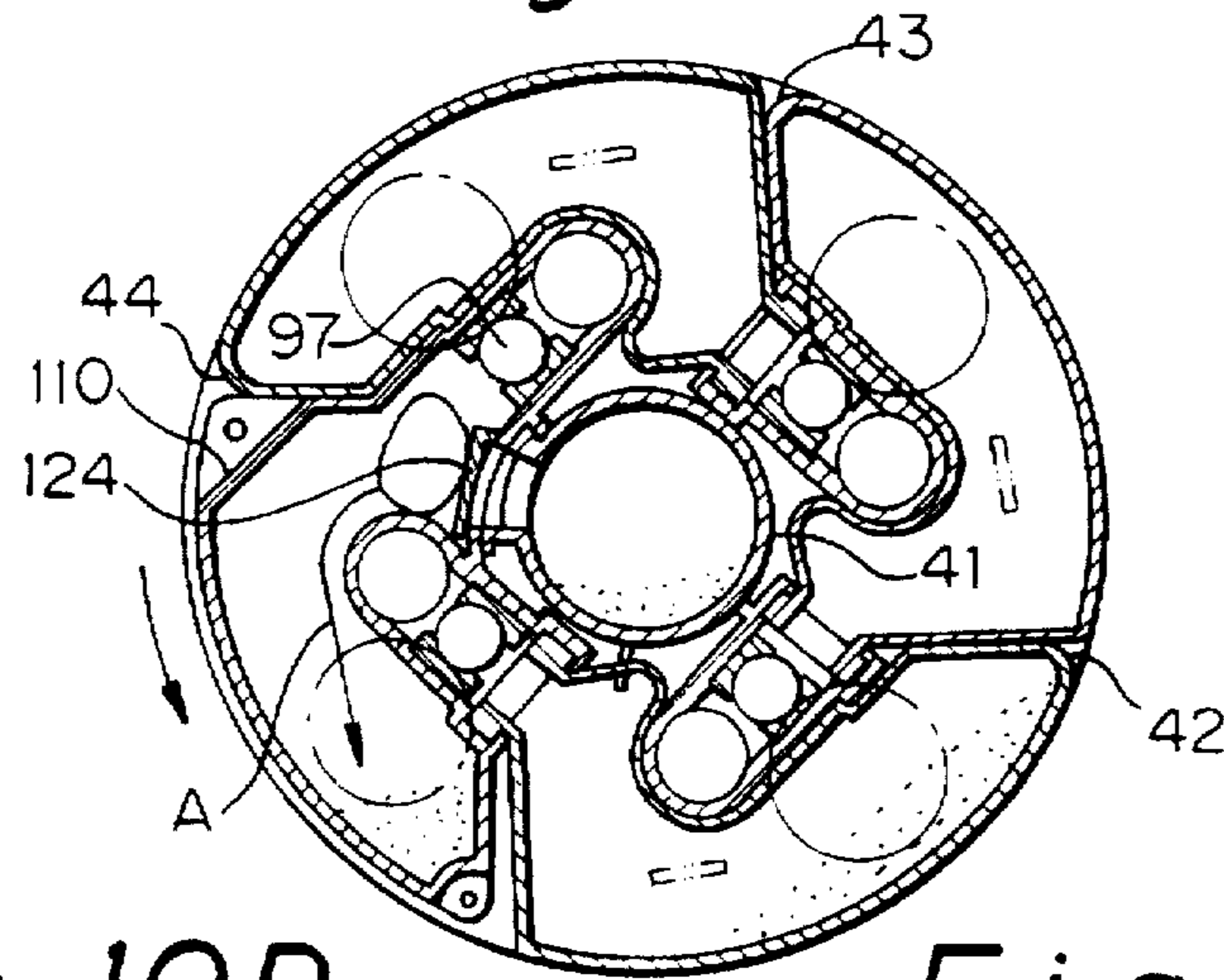
Fig. 10C
