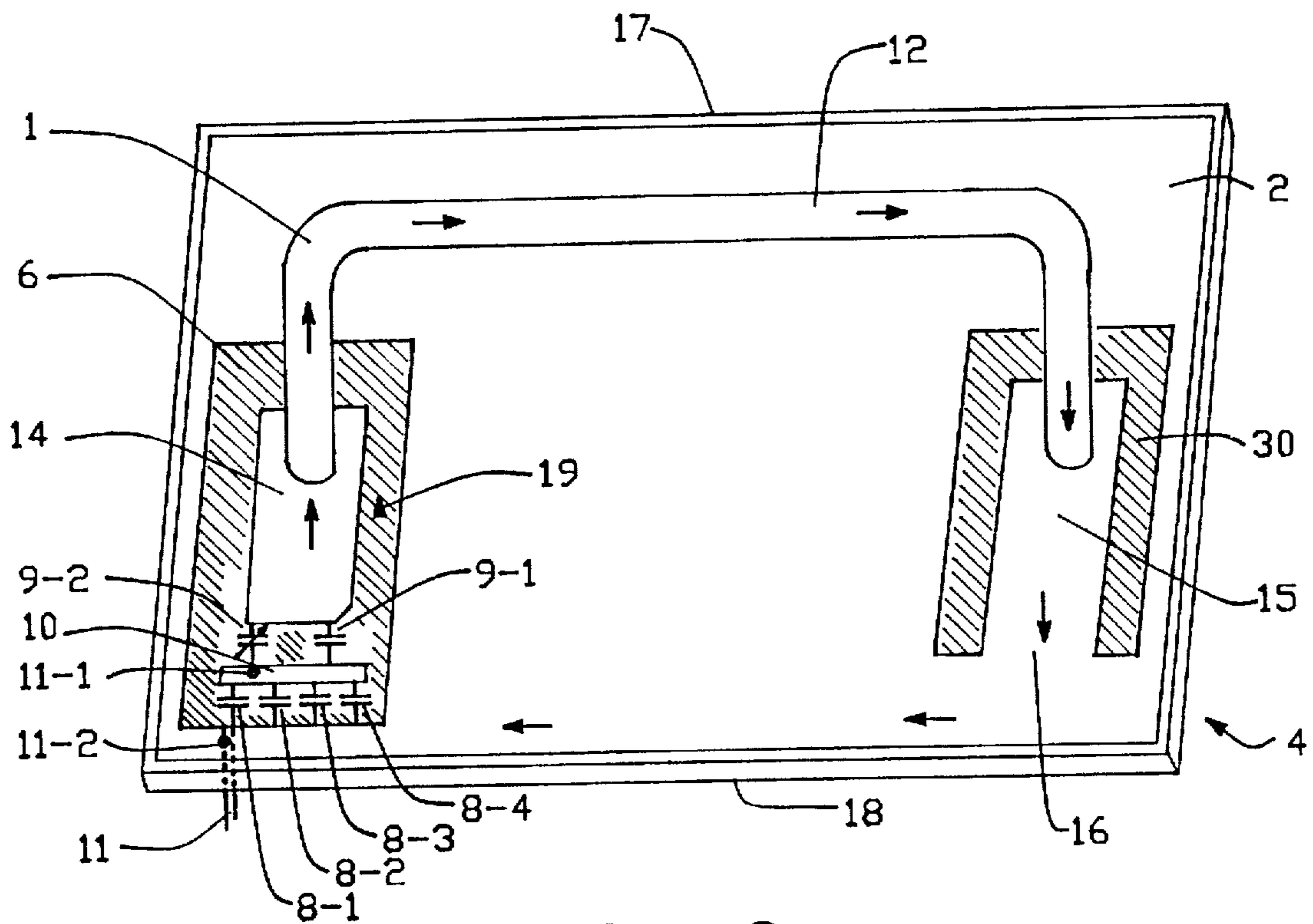
FIG. - 6a
