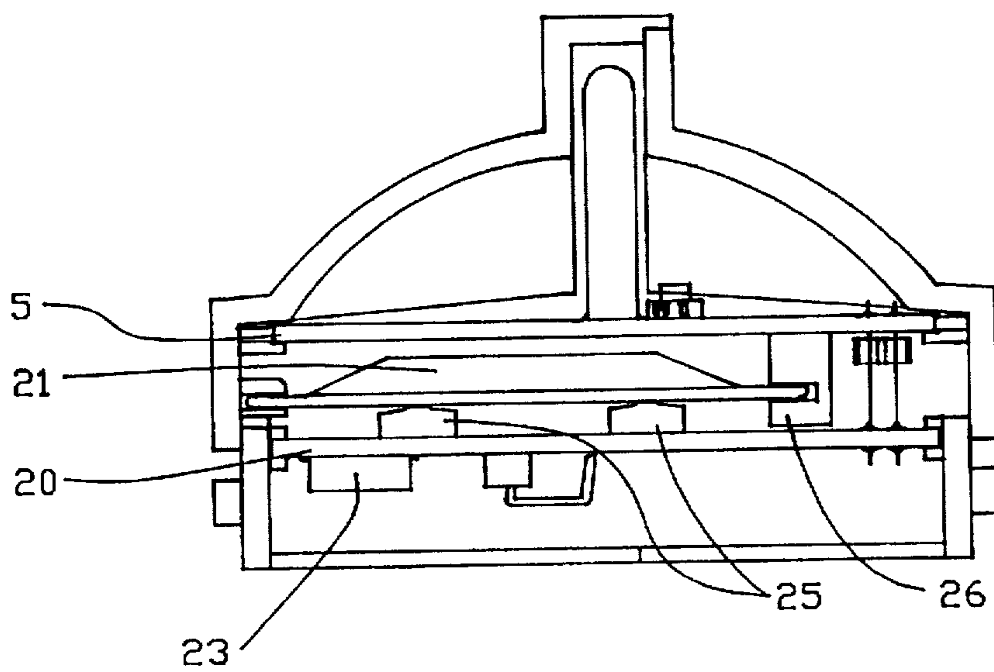
FIG. - 3b
