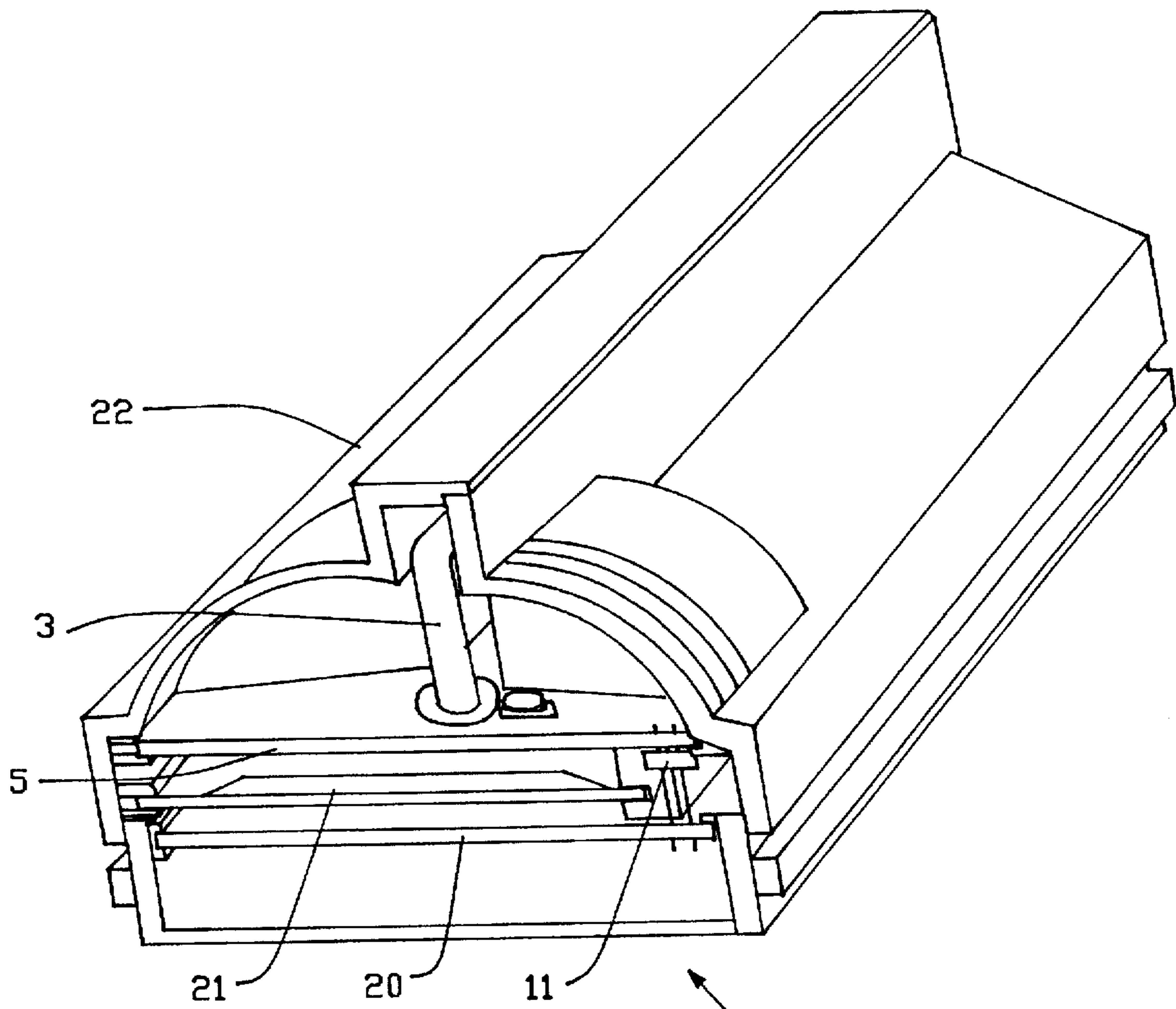
FIG. - 3a
