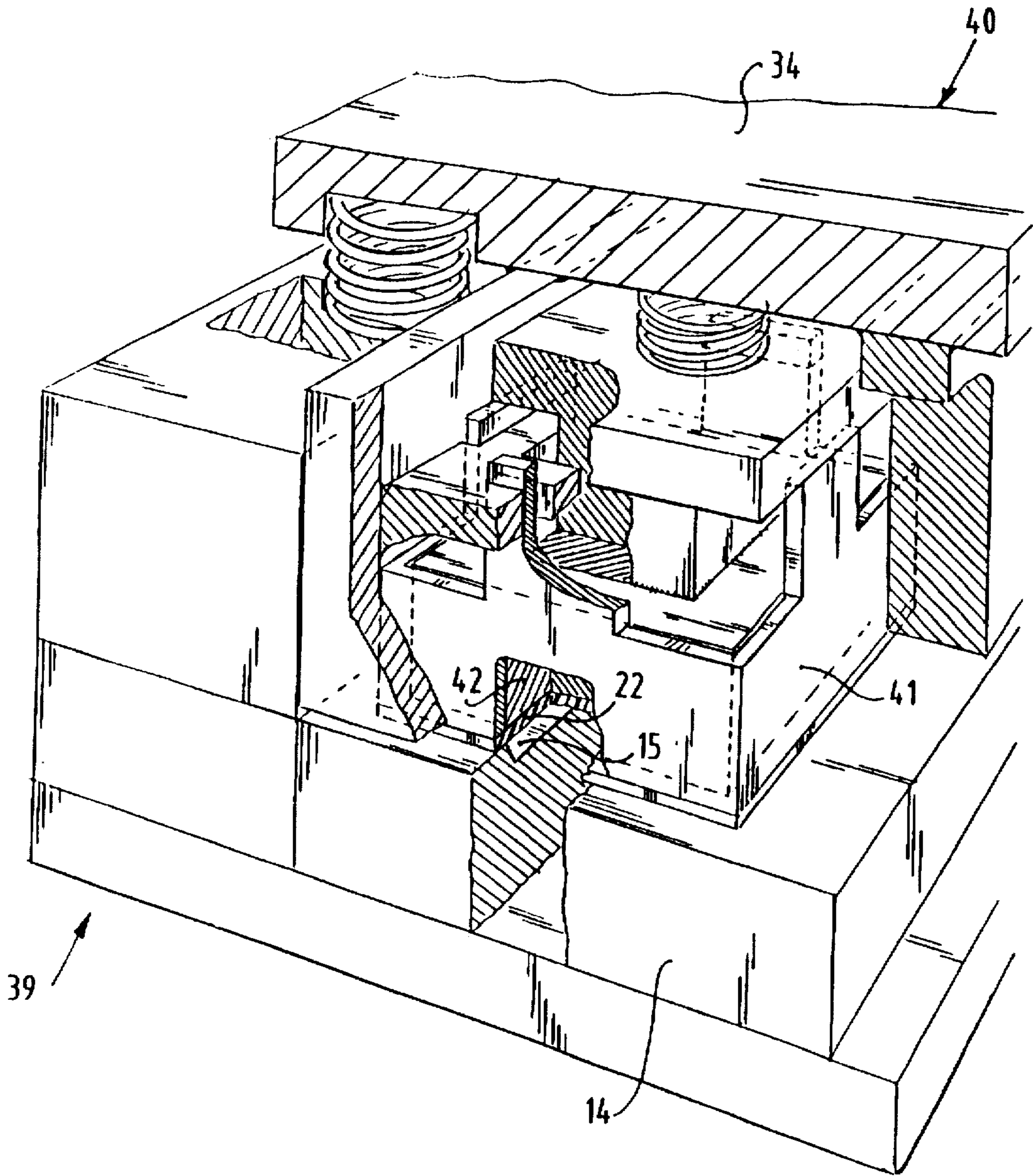
FIG. 7
