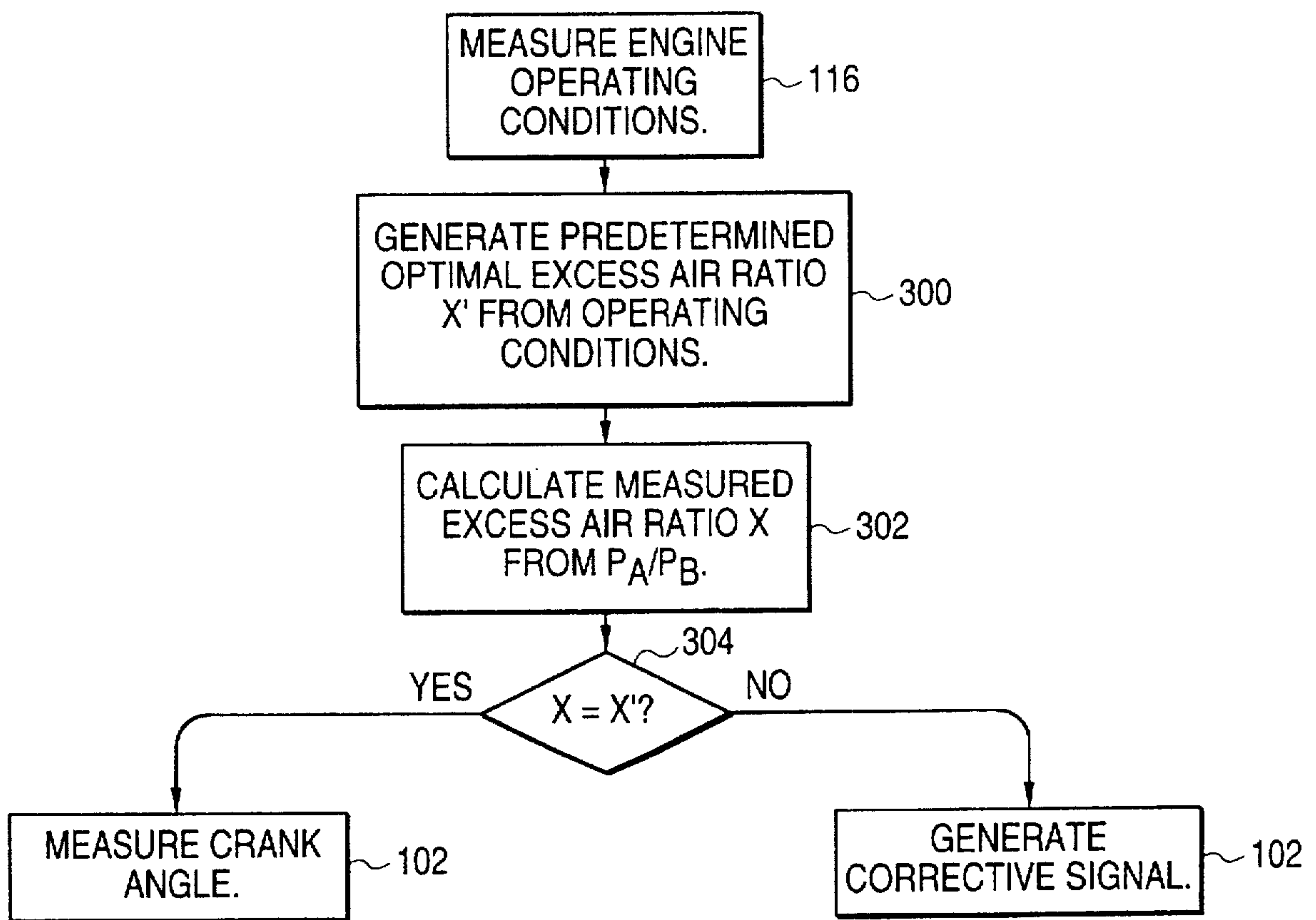
FIG. 7
