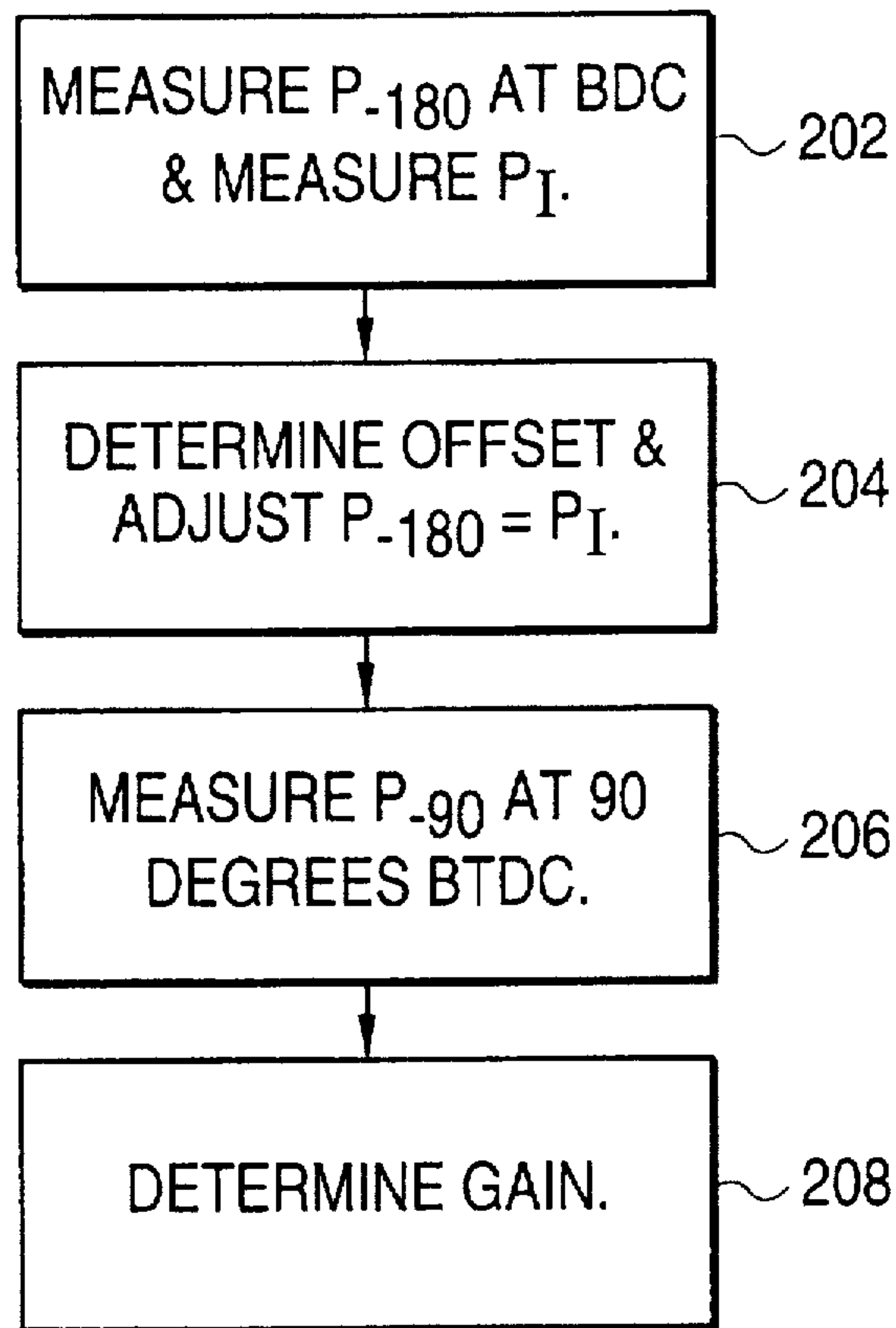
FIG. 4
