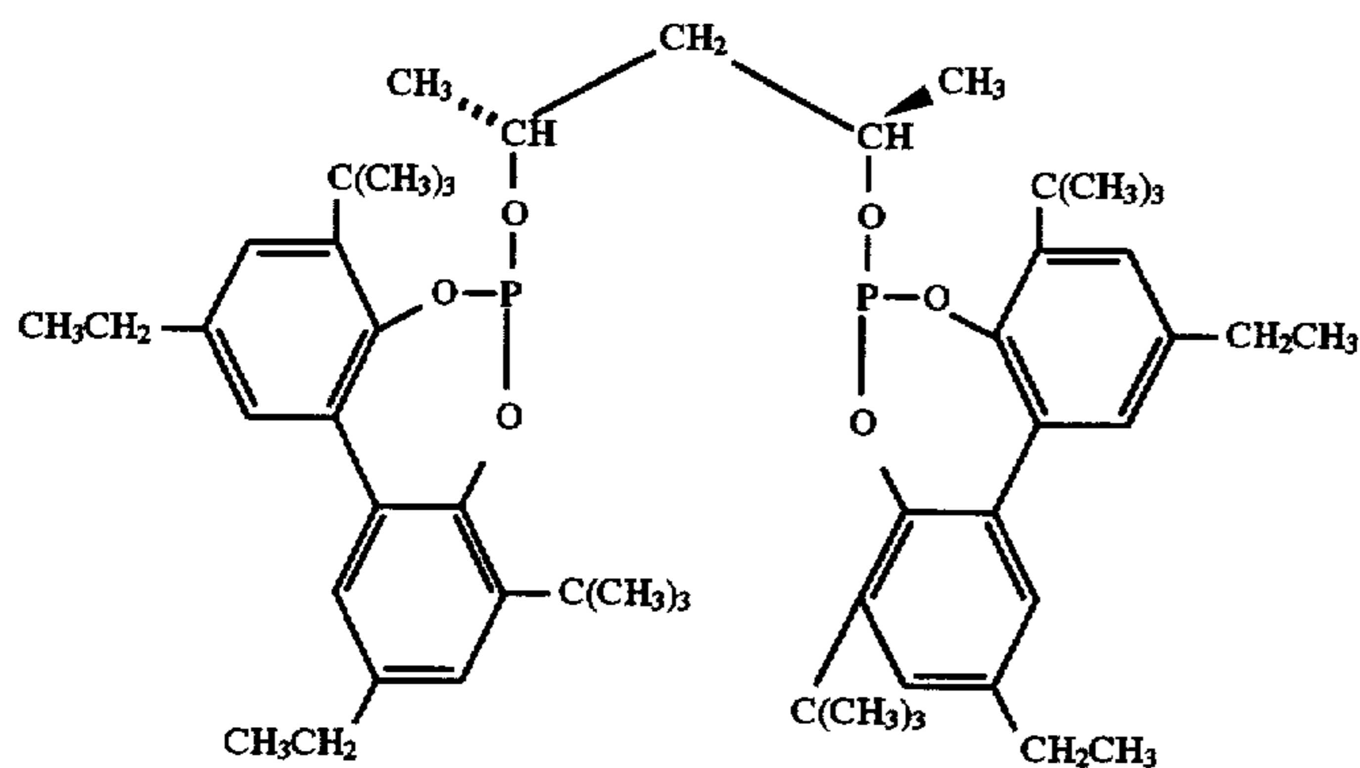
Ligand L
