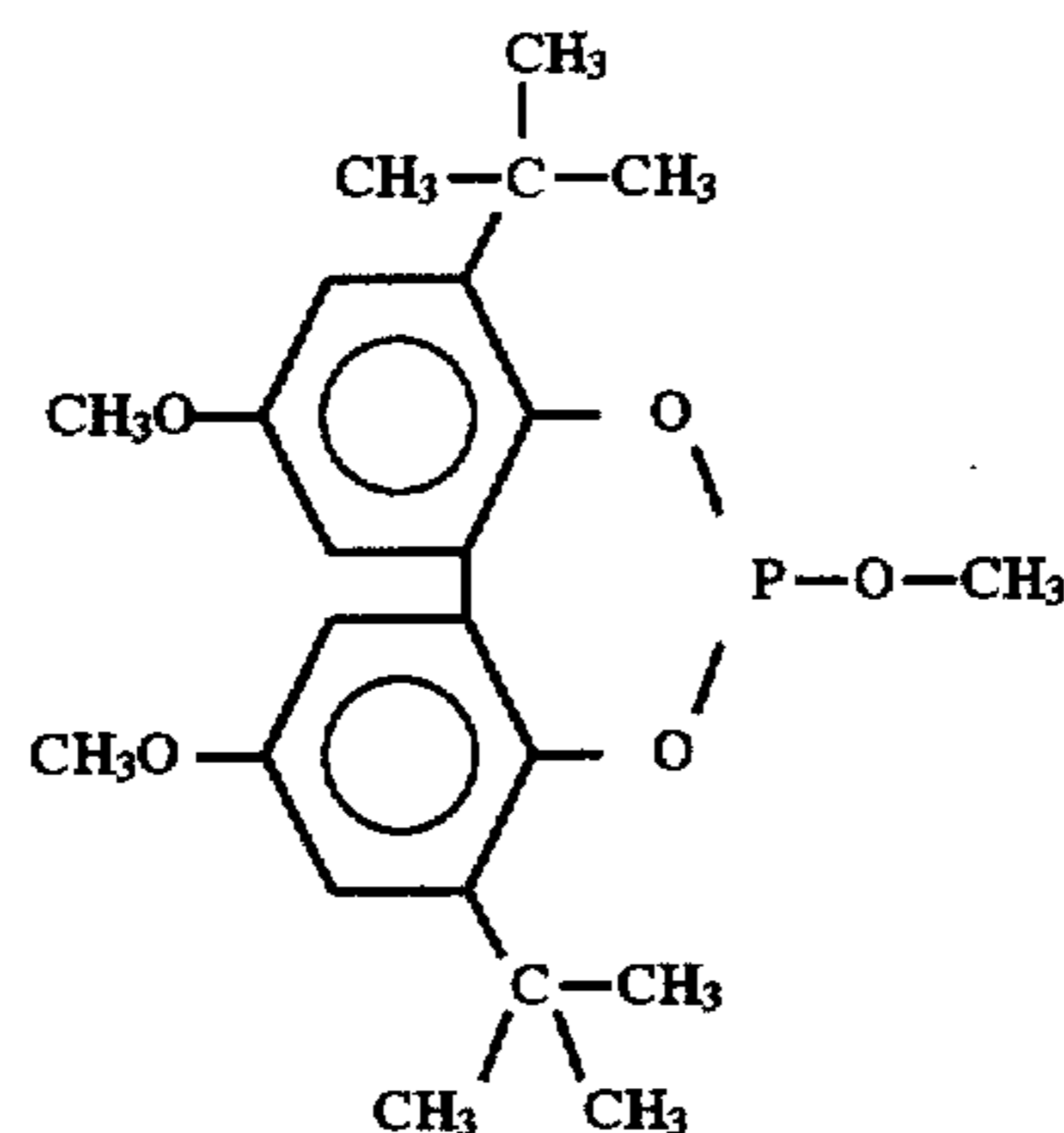
Ligand B
