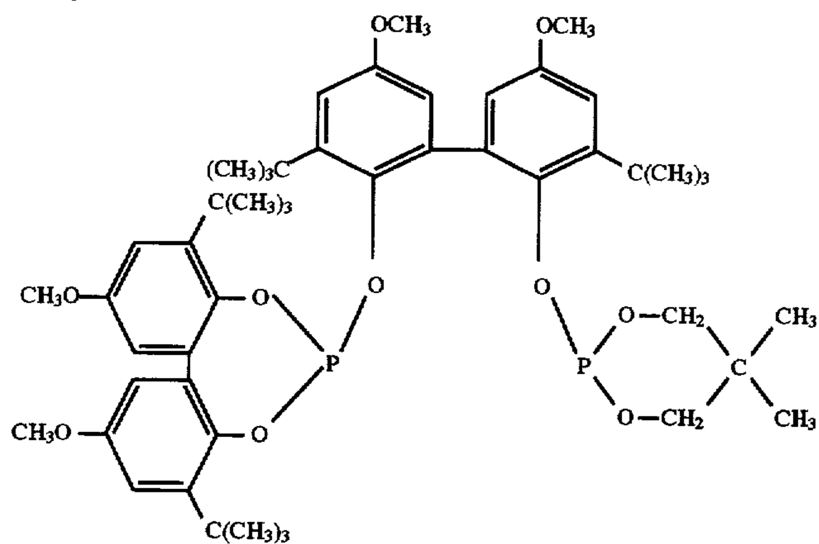
Ligand P
