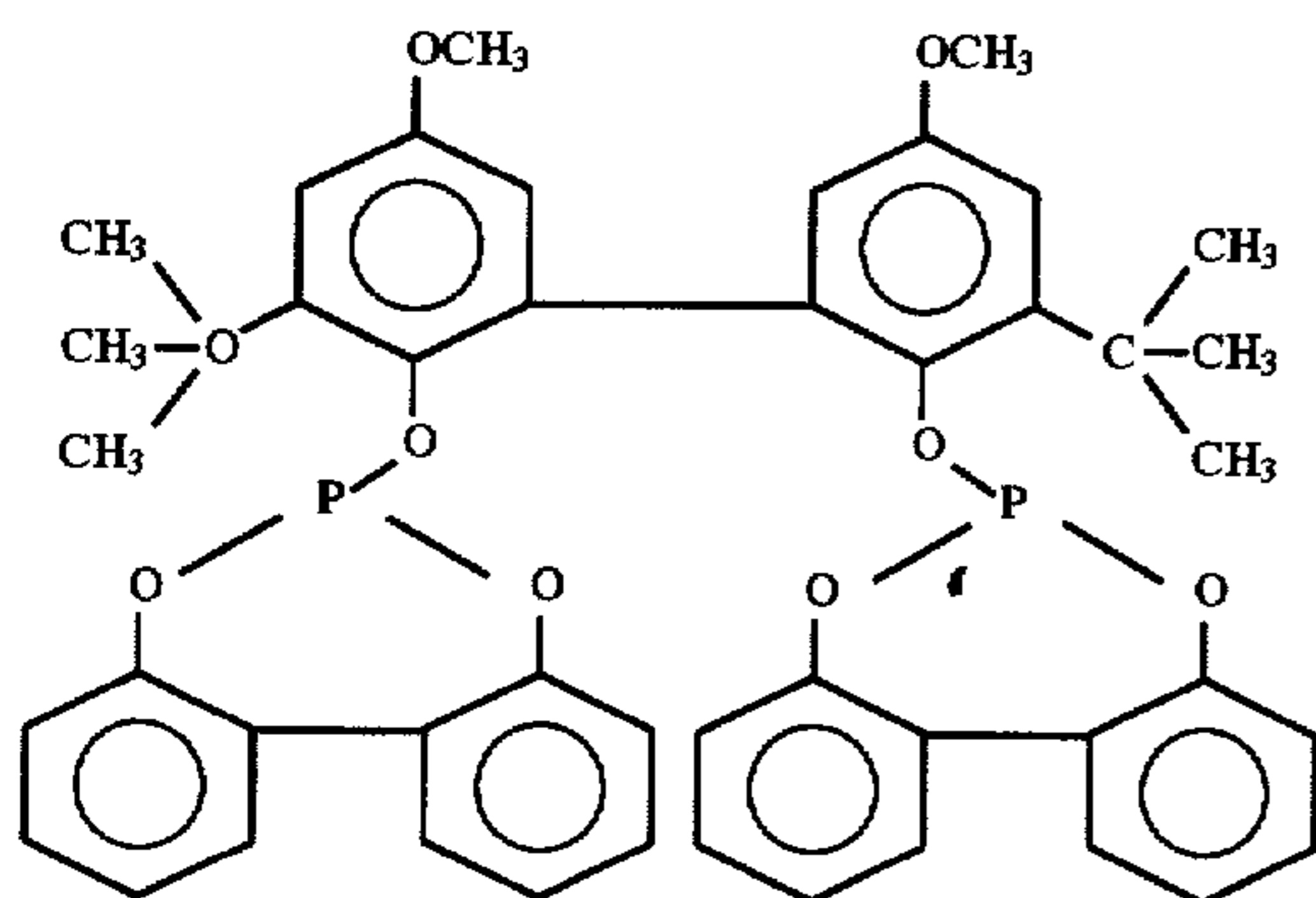
Ligand D
