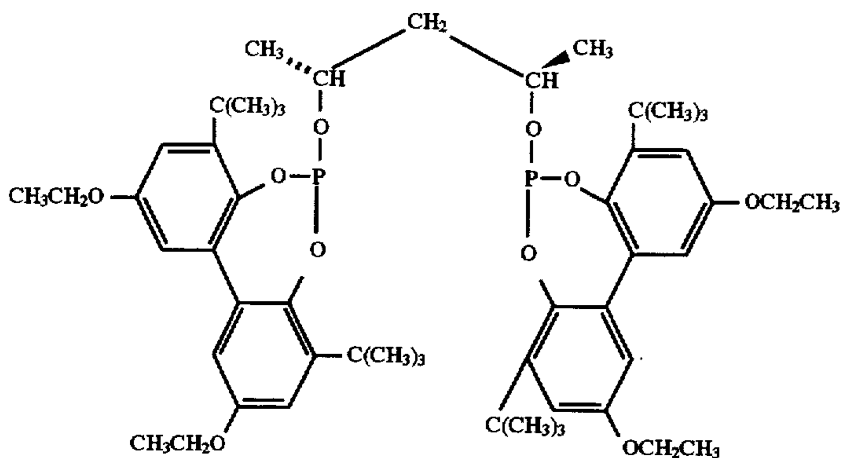
Ligand K
