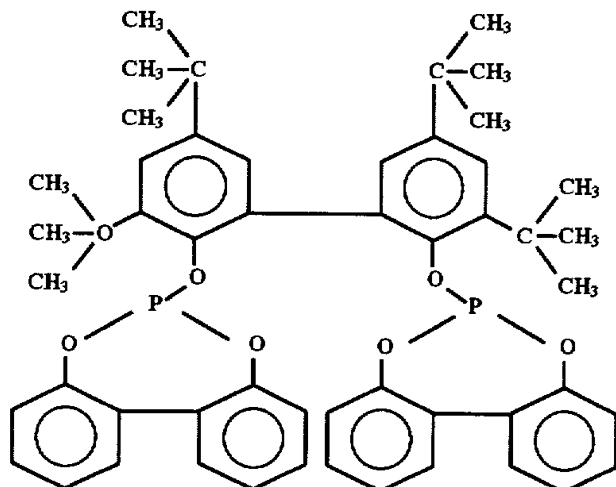
Ligand F
