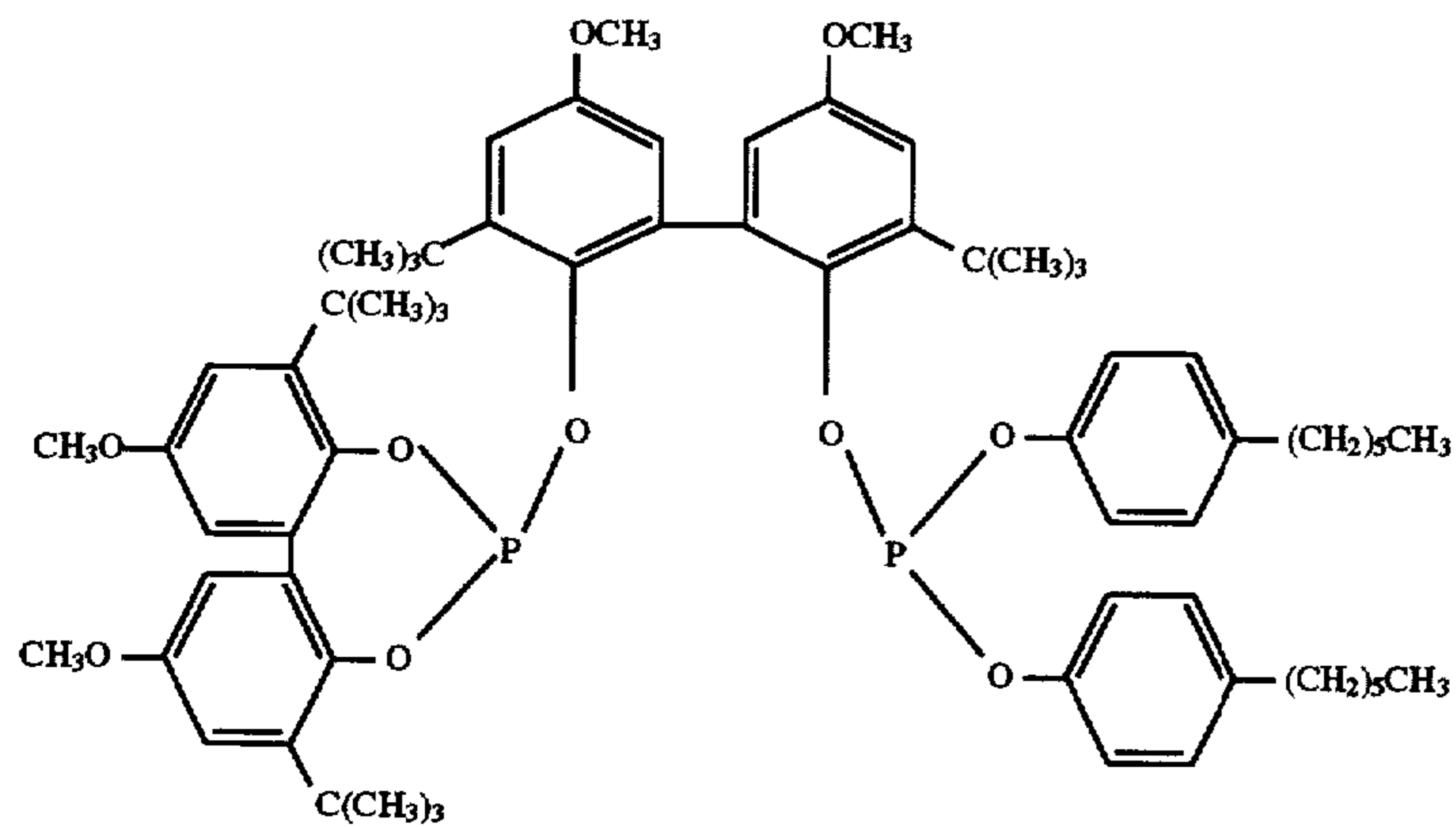
Ligand Q
