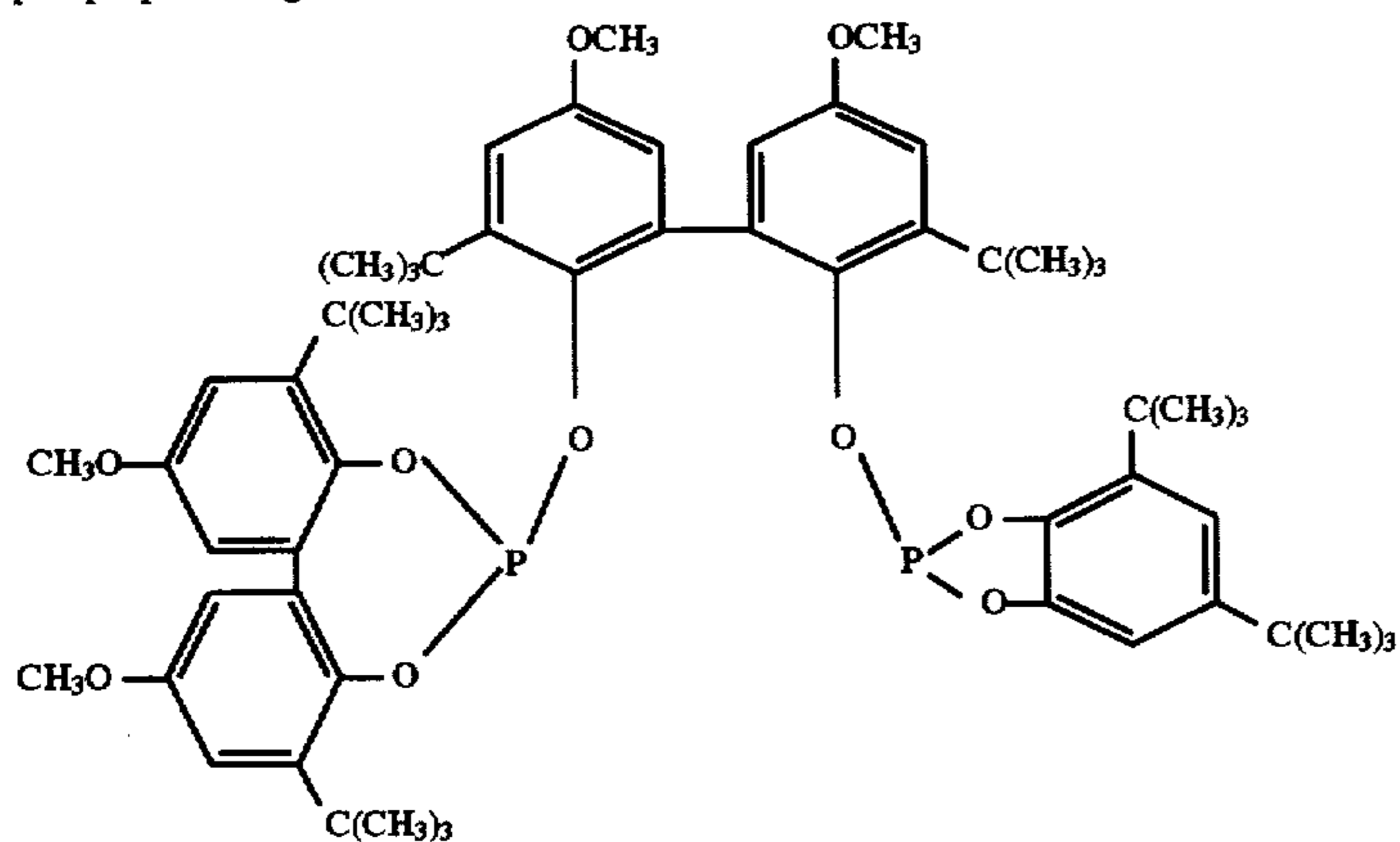
Ligand N
