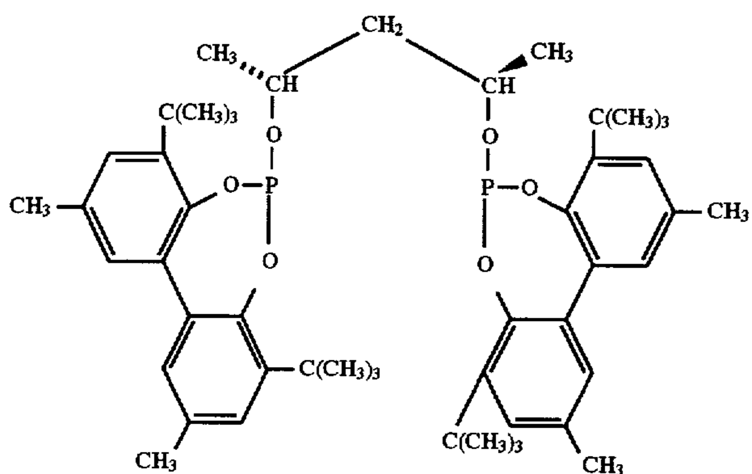
Ligand J
