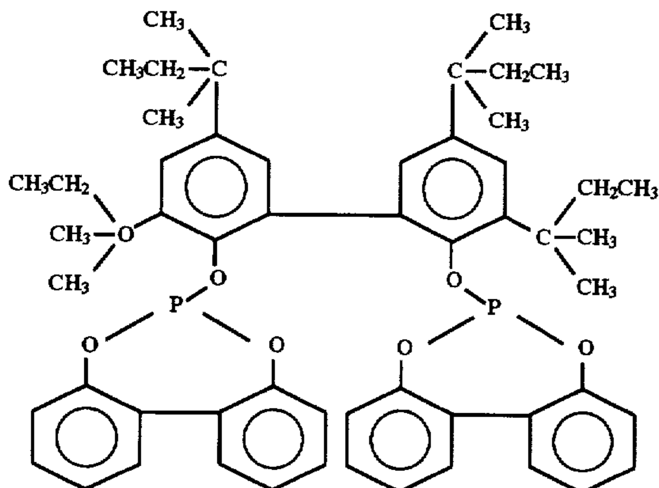
Ligand E
