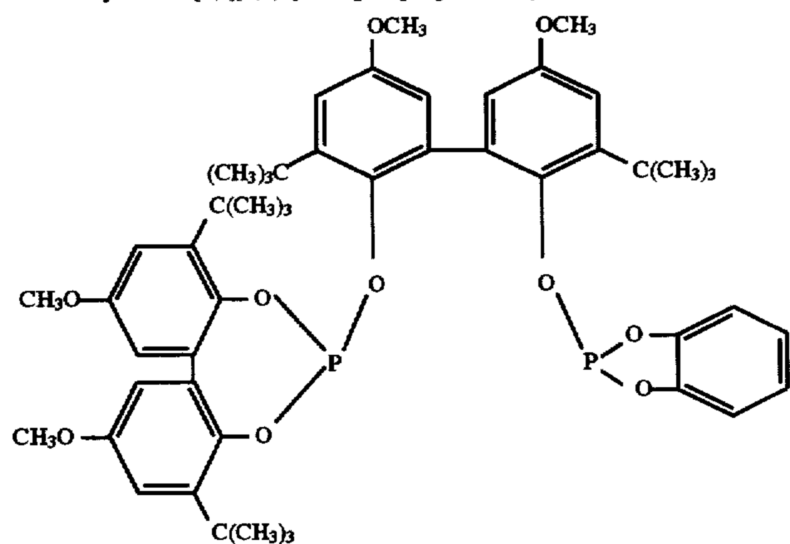
Ligand O
