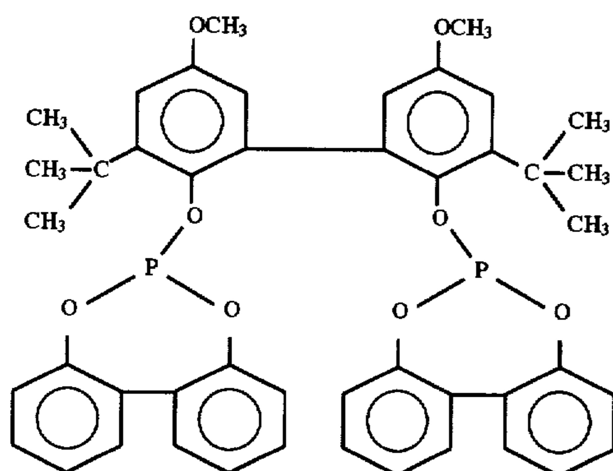
Ligand D
