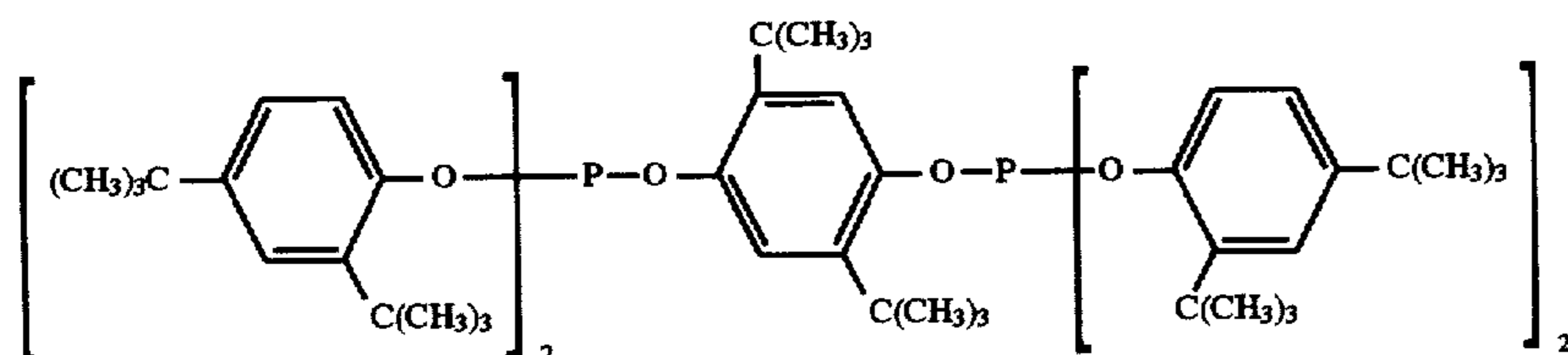
Ligand T
