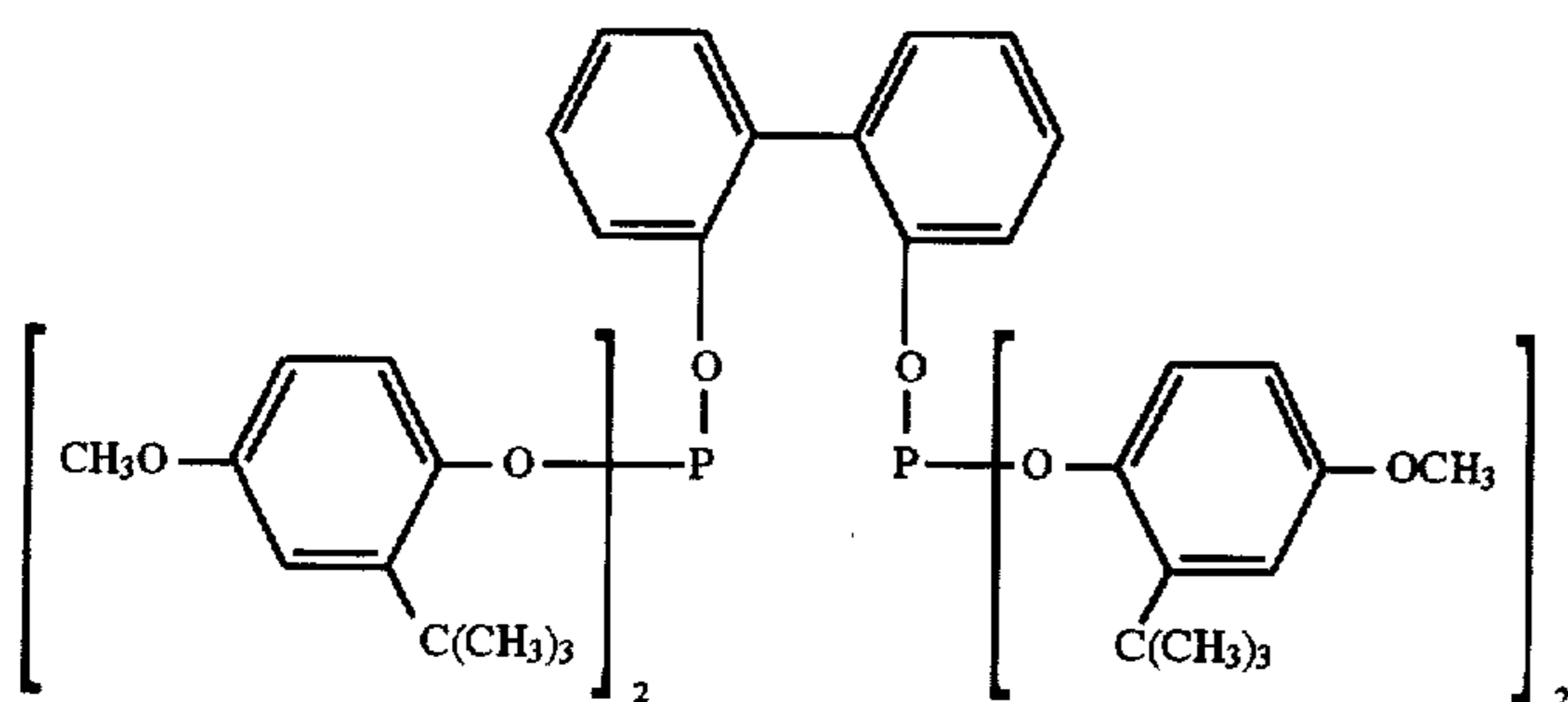
Ligand V
