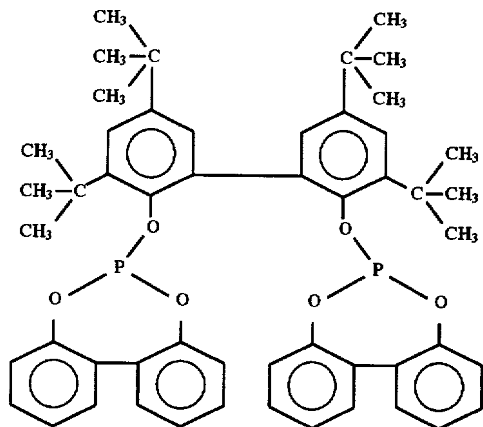
Ligand F
