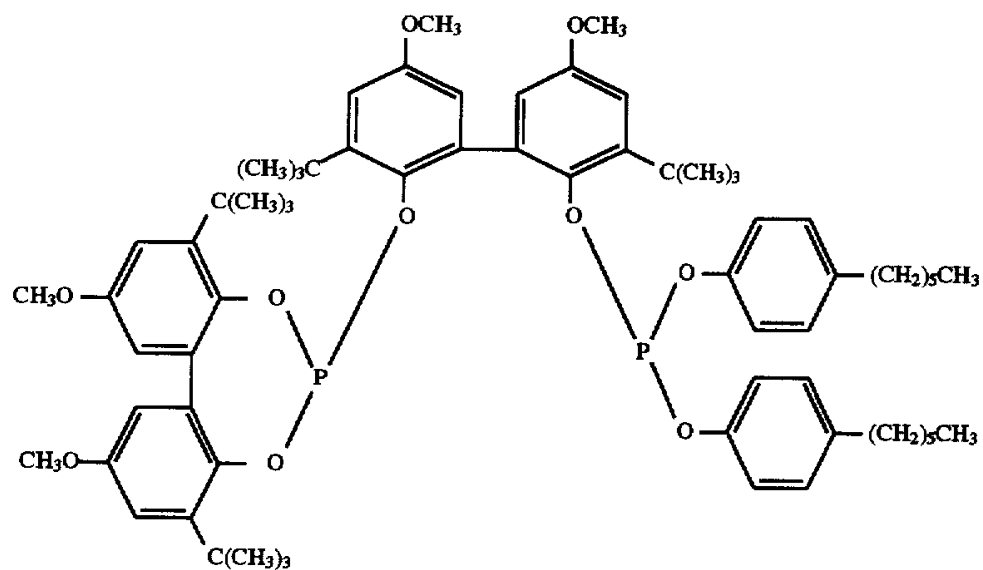
Ligand Q
