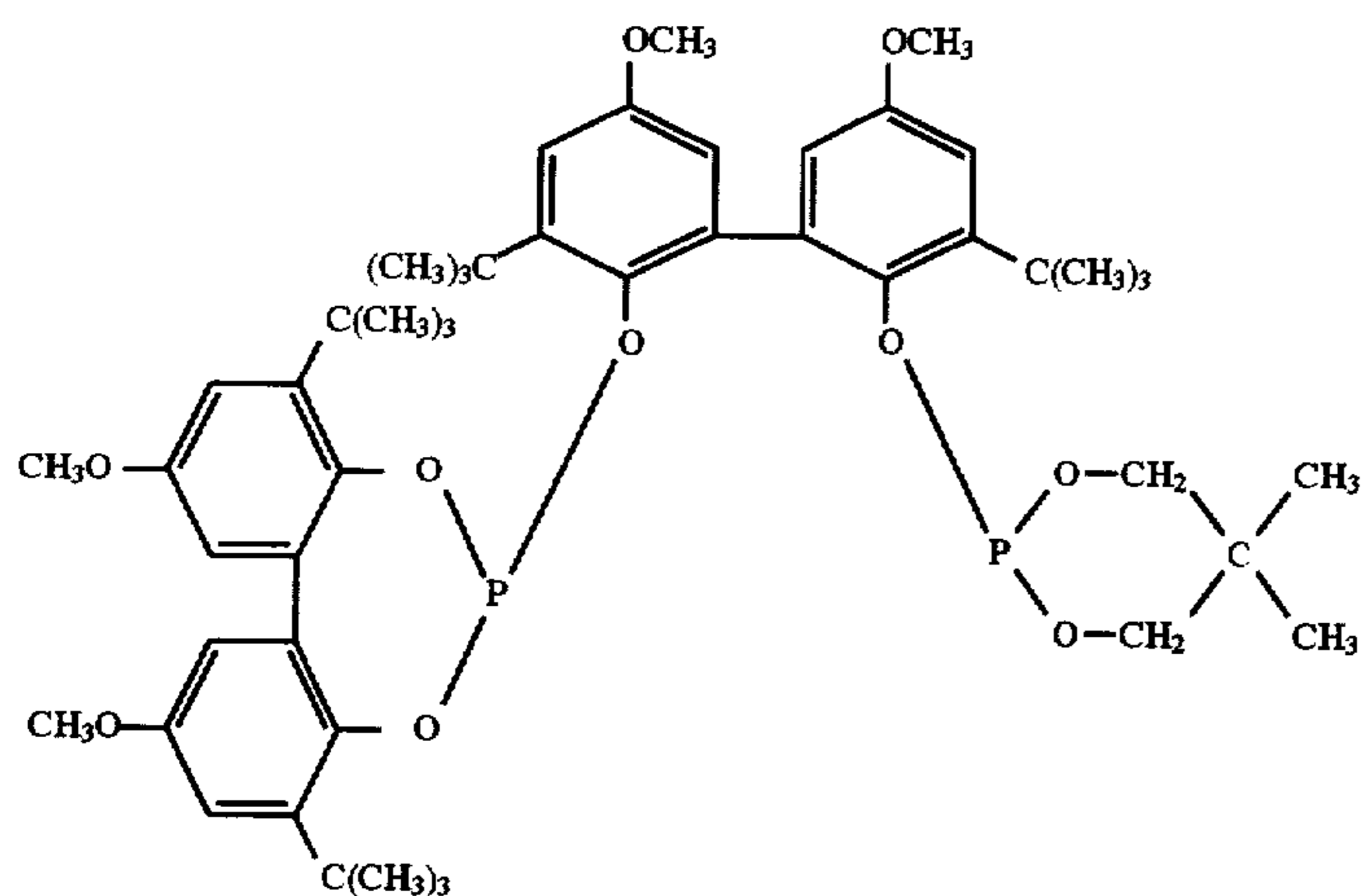
Ligand P
