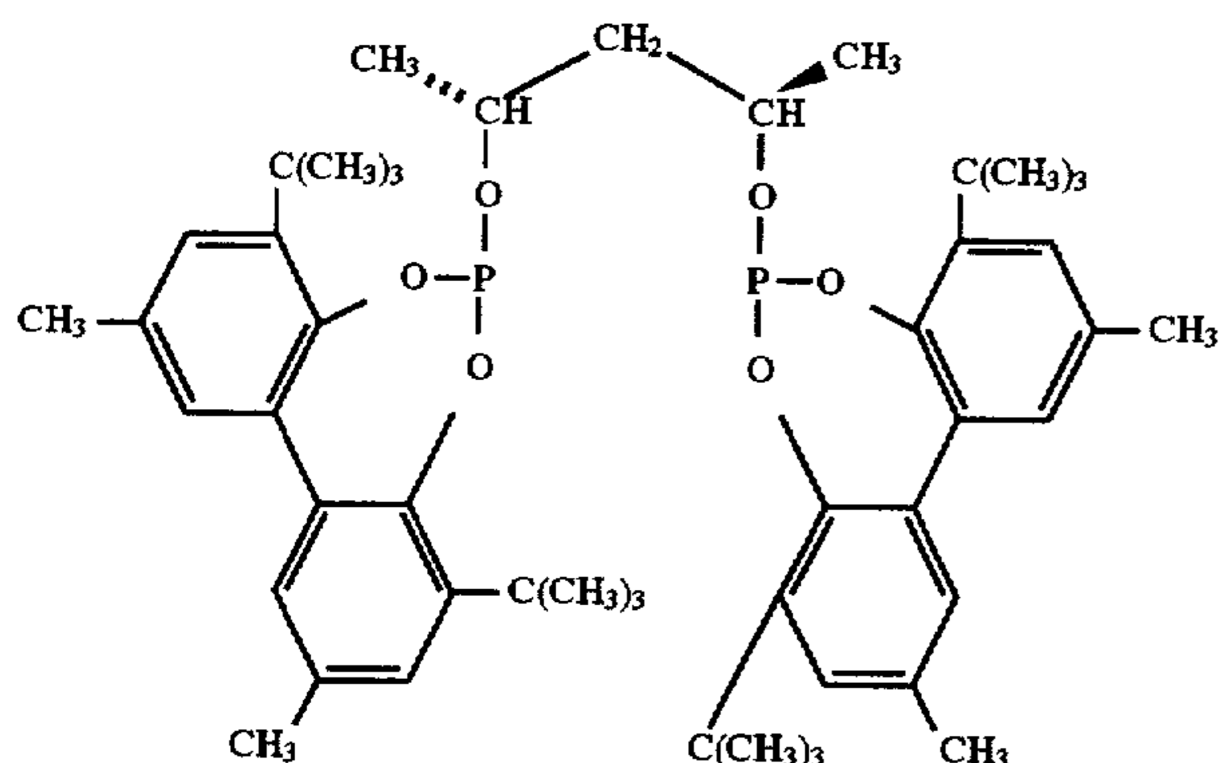
Ligand J
