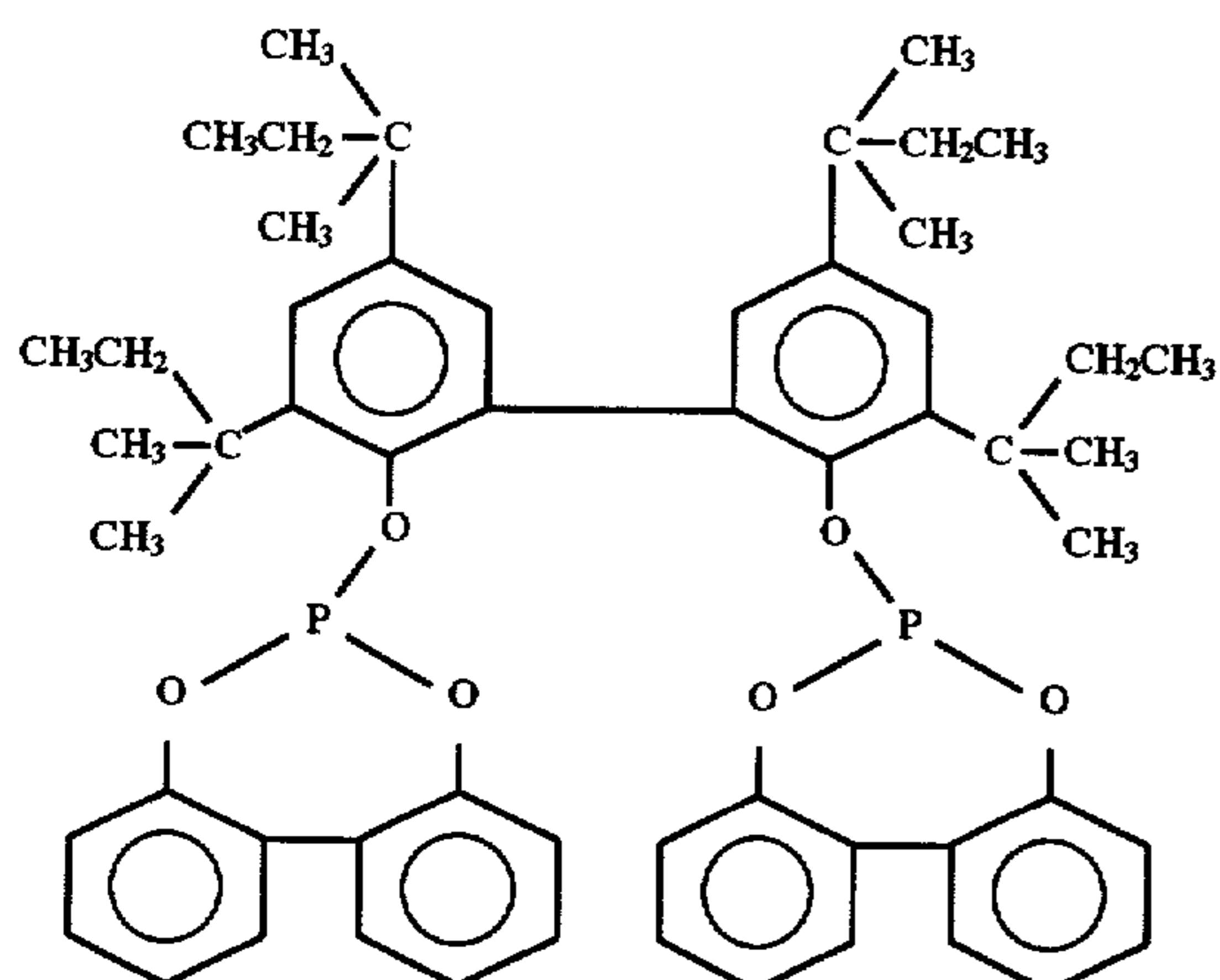
Ligand E
