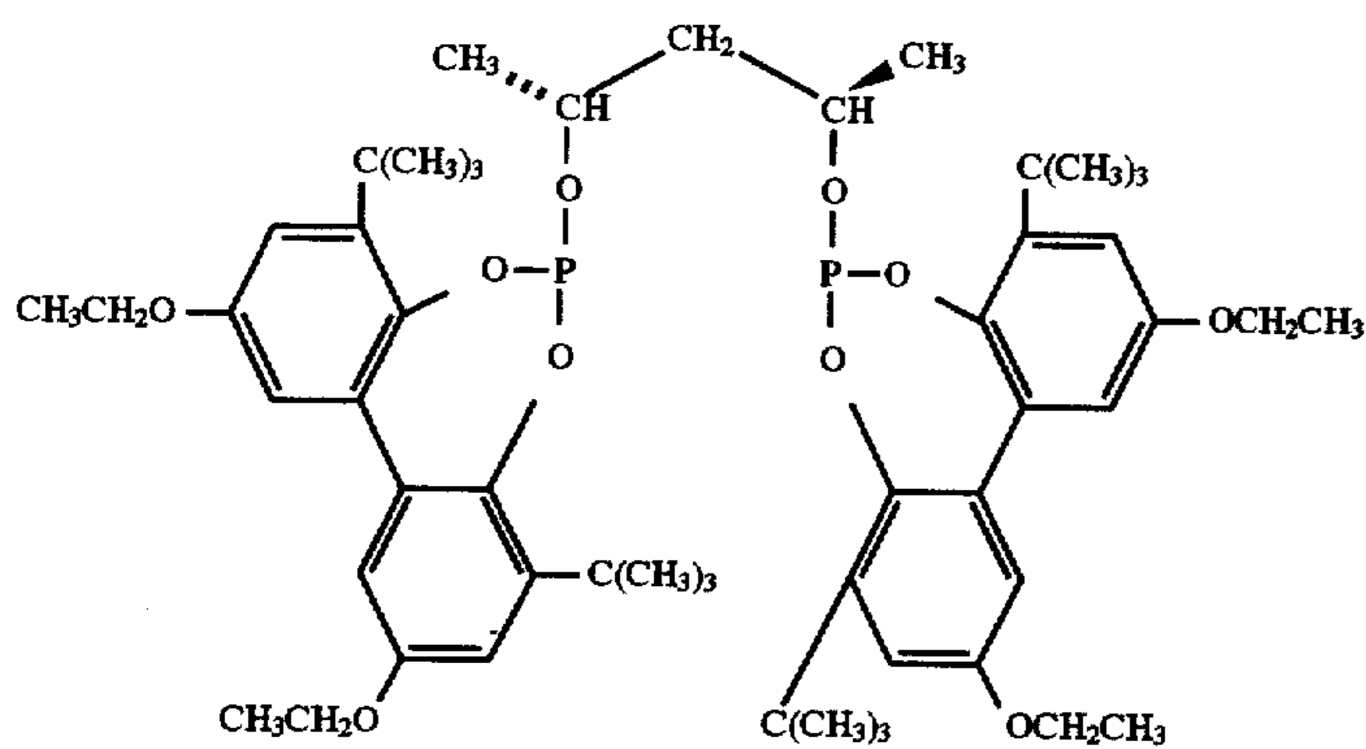
Ligand K
