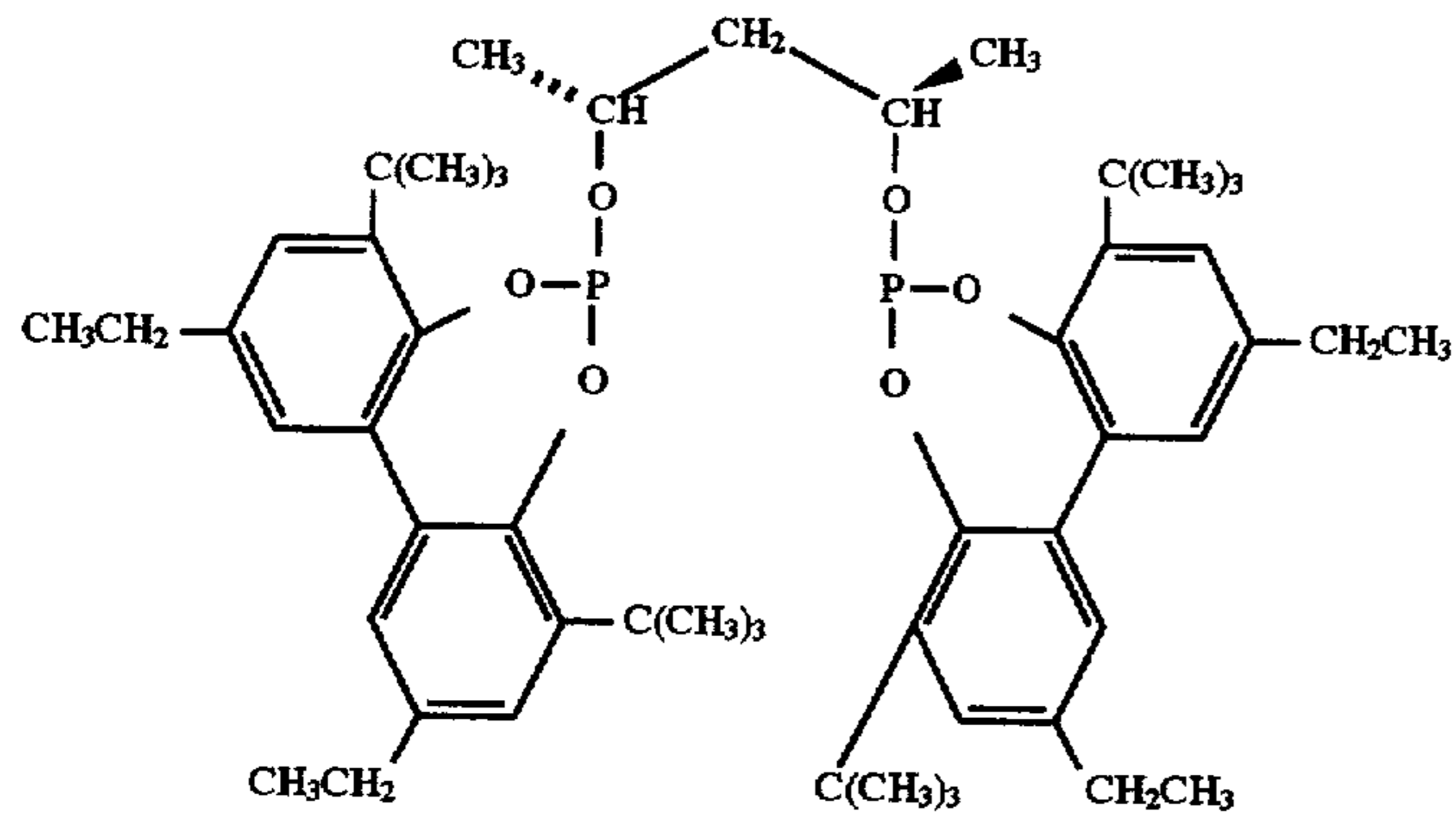
Ligand L
