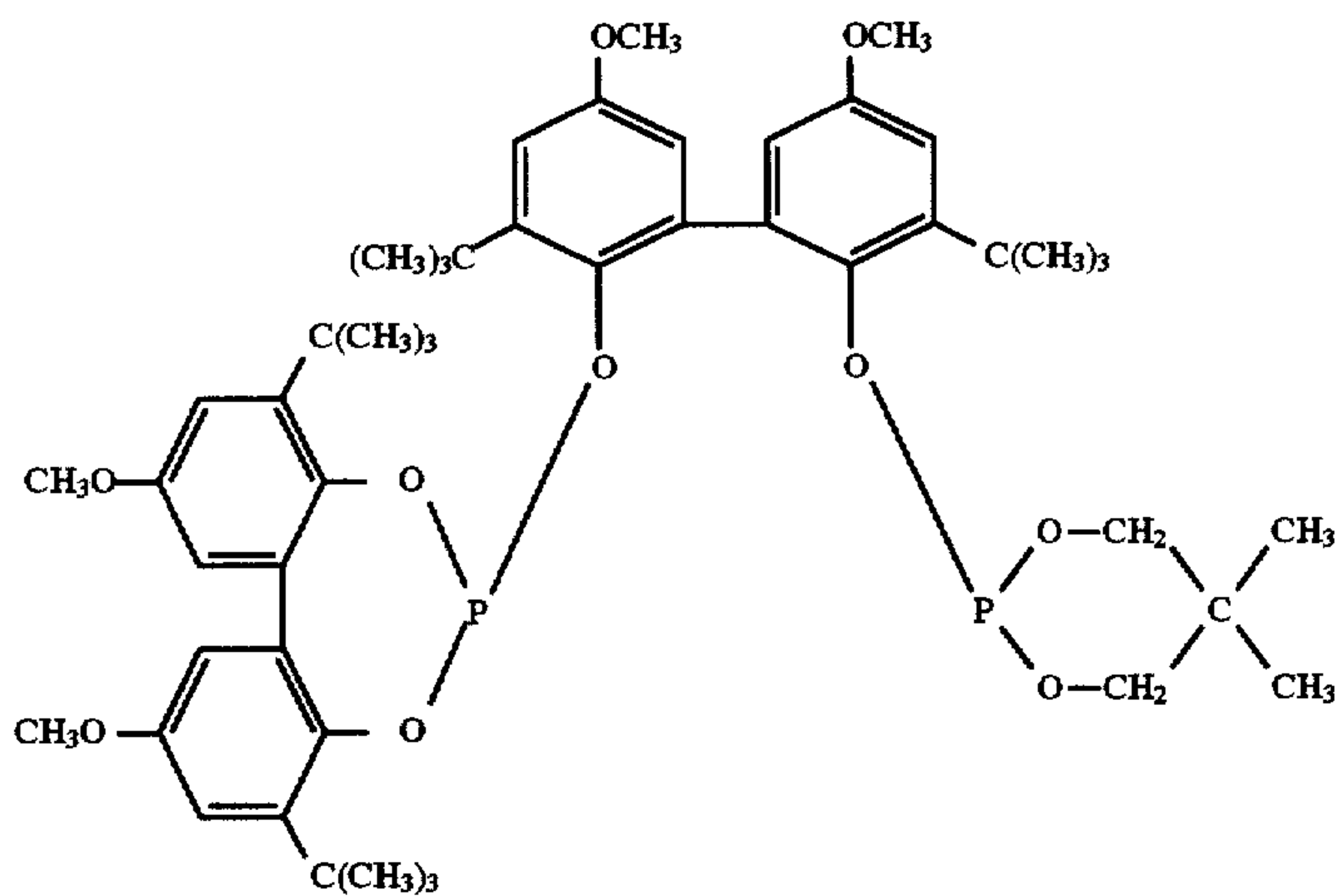
Ligand N
