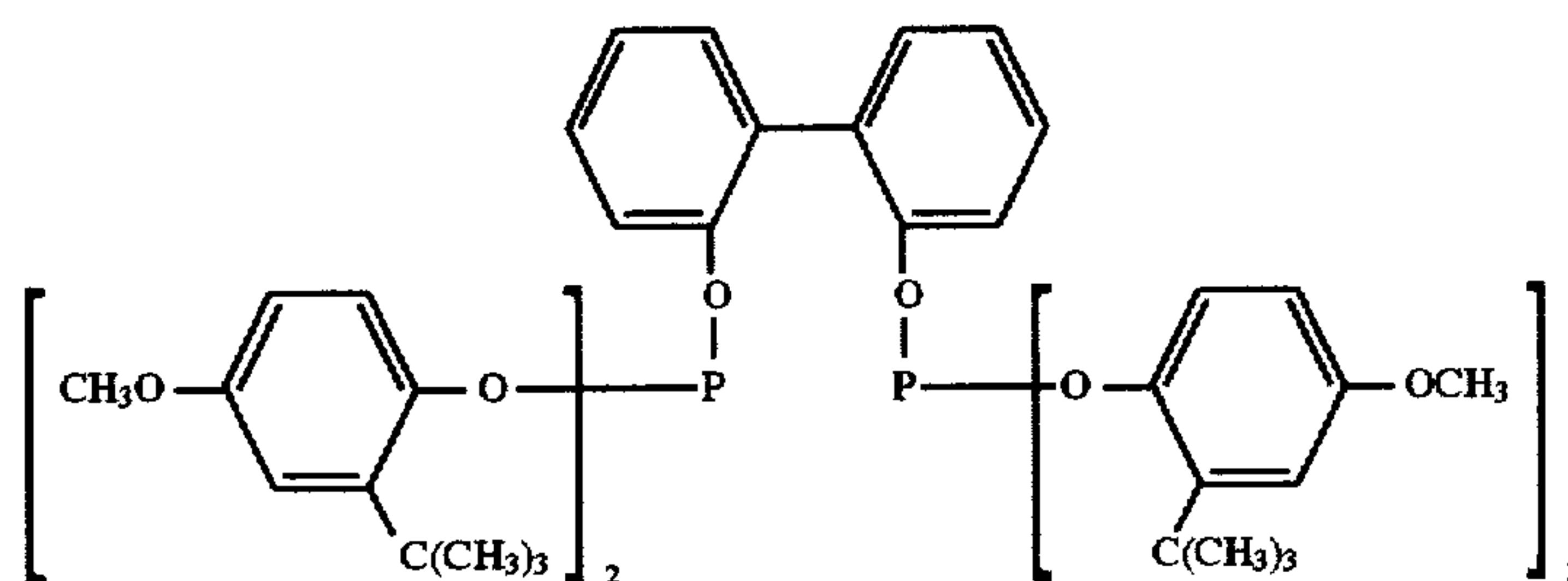
Ligand T
