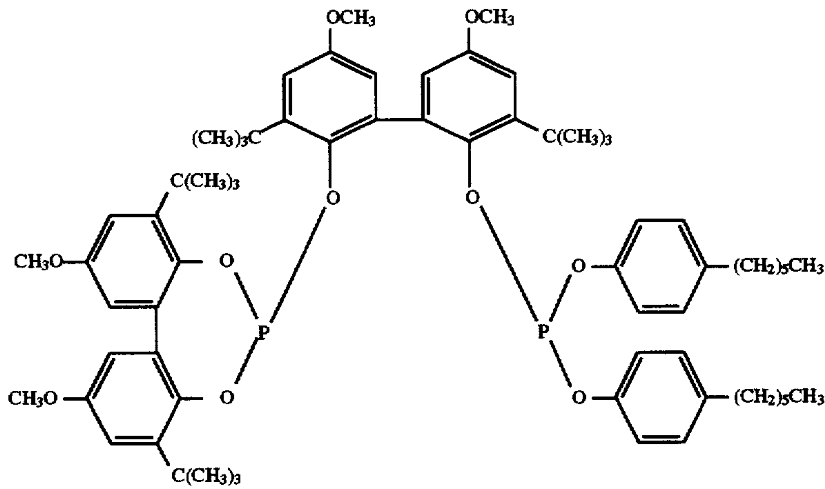
Ligand O
