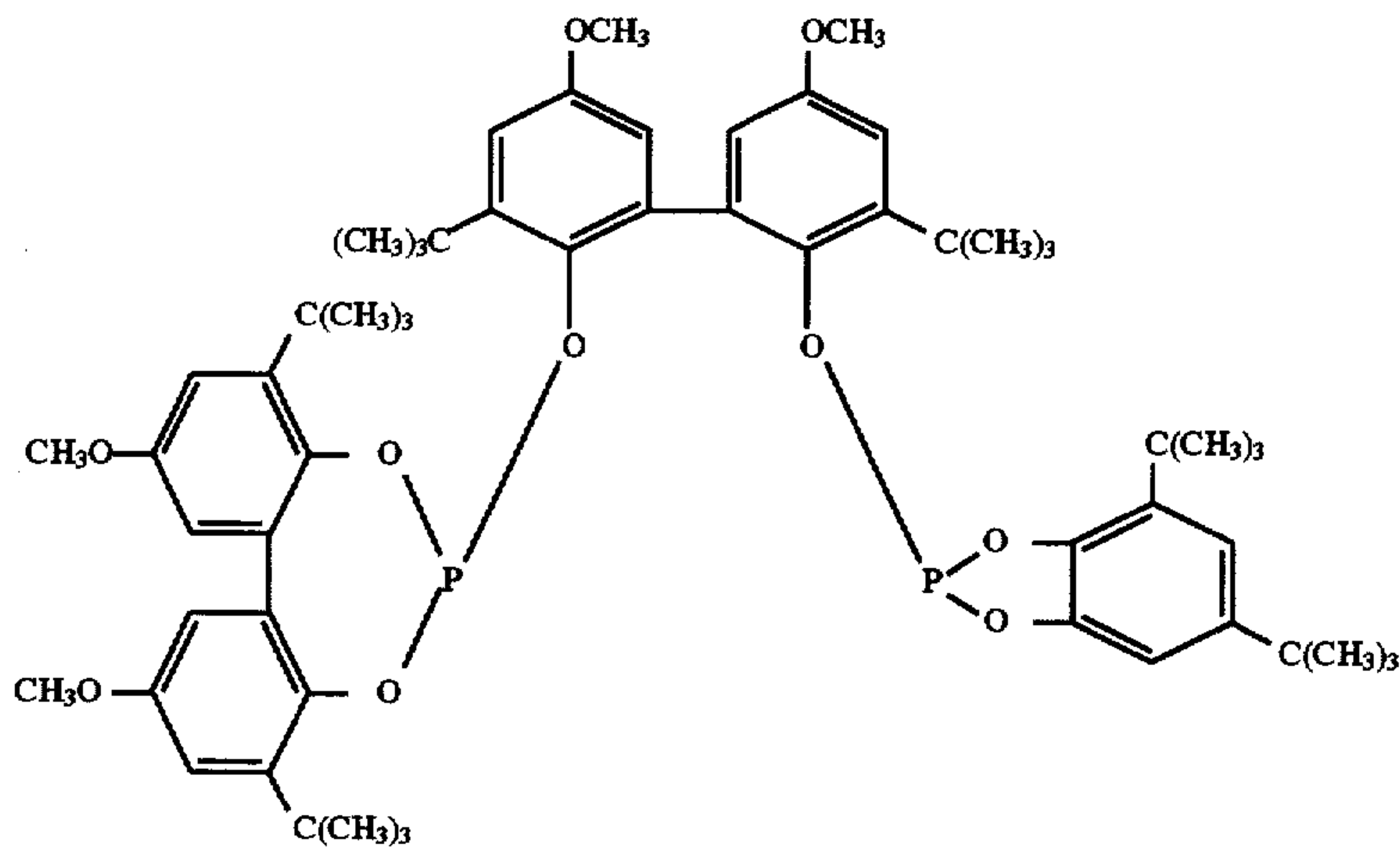
Ligand L
