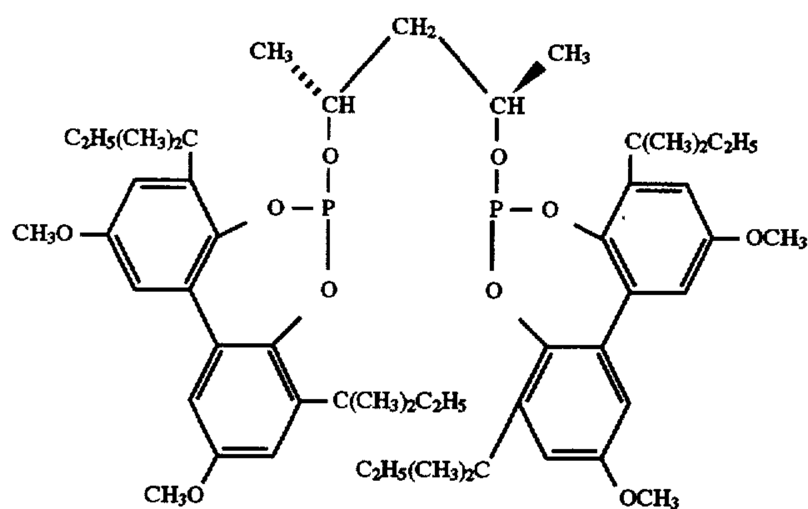
Ligand G
