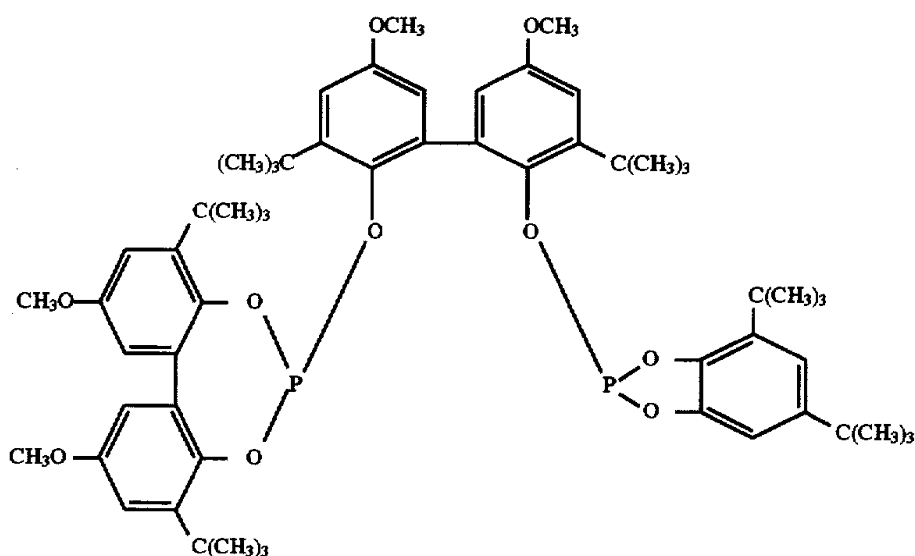
Ligand L
