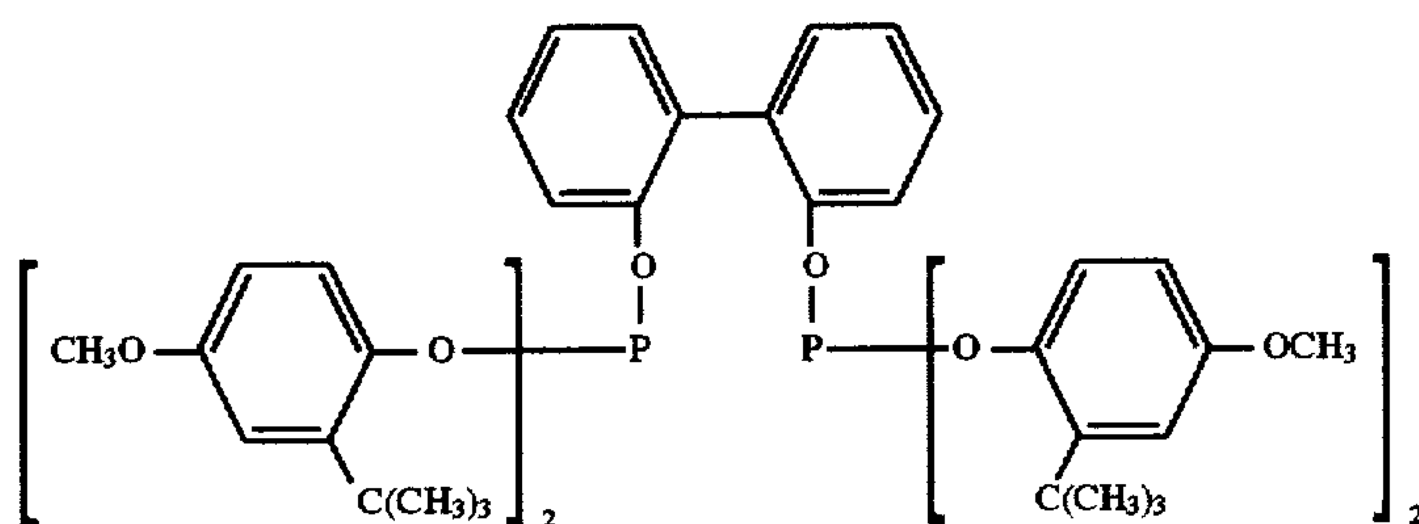
Ligand T
