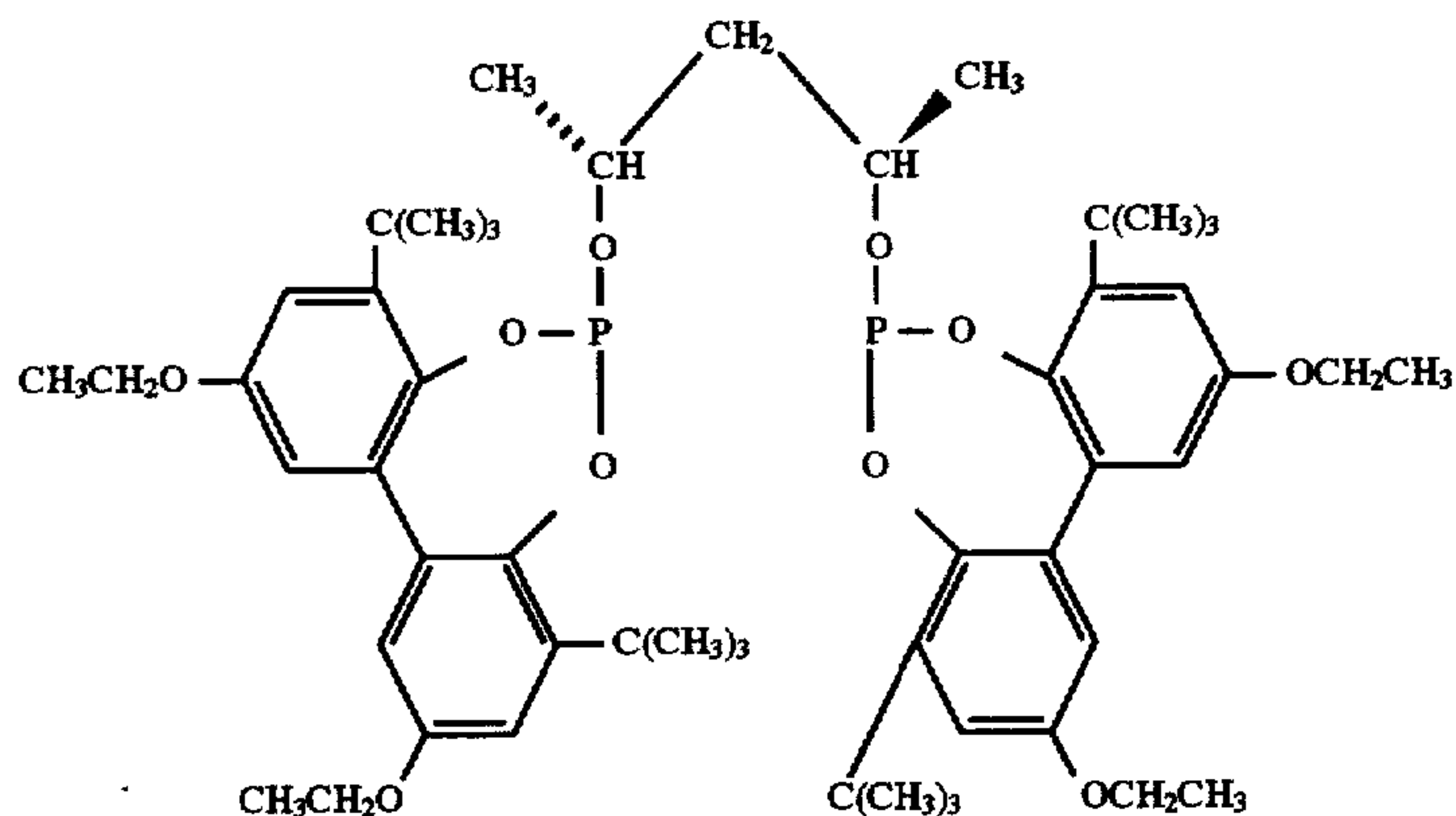
Ligand I
