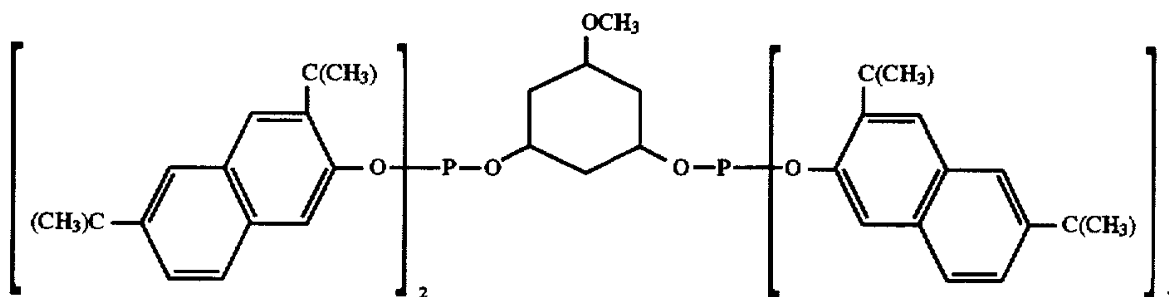
Ligand Q
