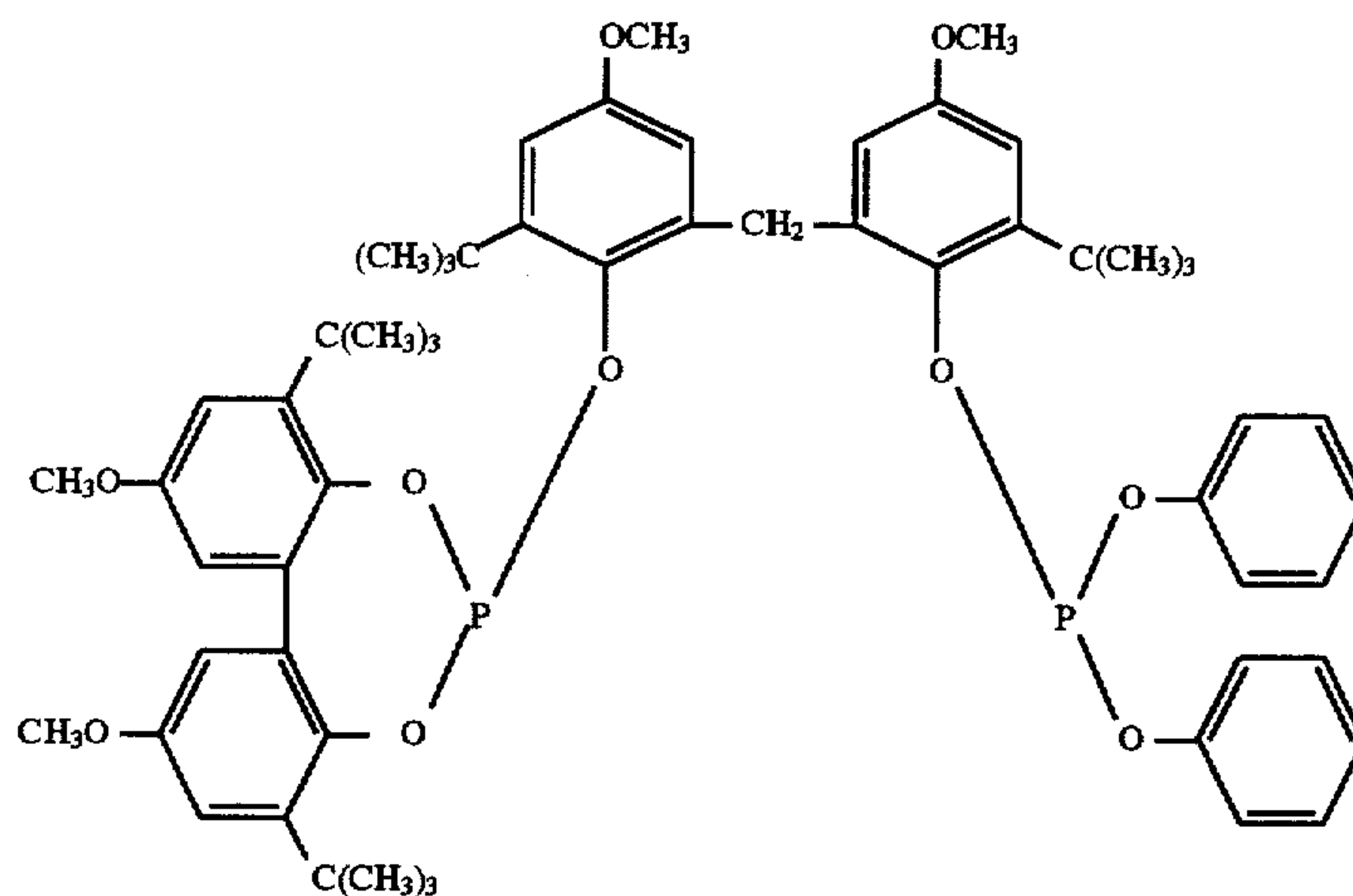
Ligand P
