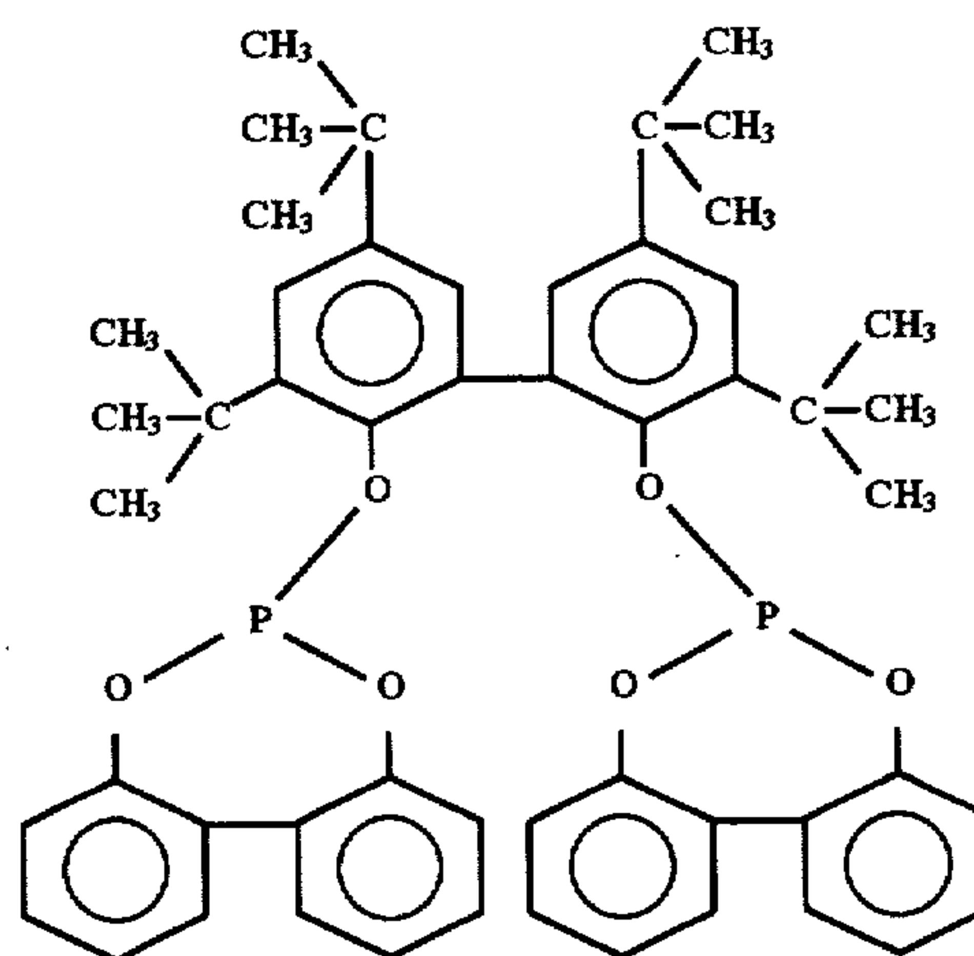
Ligand D
