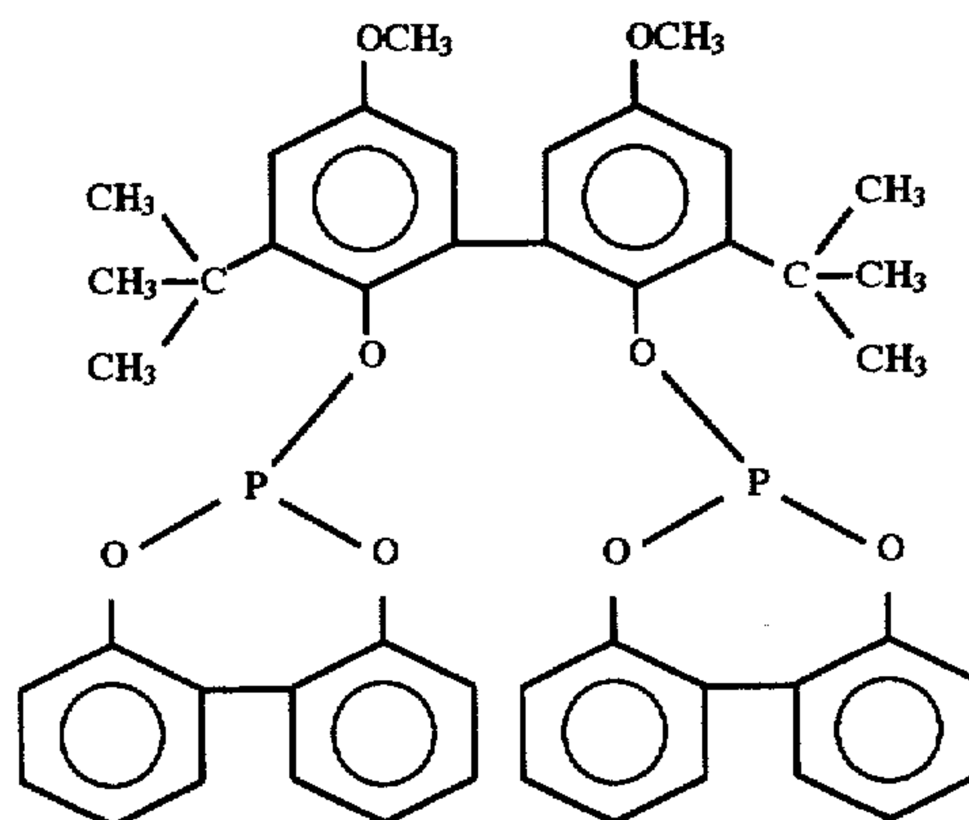
Ligand B
