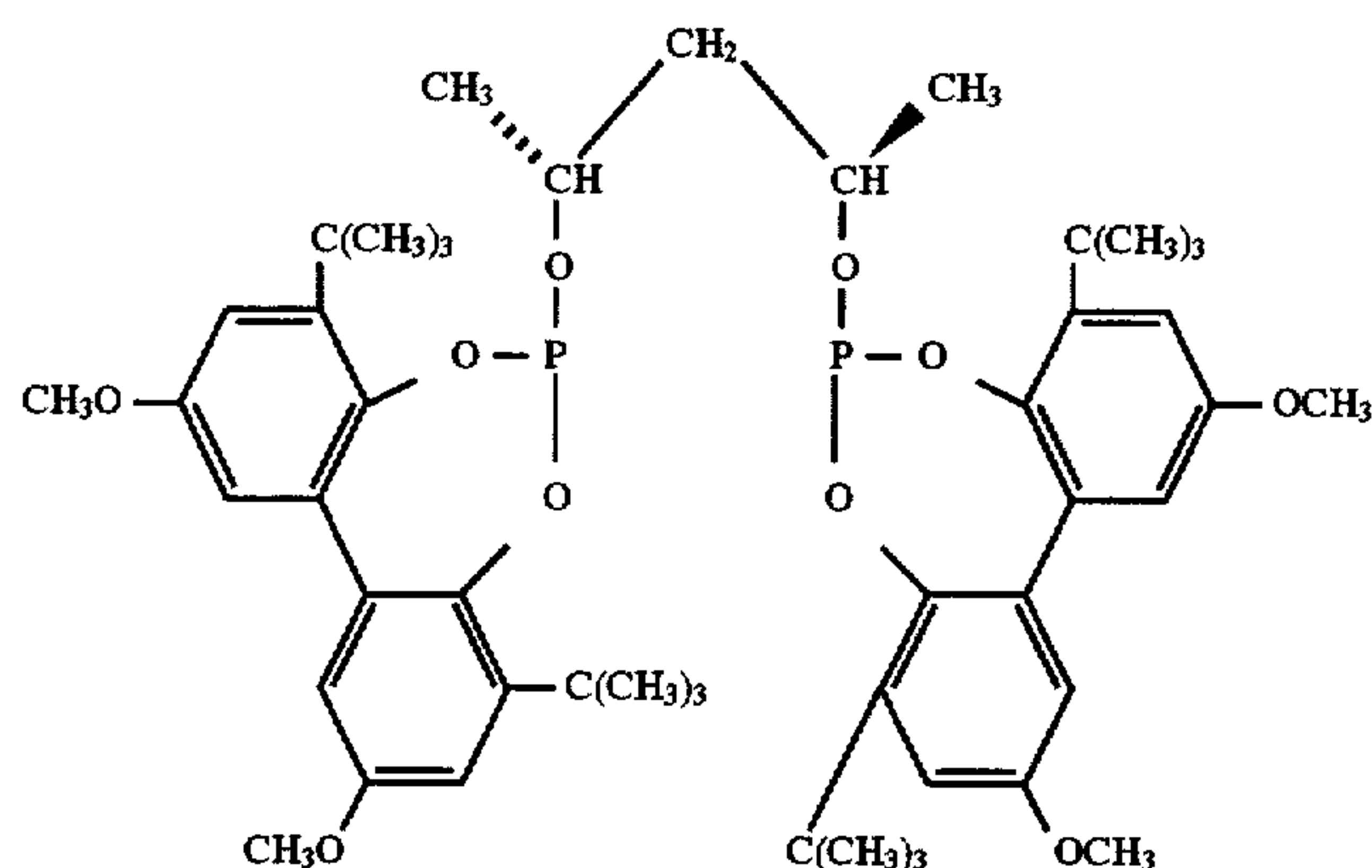
Ligand K
