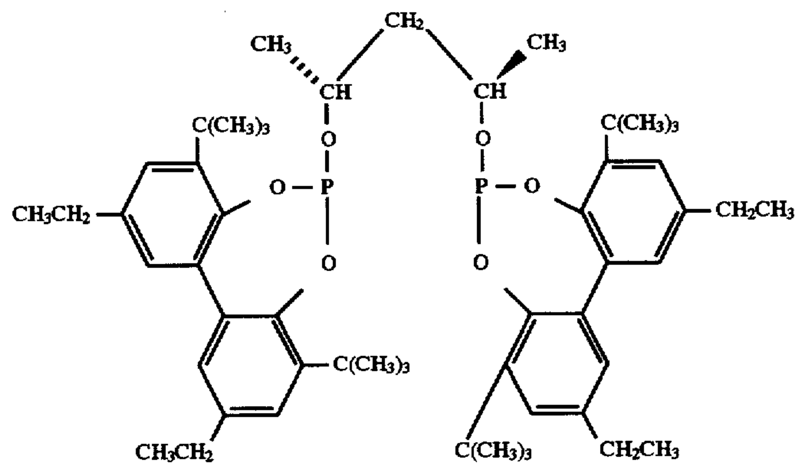
Ligand J
