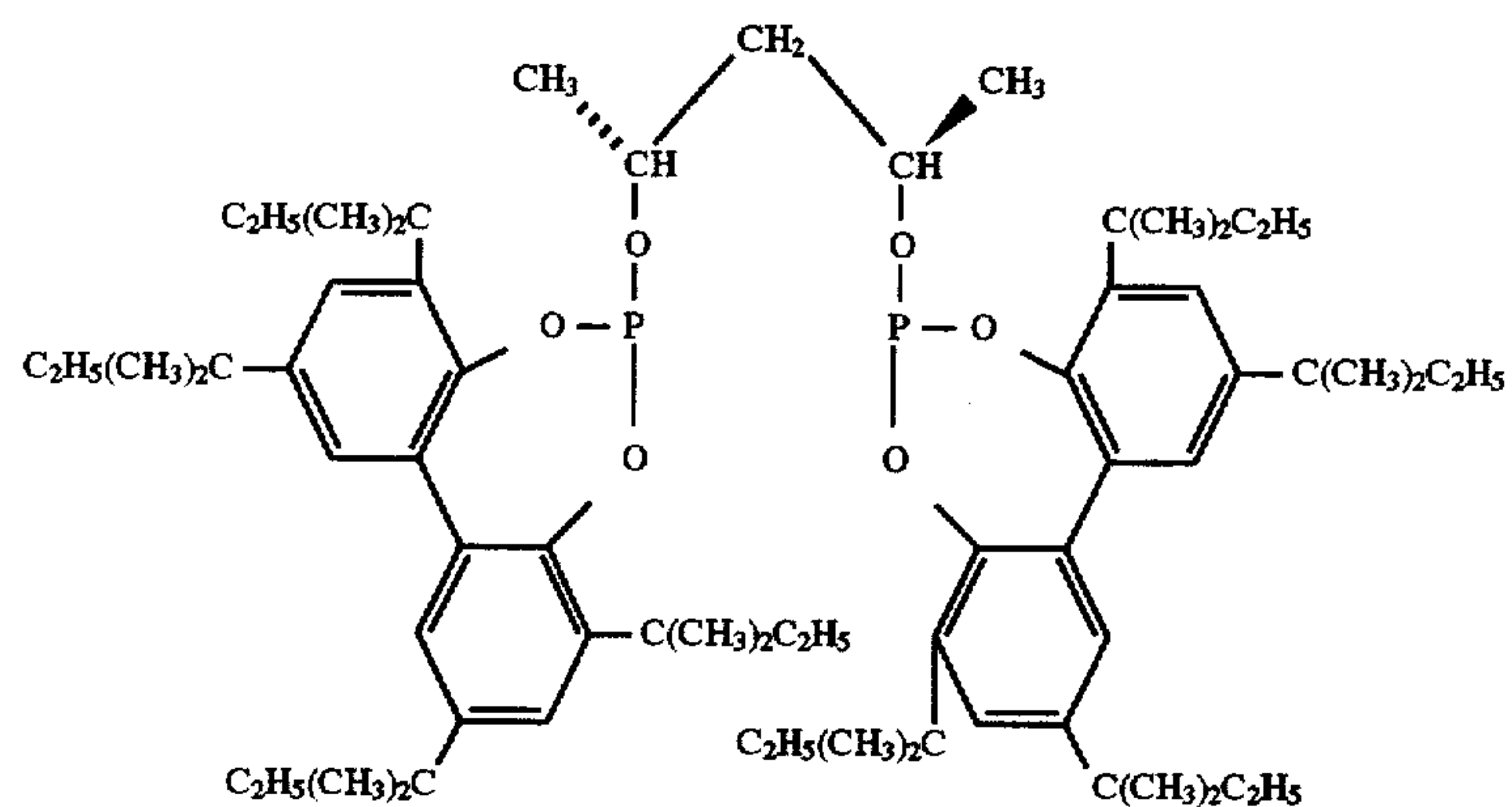
Ligand E
