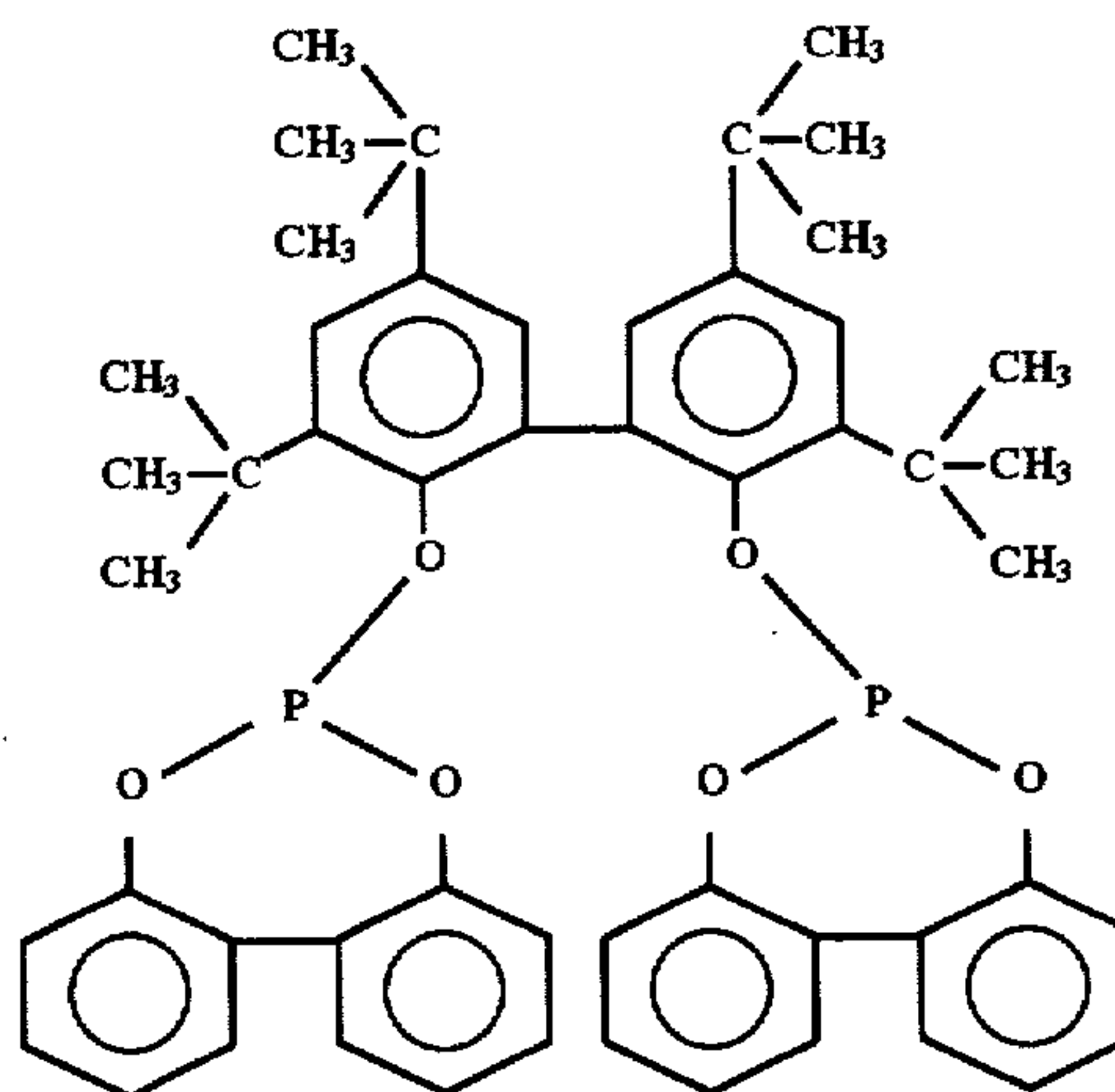
Ligand D
