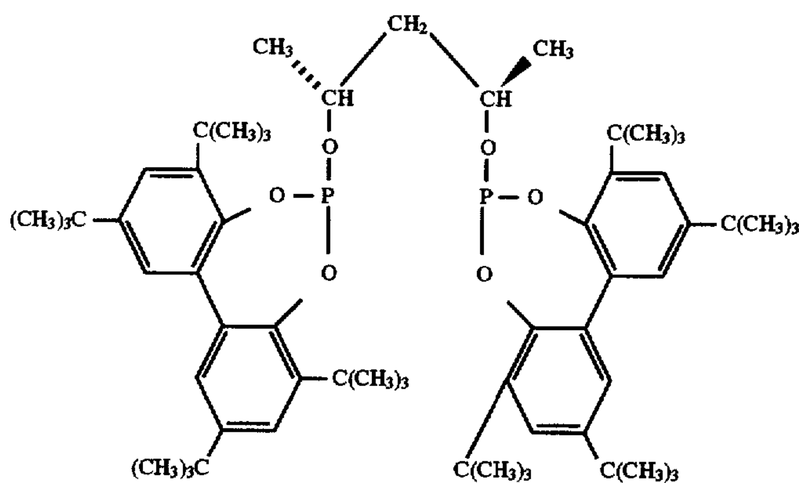
Ligand F
