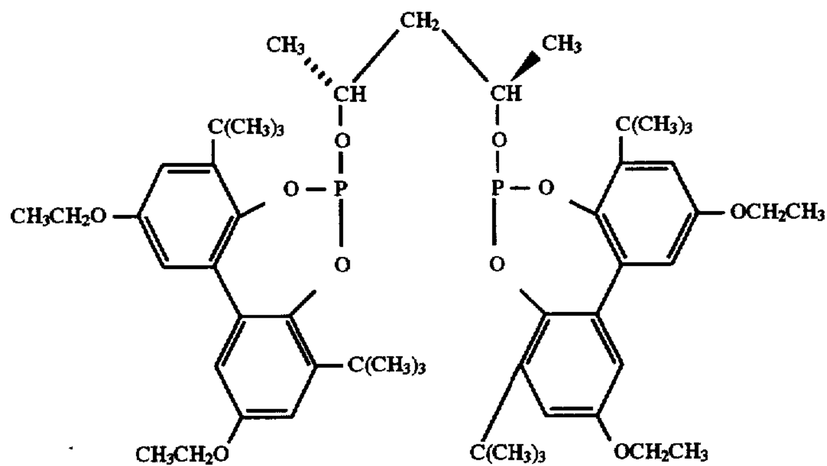
Ligand I
