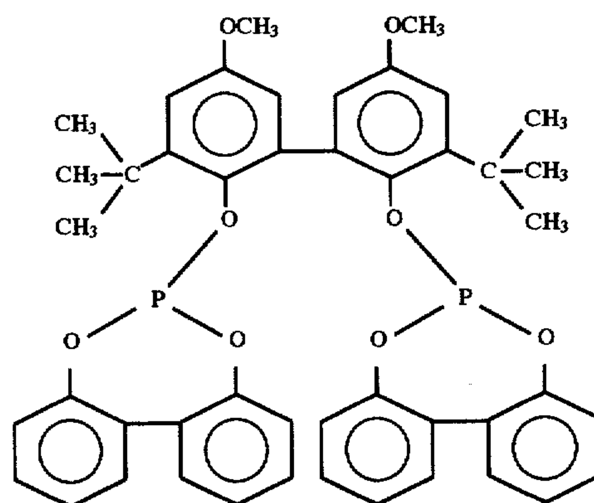
Ligand B
