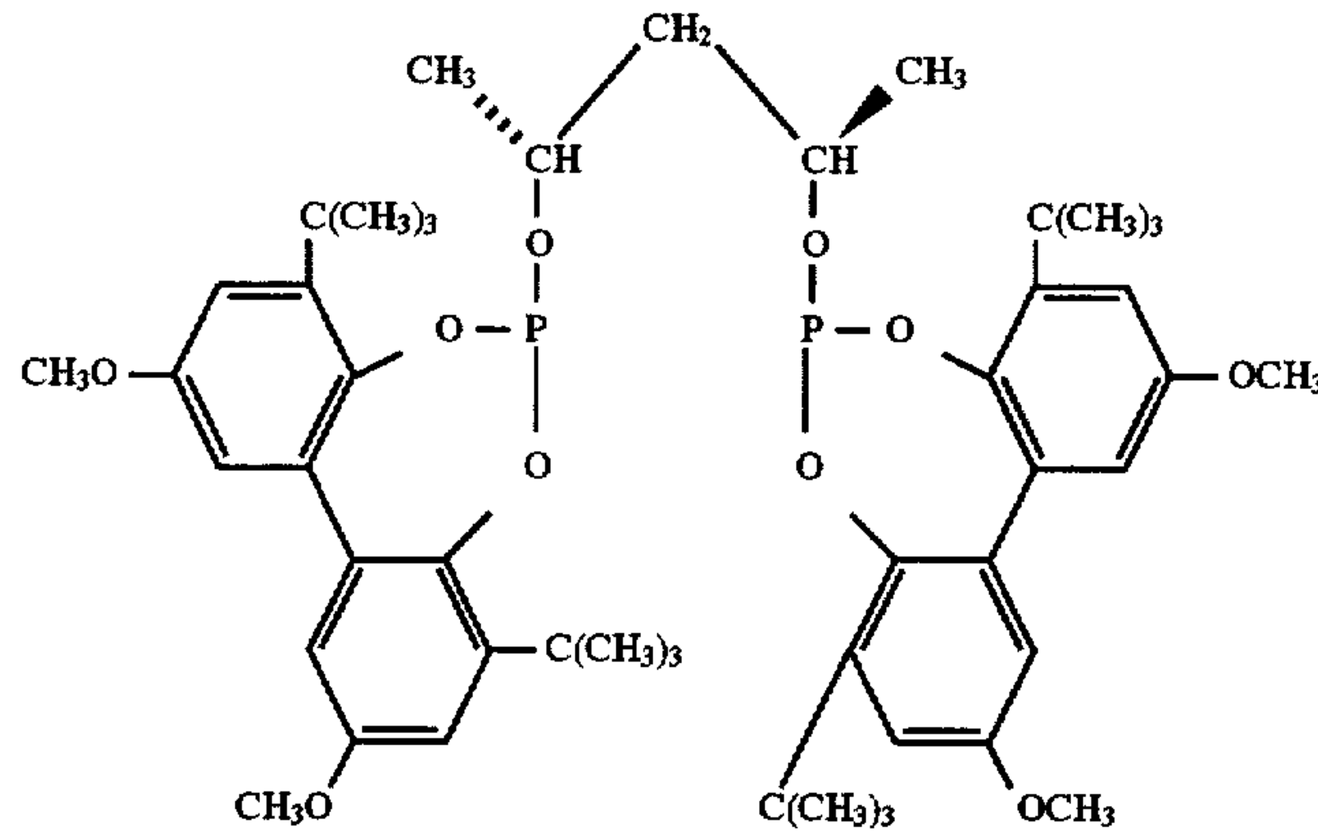
Ligand K
