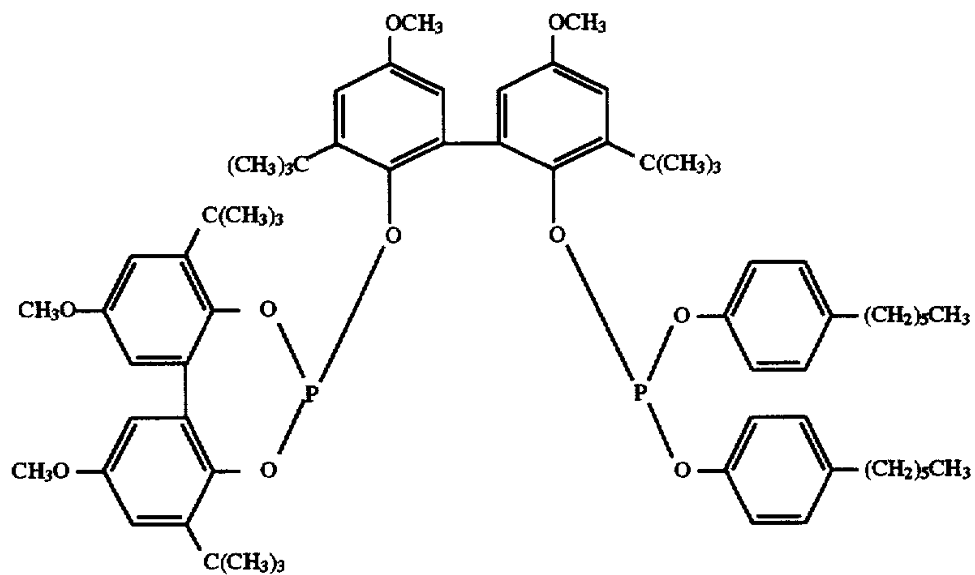
Ligand O
