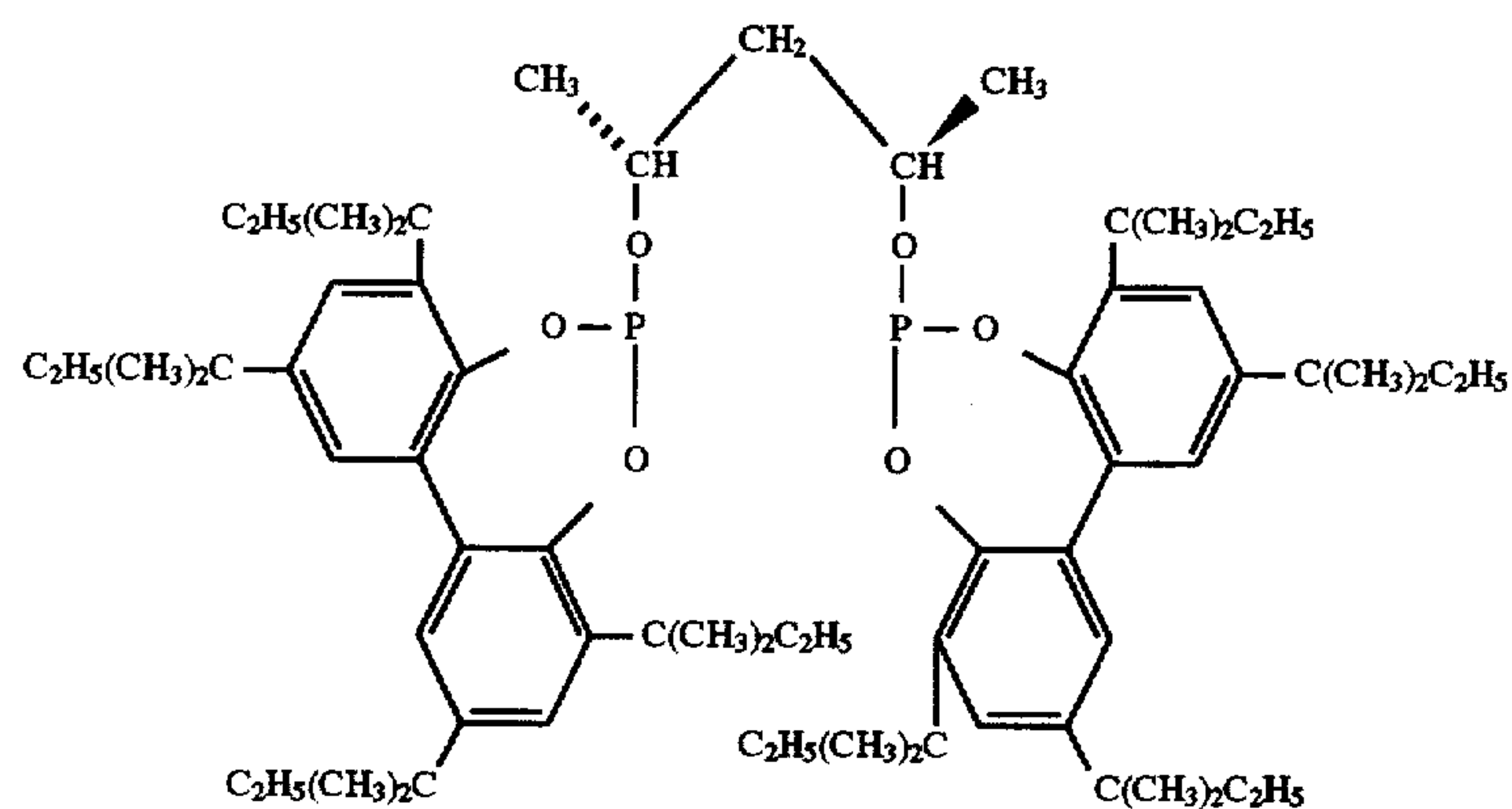
Ligand E
