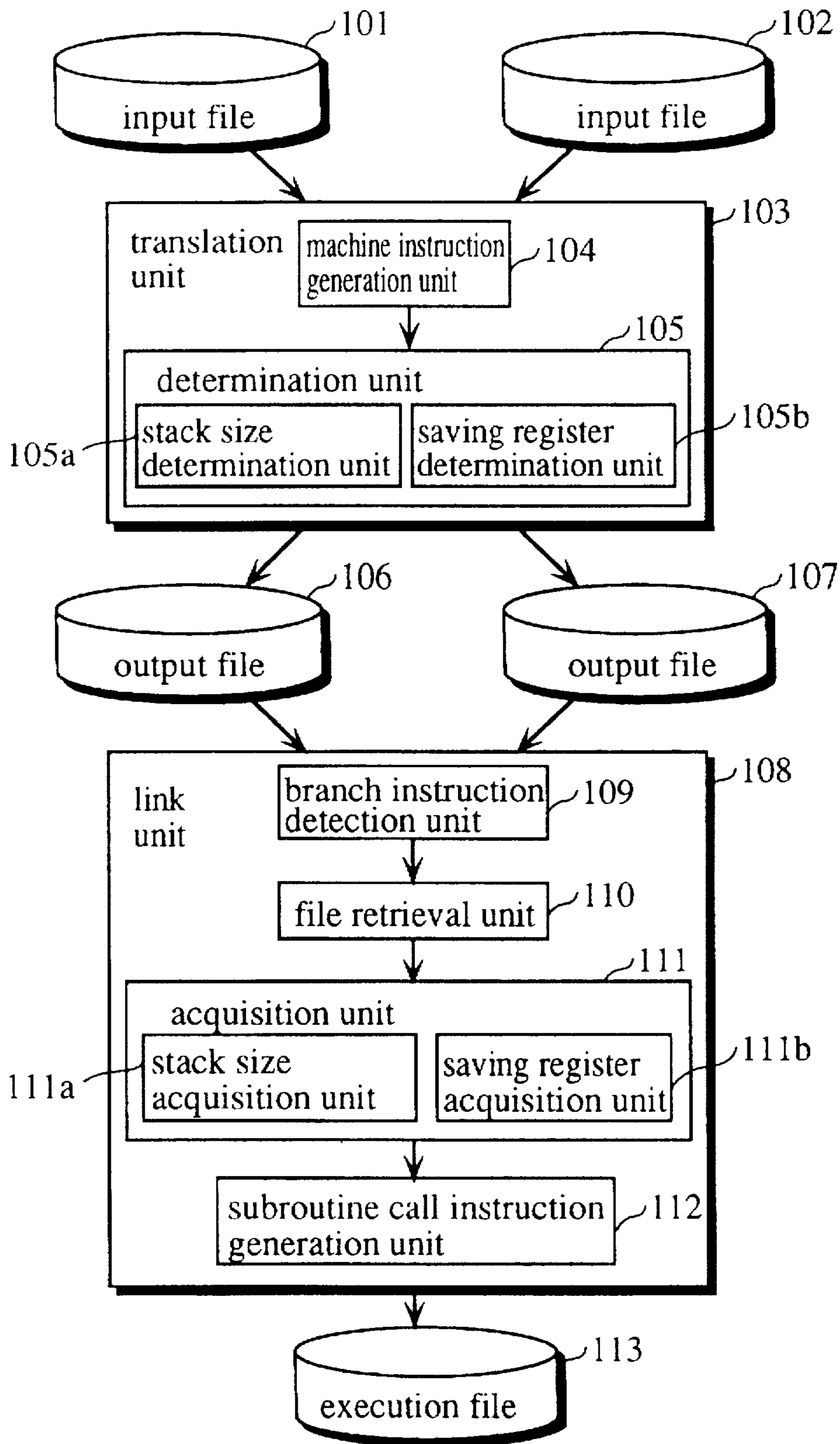
FIG. 5
