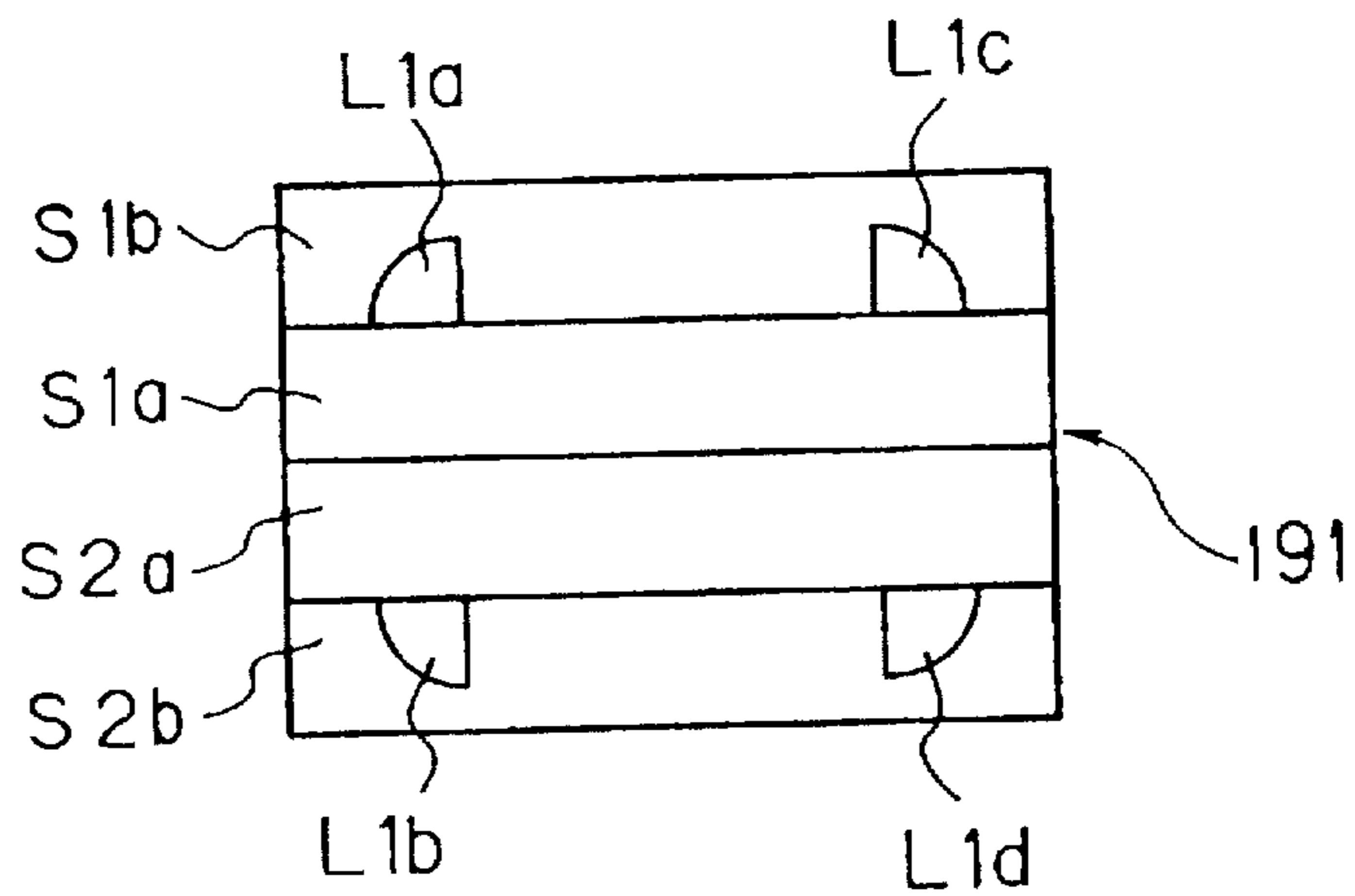
FIG. 10B
