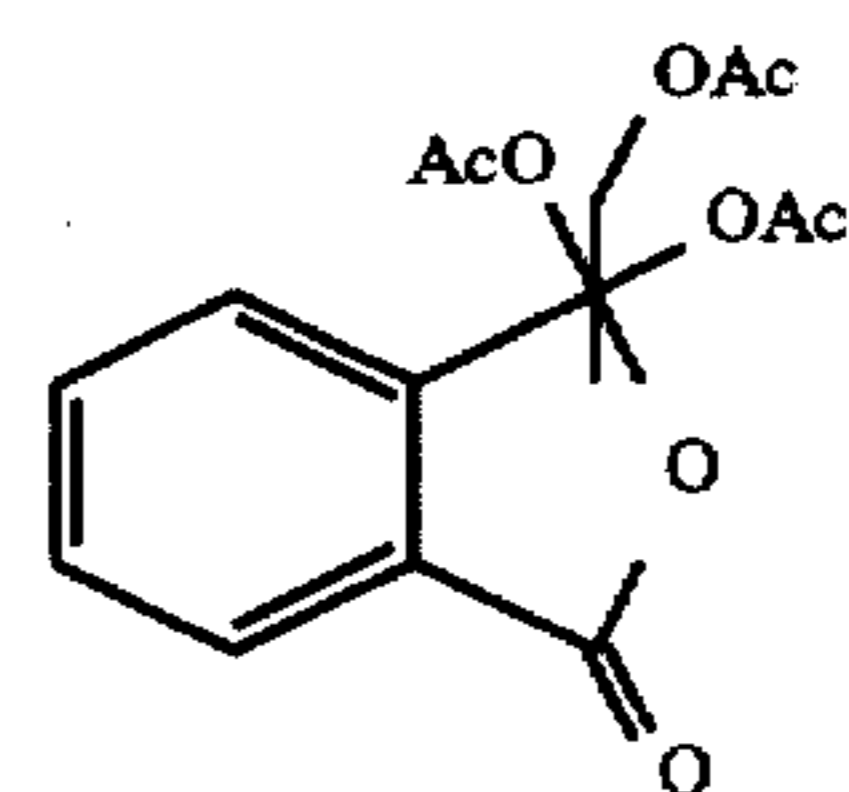
Dess-Martin periodinane
