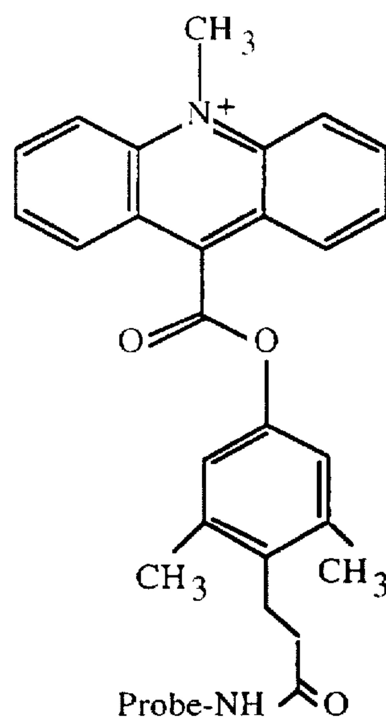
m -diMe-AE
