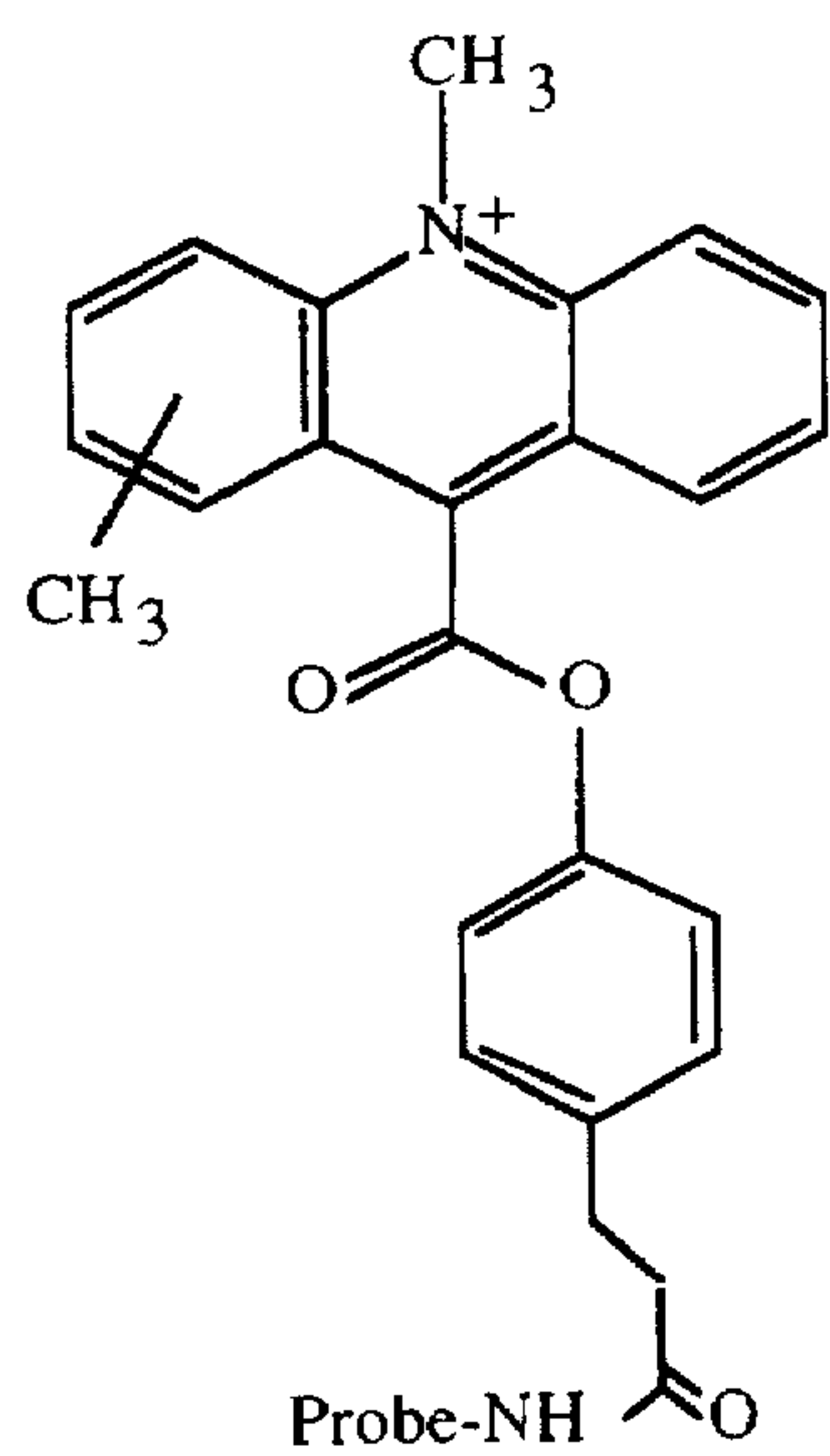
1 or 3-Me-AE
