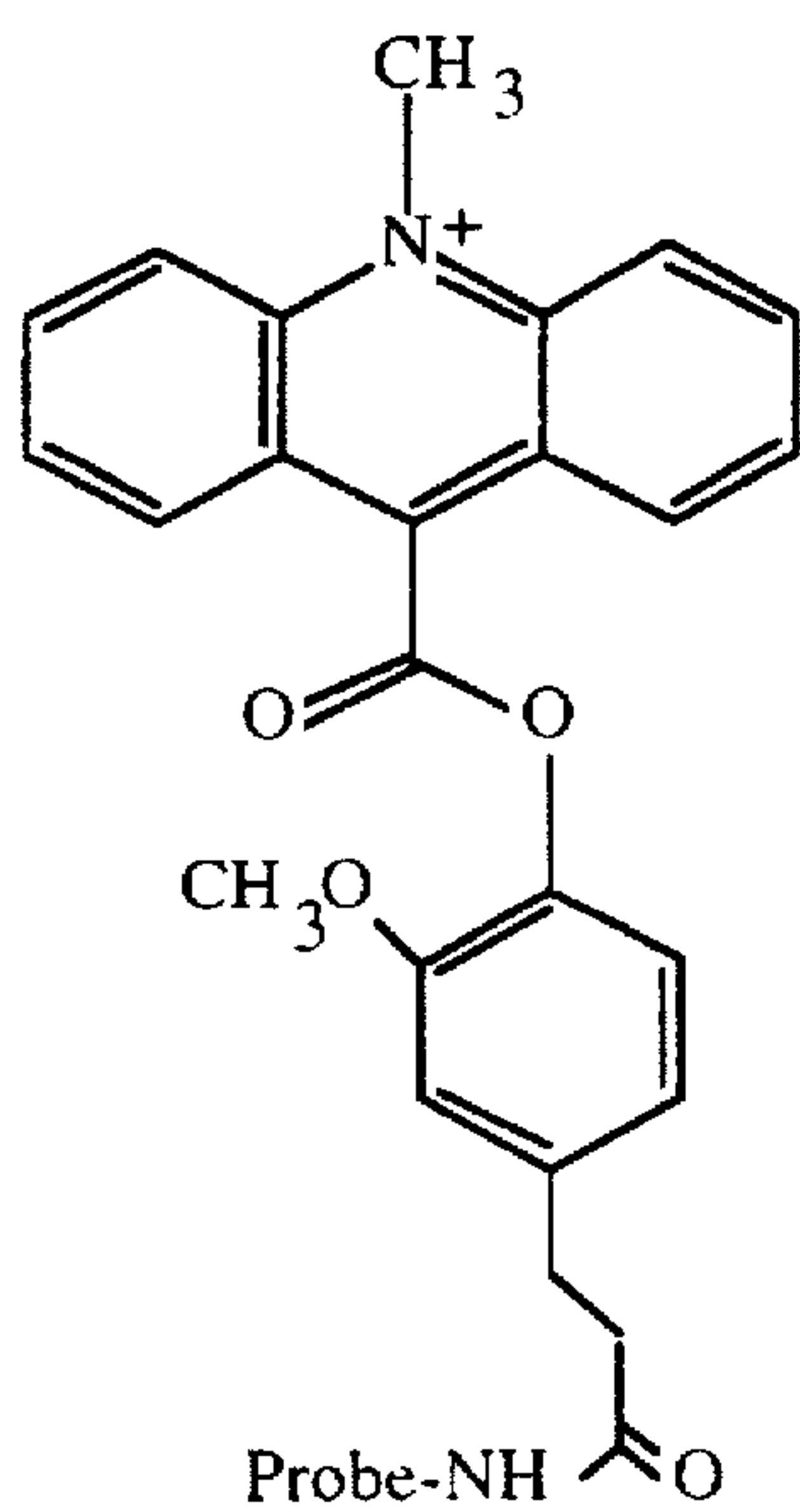
o -MeO-AE
