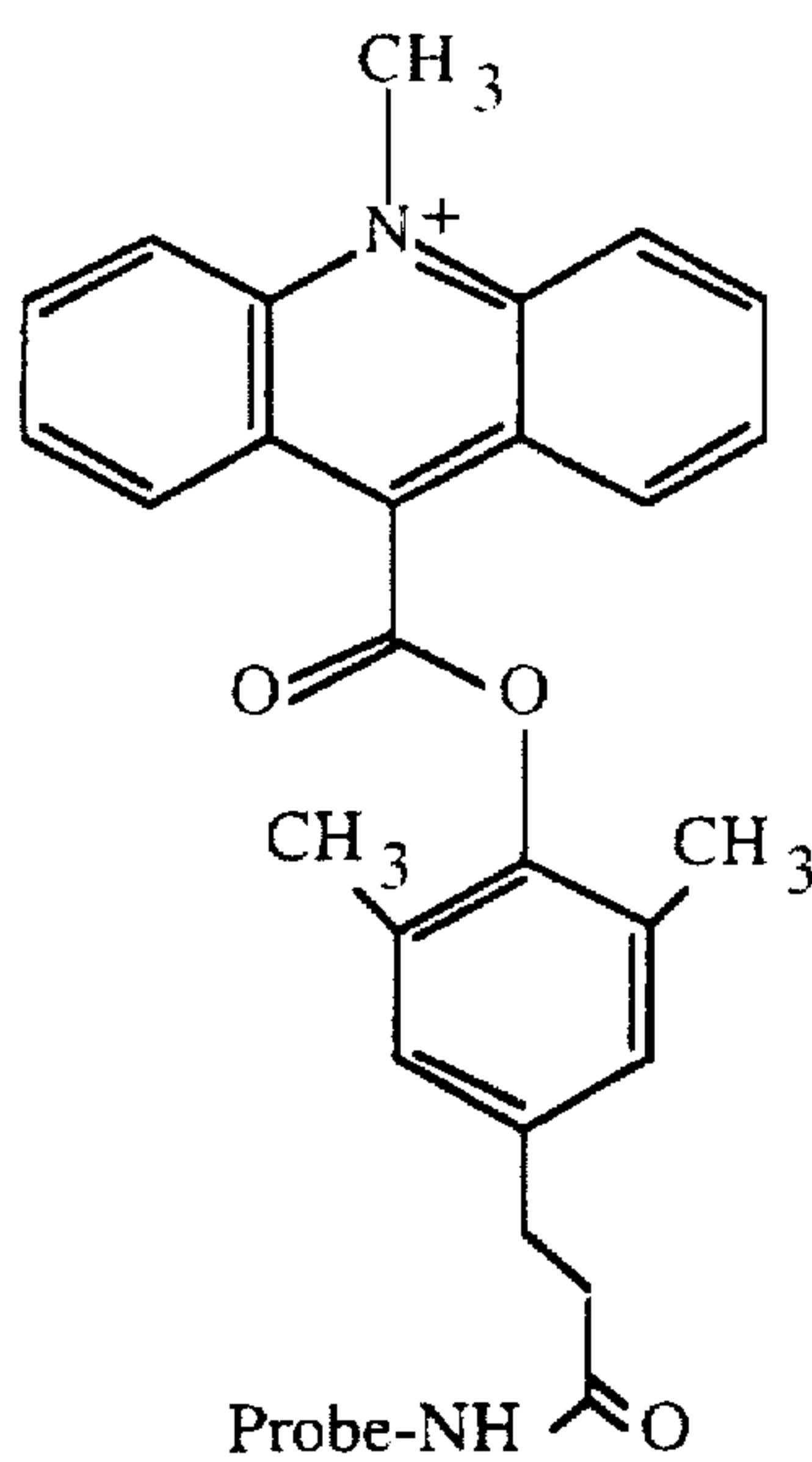
o -diMe-AE
