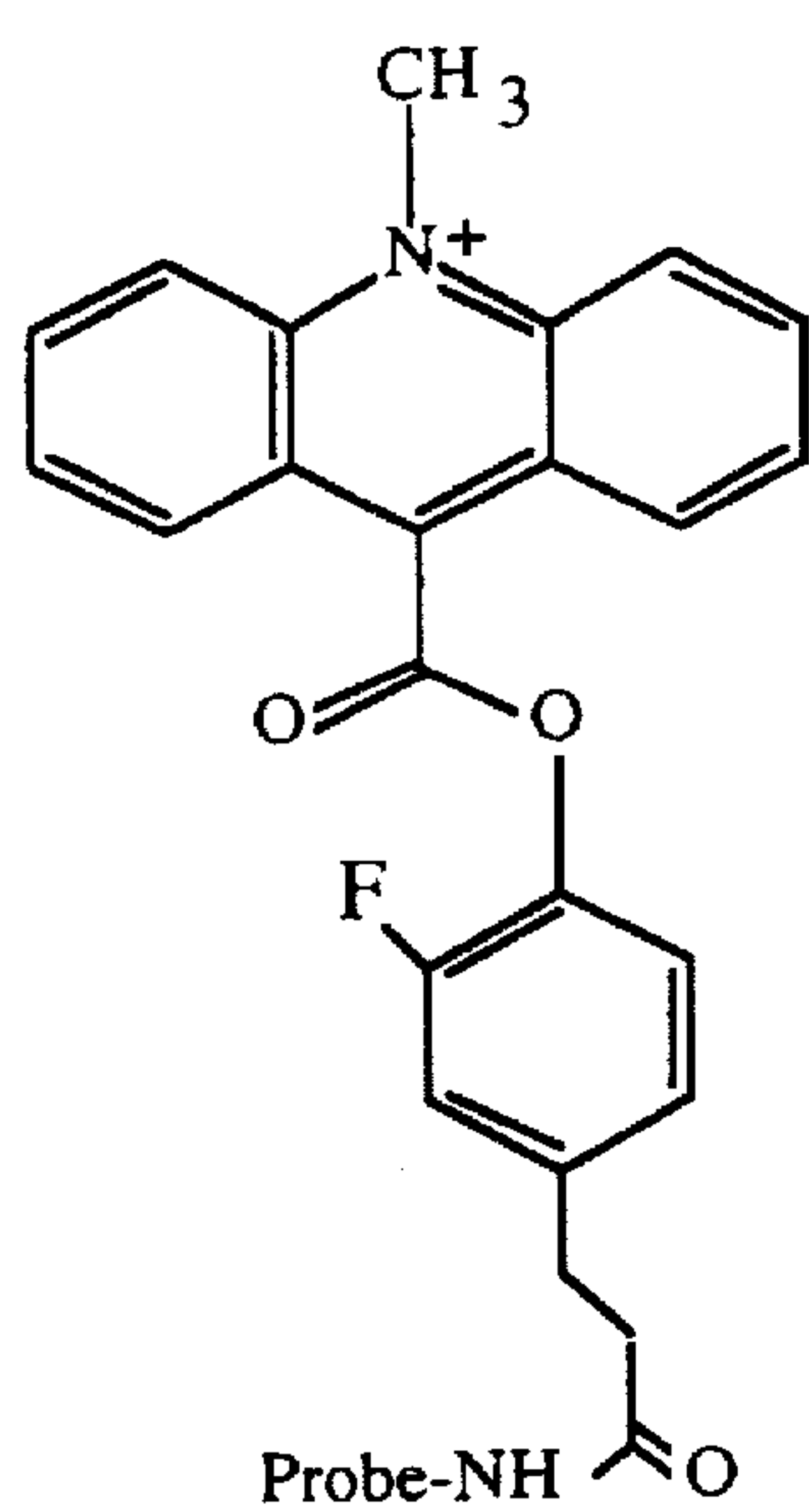
o -F-AE
