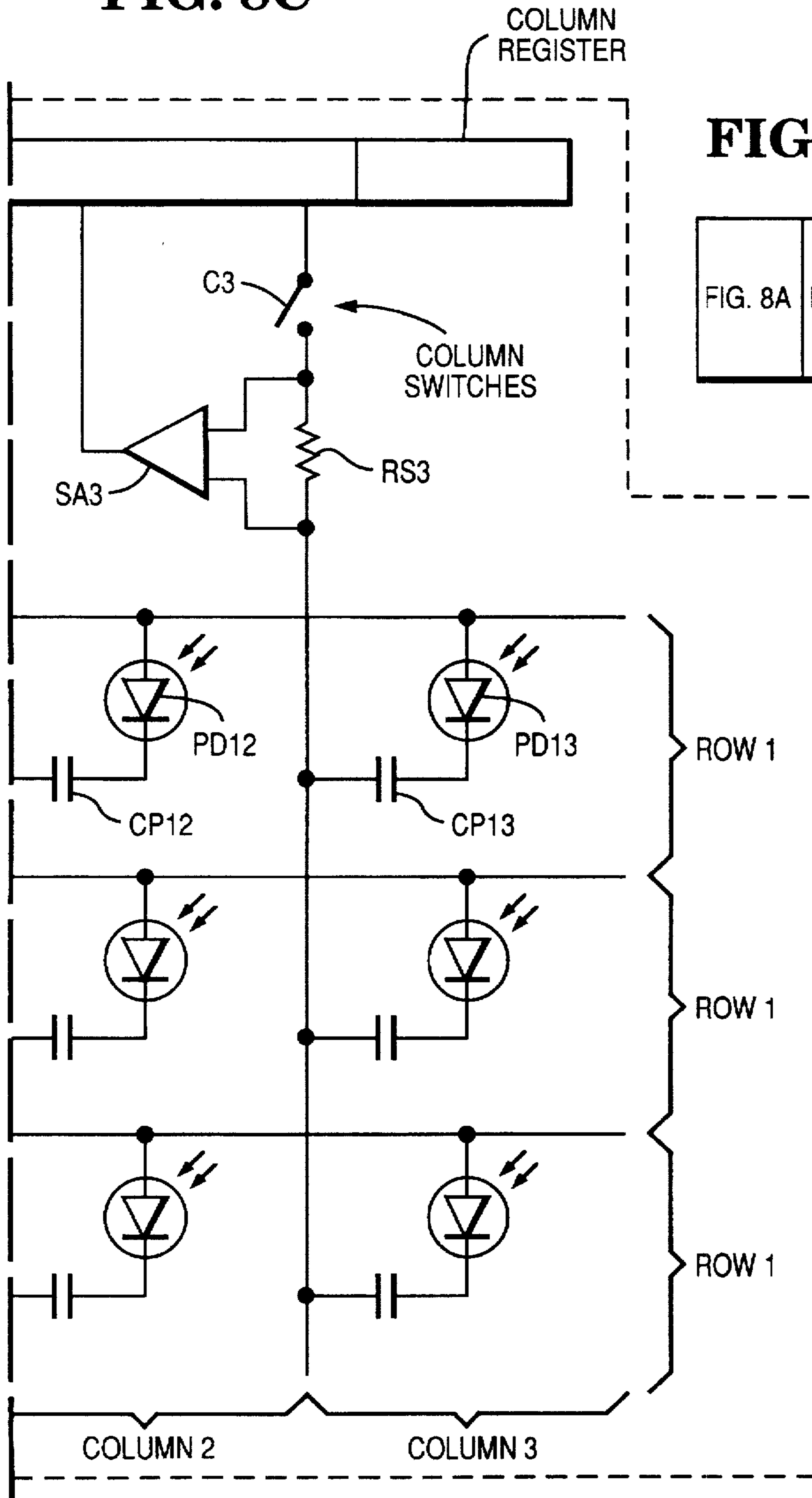
FIG. 8C
