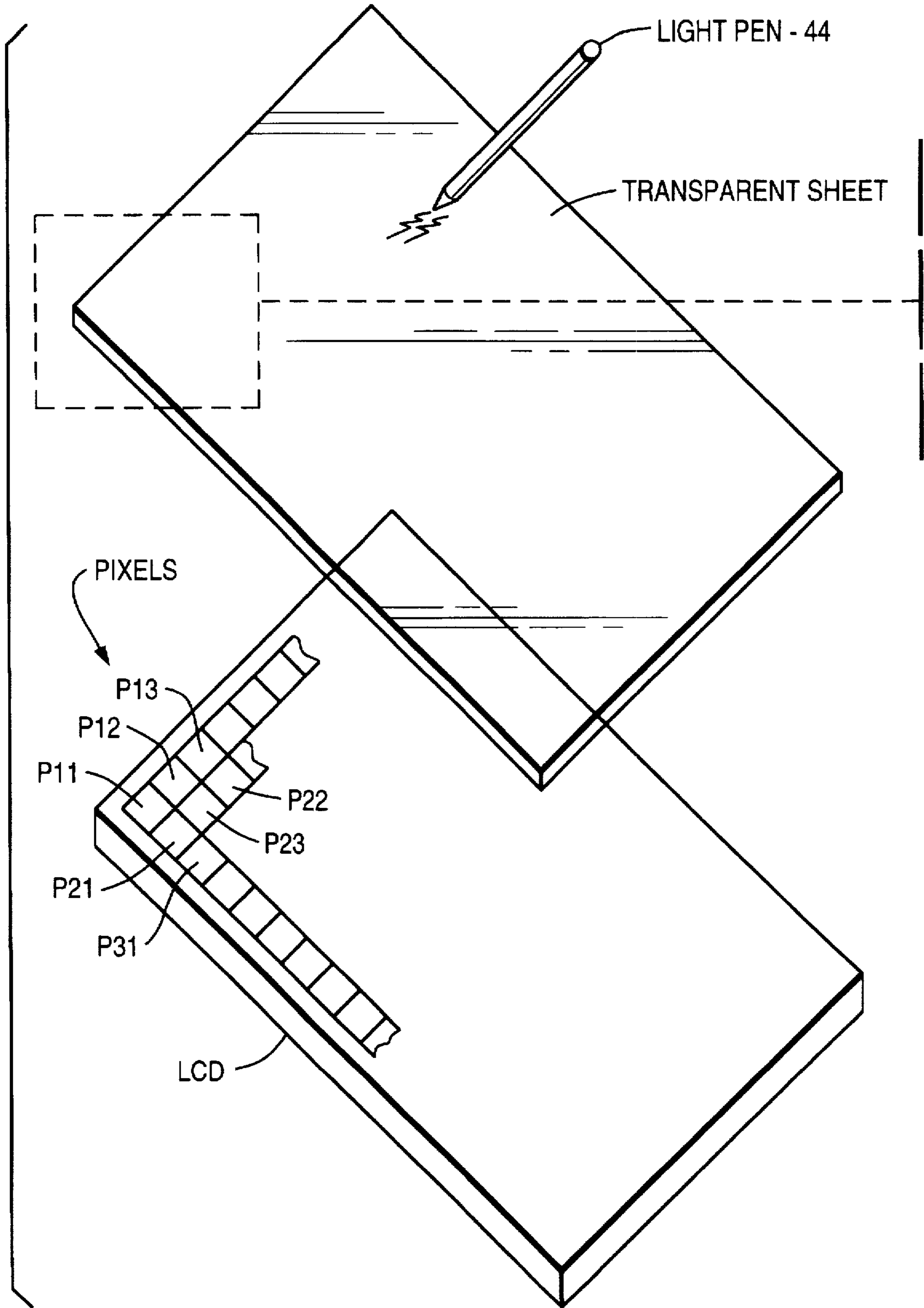
FIG. 8A
