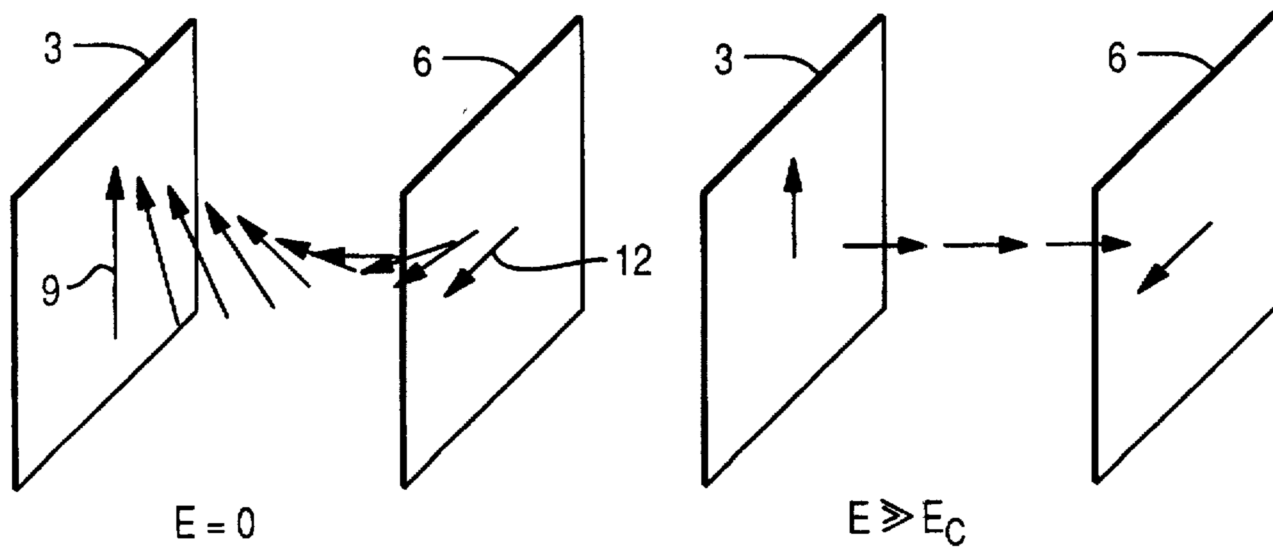
FIG. 3A
