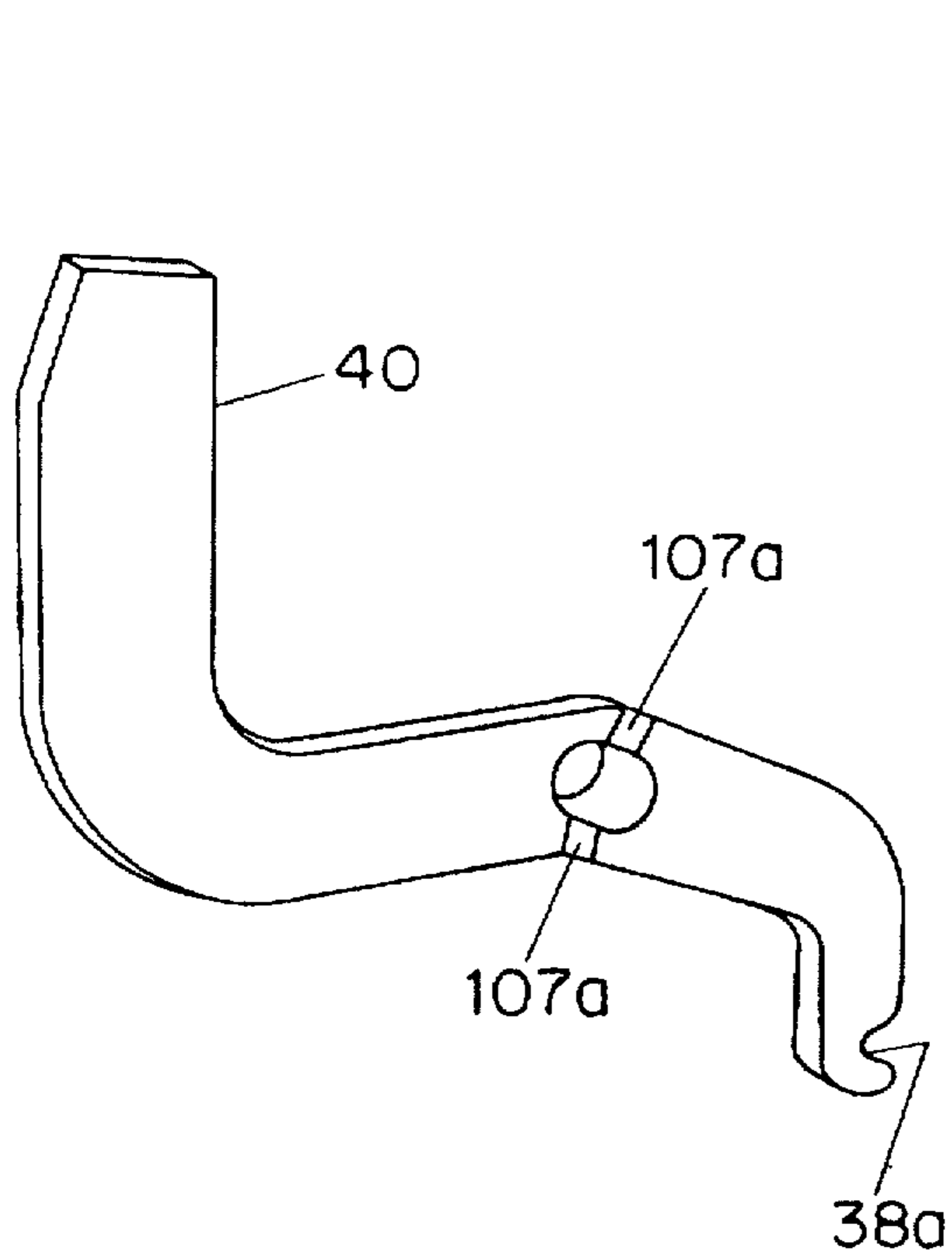
FIG. 13
