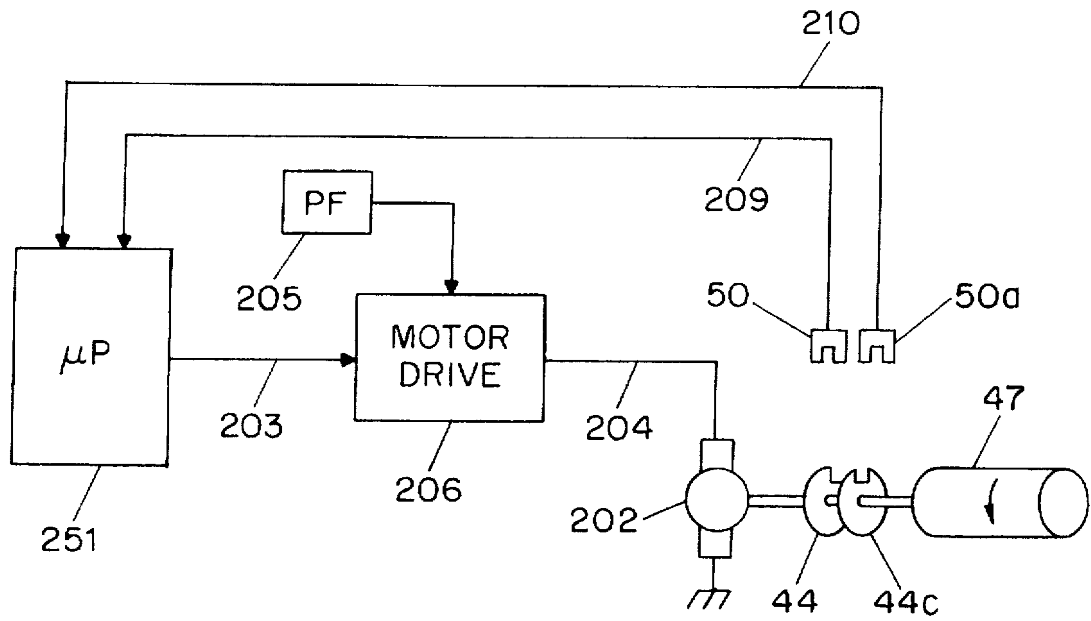
FIG. 19
