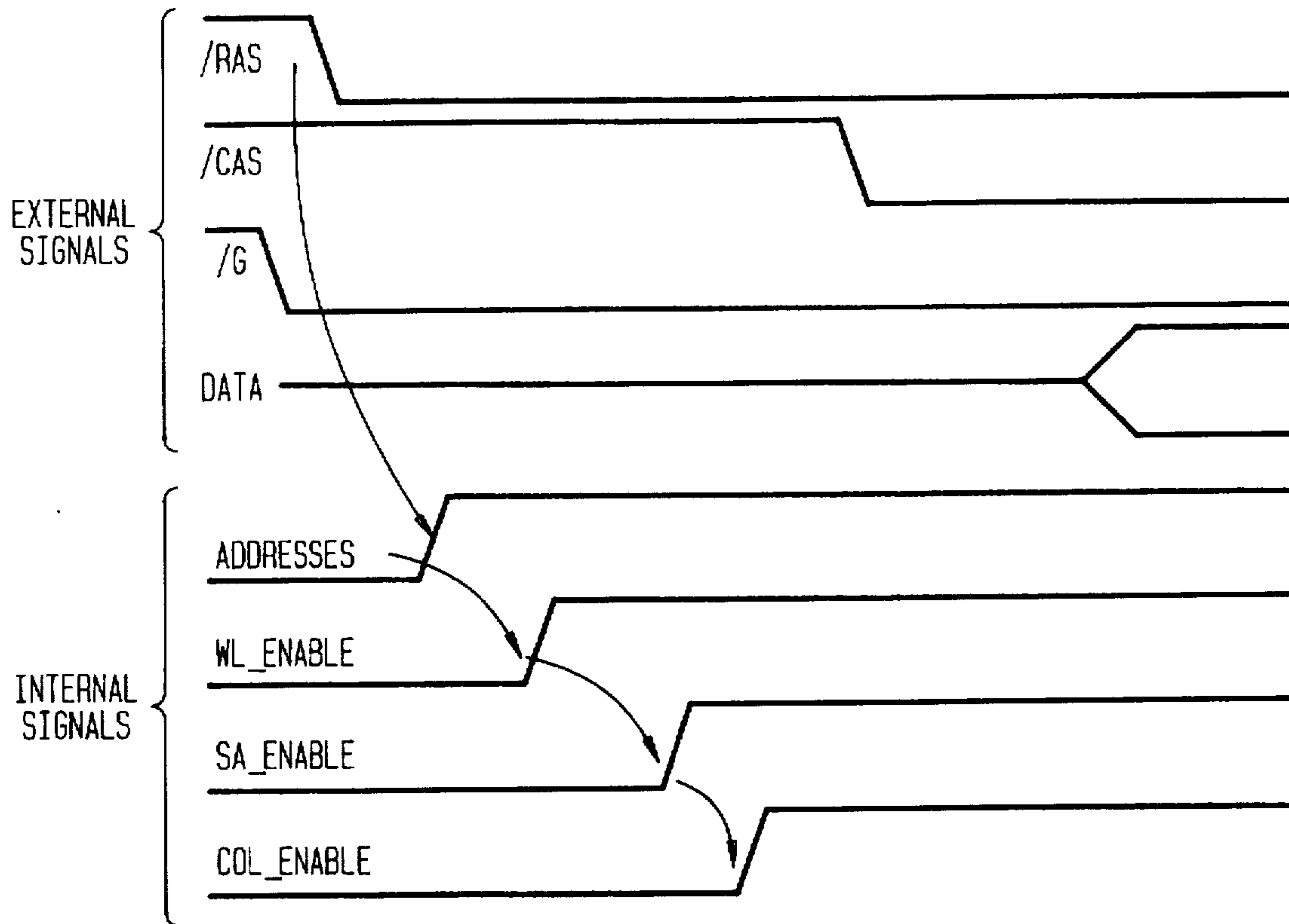
FIG. 3A
