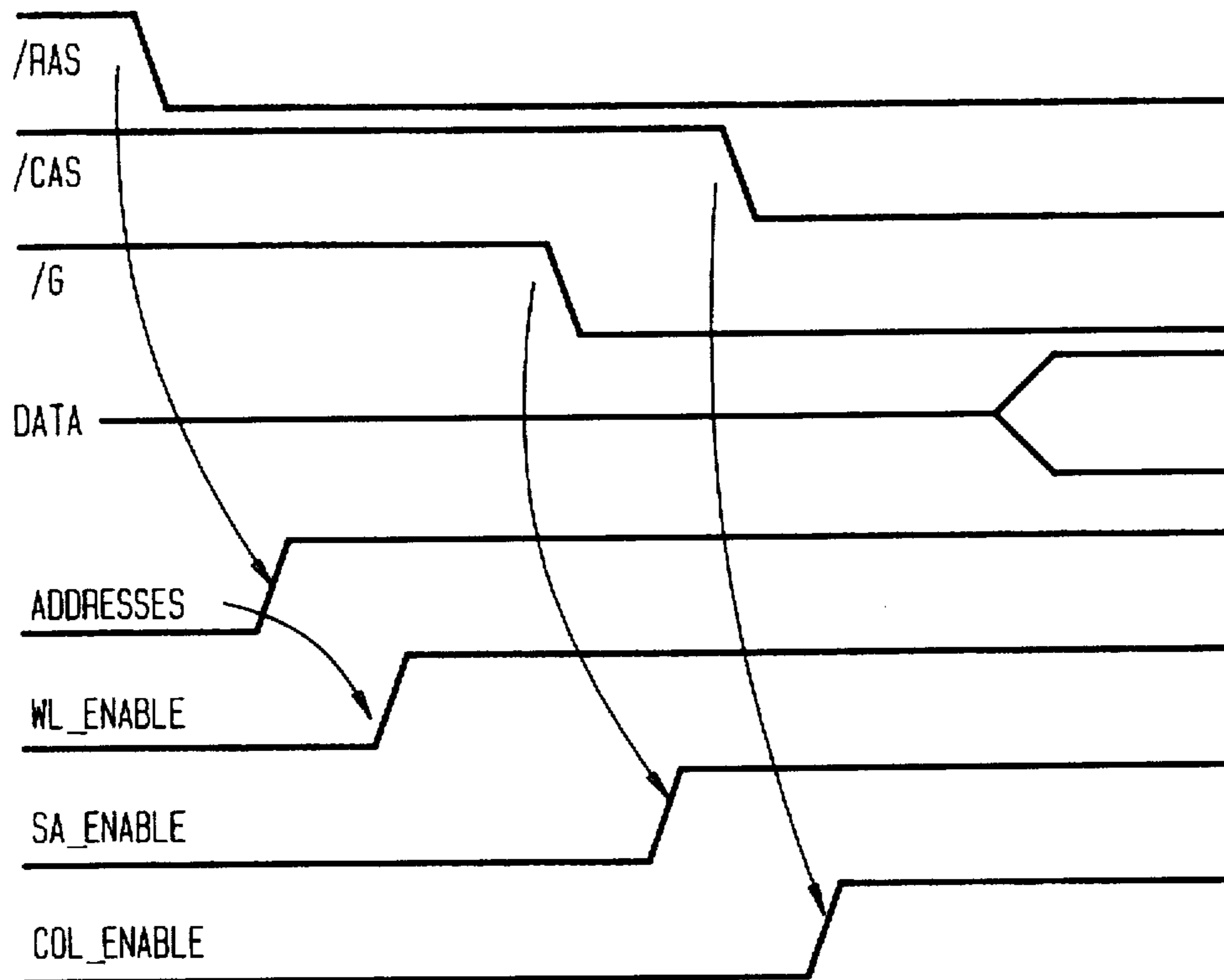
FIG. 3B
