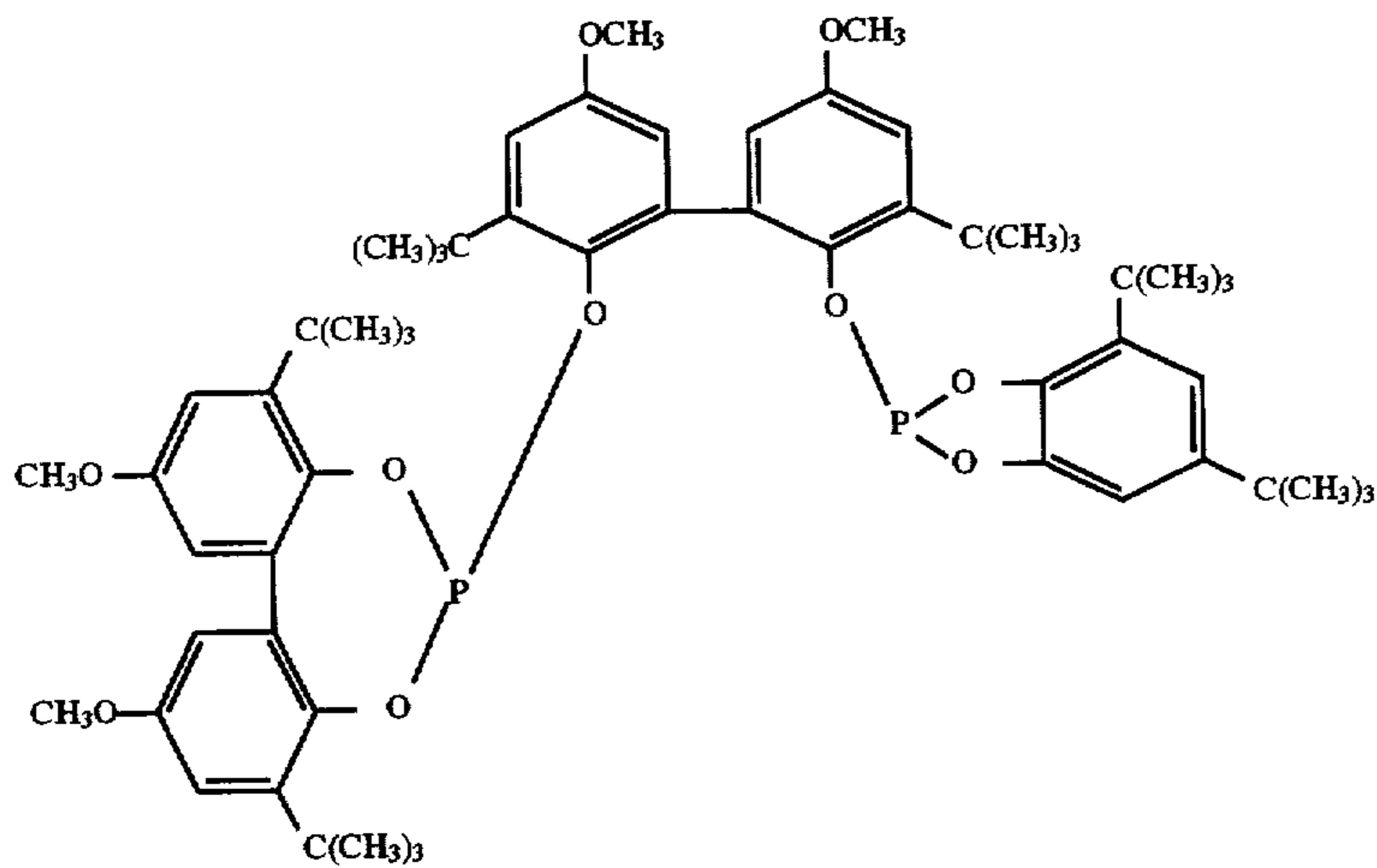
Ligand N
