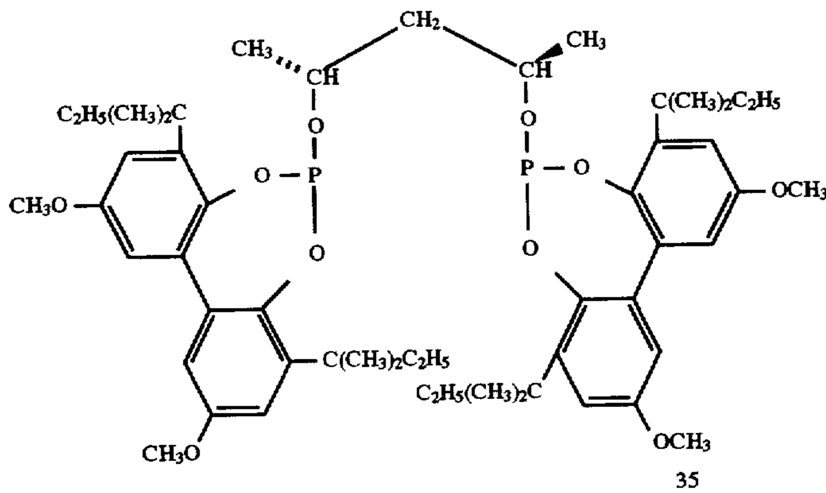
Ligand I
