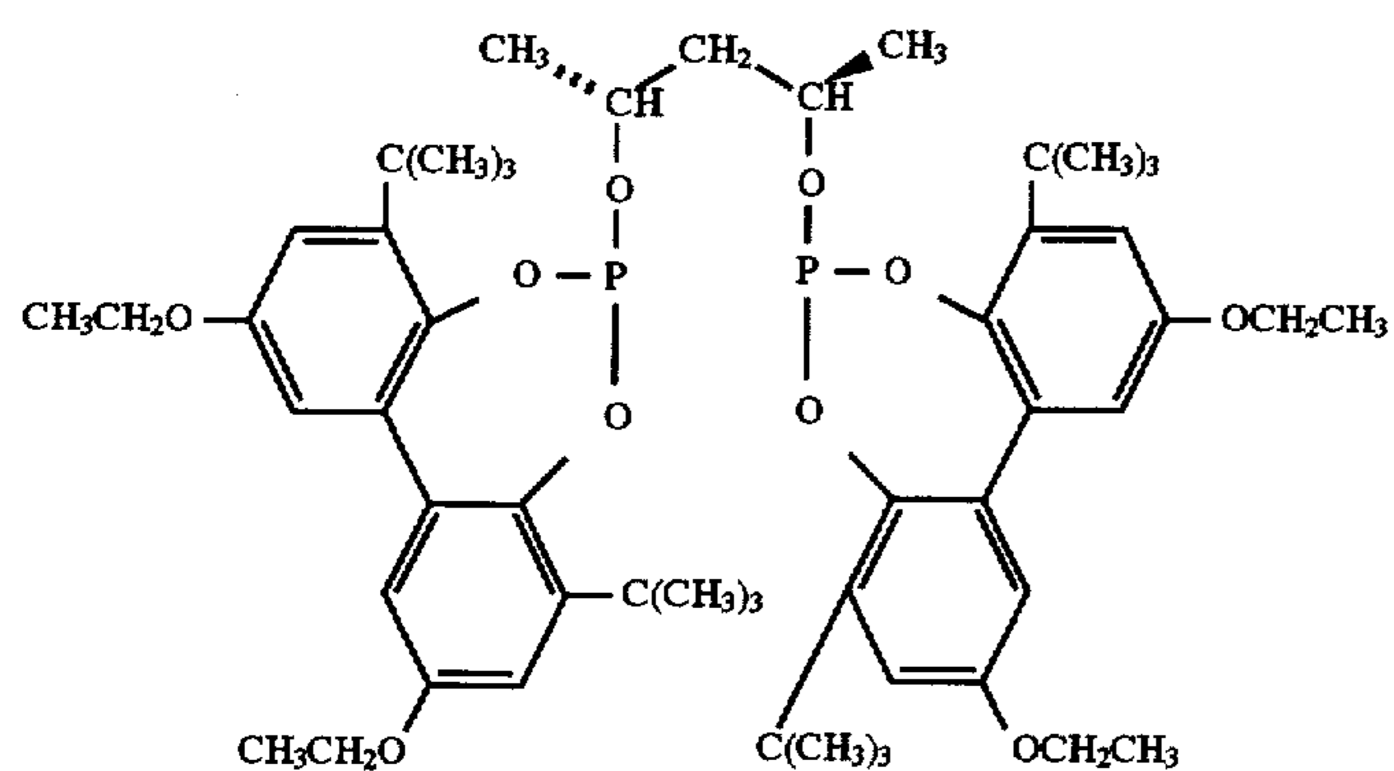
Ligand K
