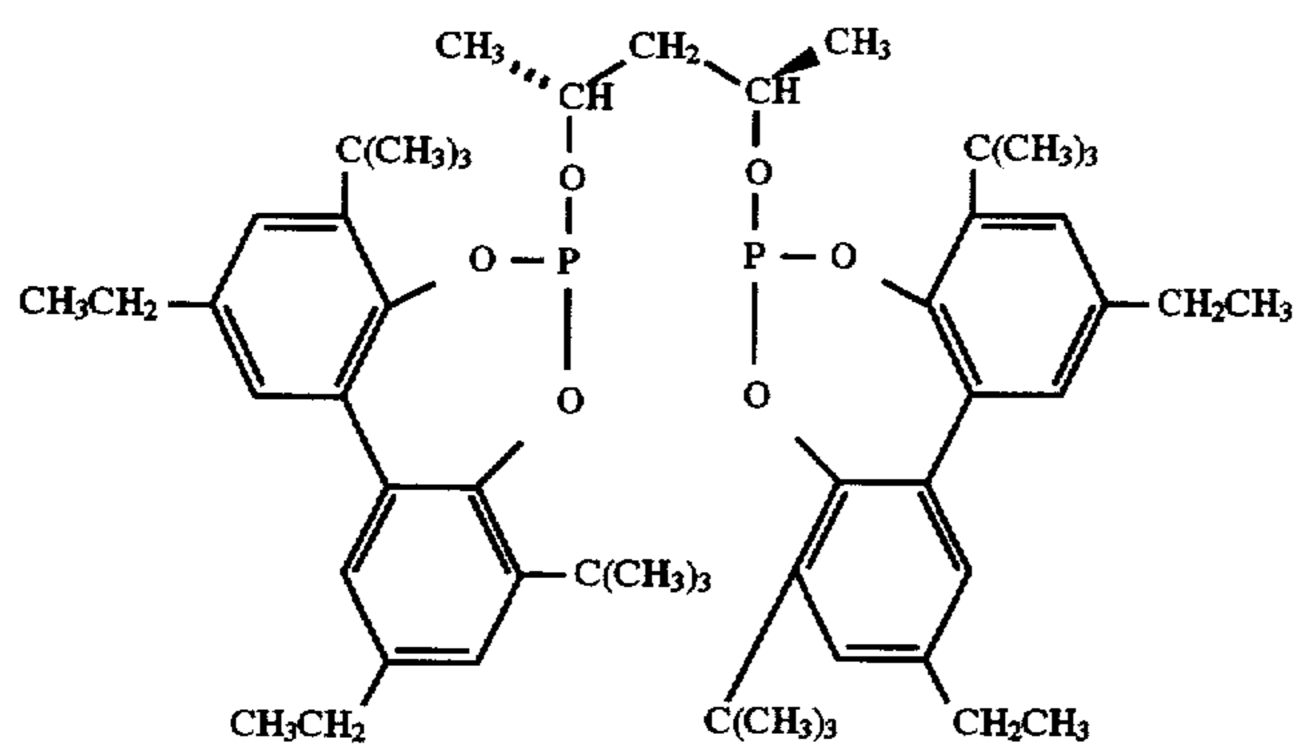
Ligand L
