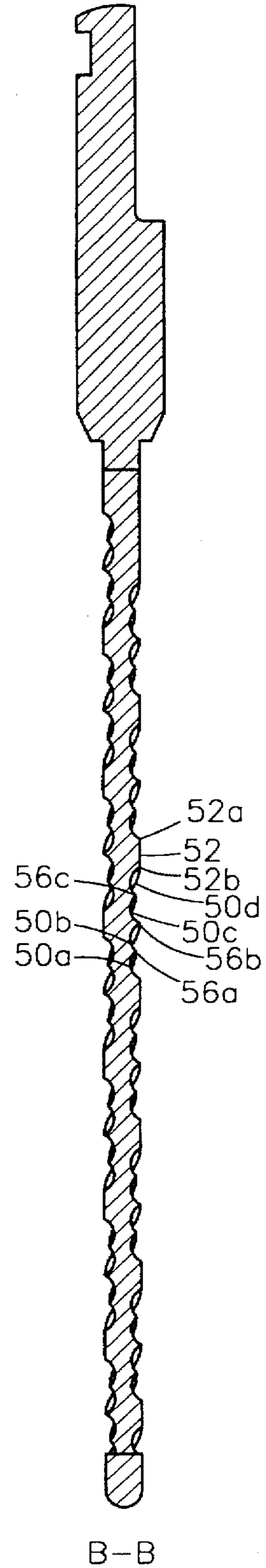
B-B Fig. 12
