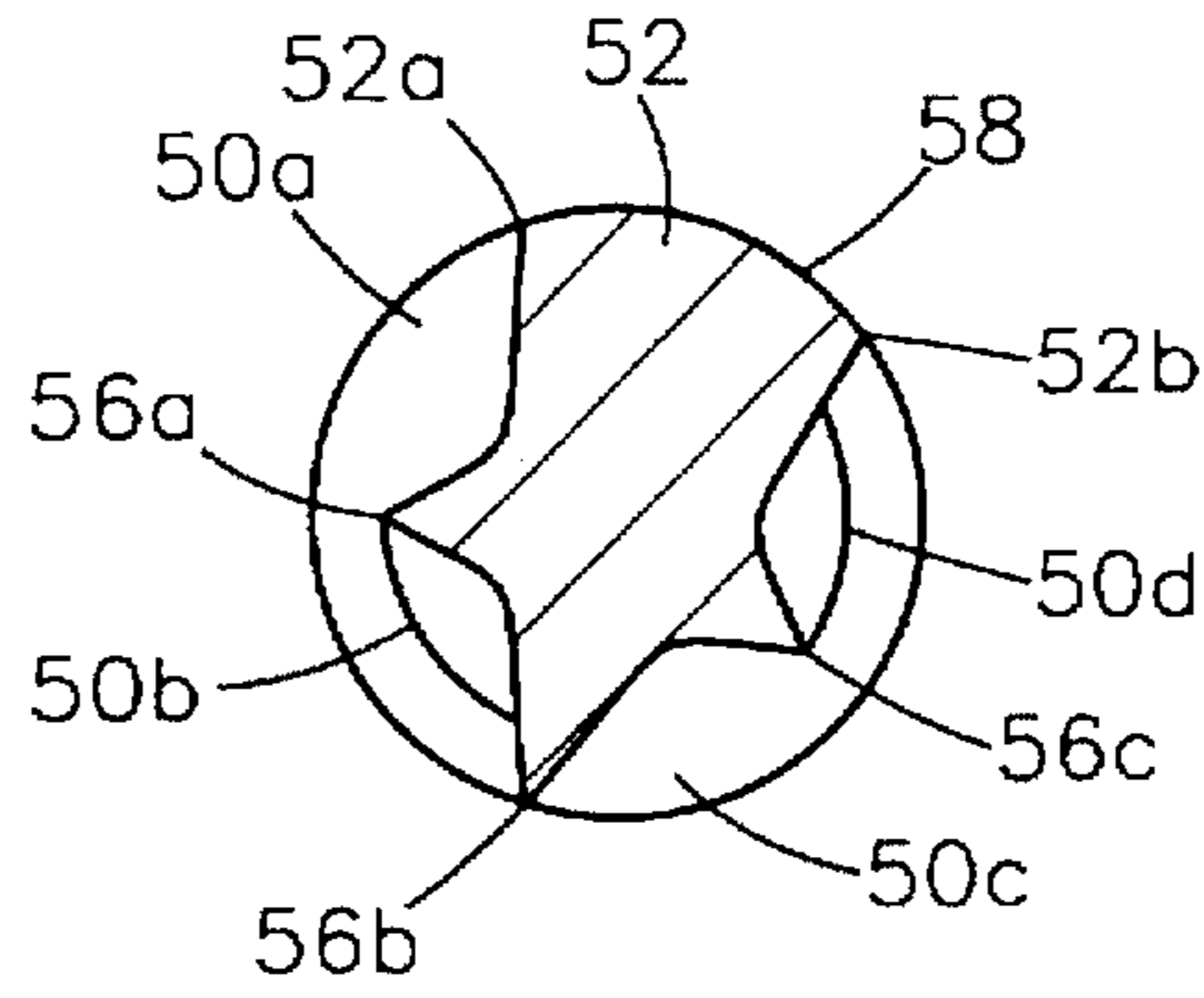
A-A Fig. 11
