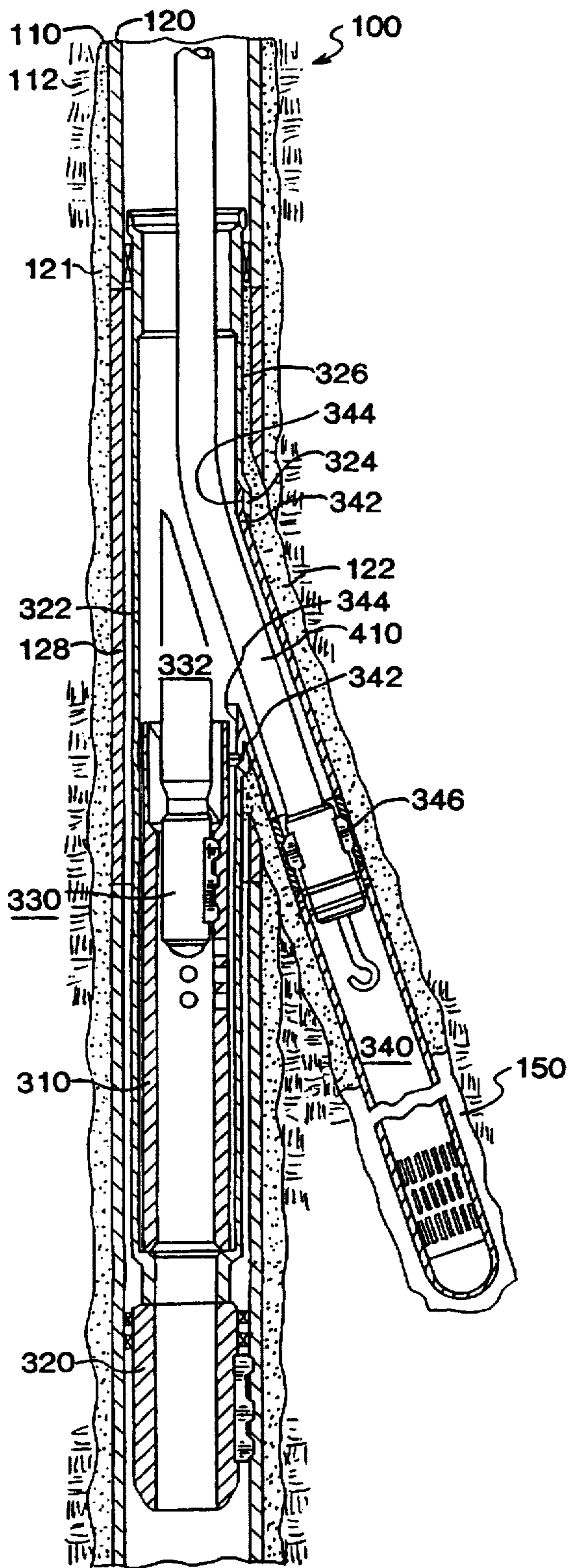
FIG. 4
