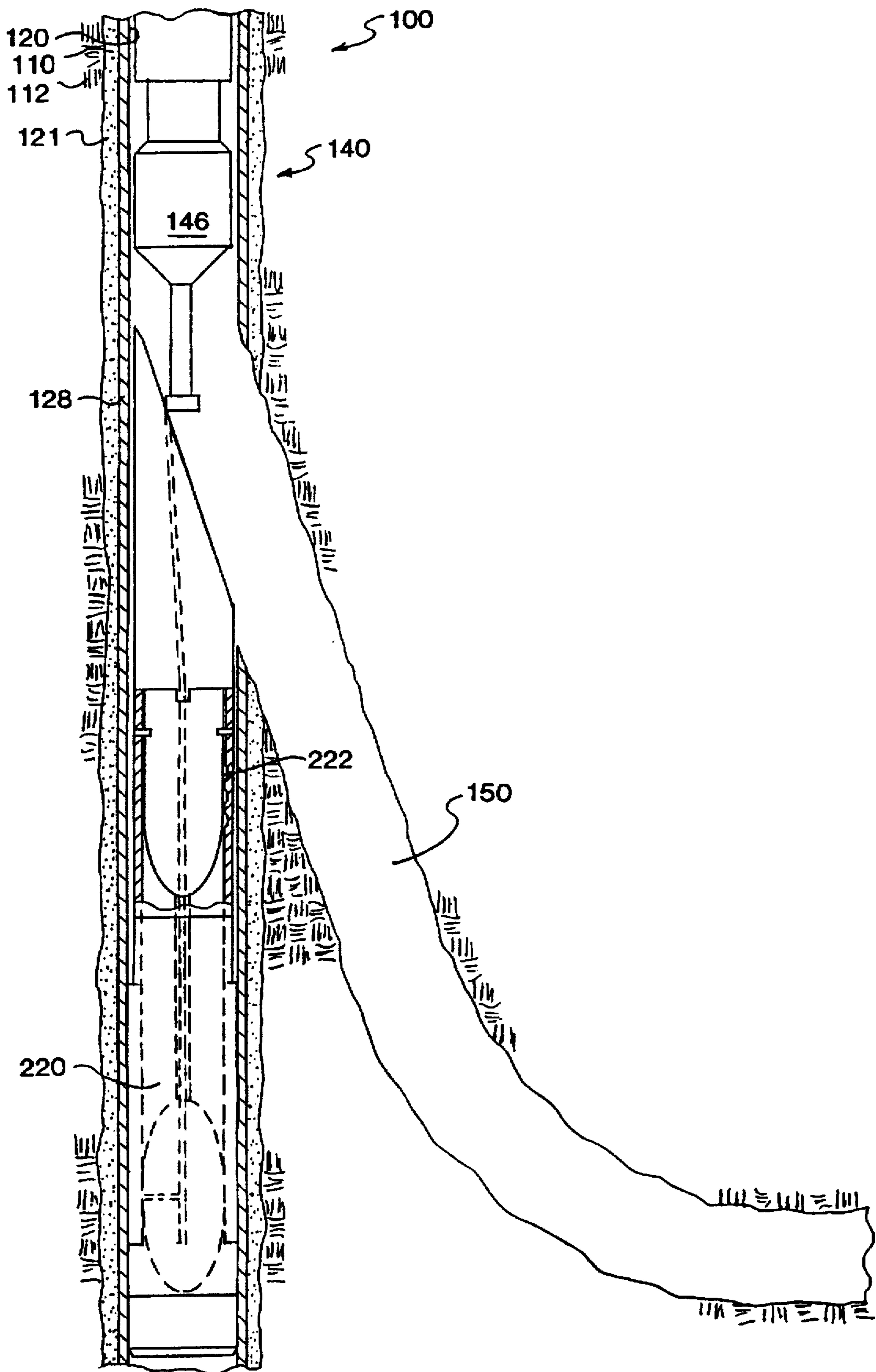
FIG. 2
