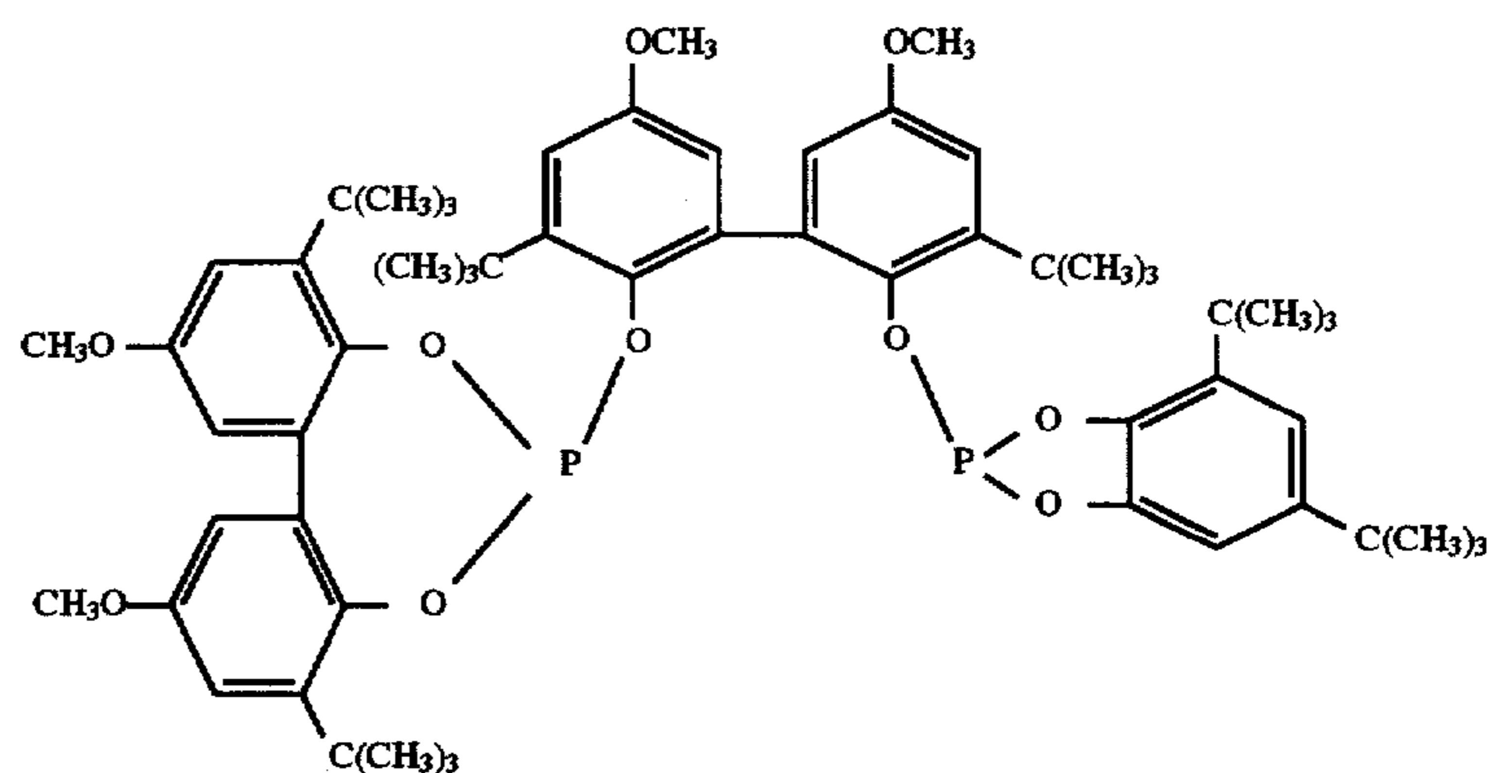
Ligand L
