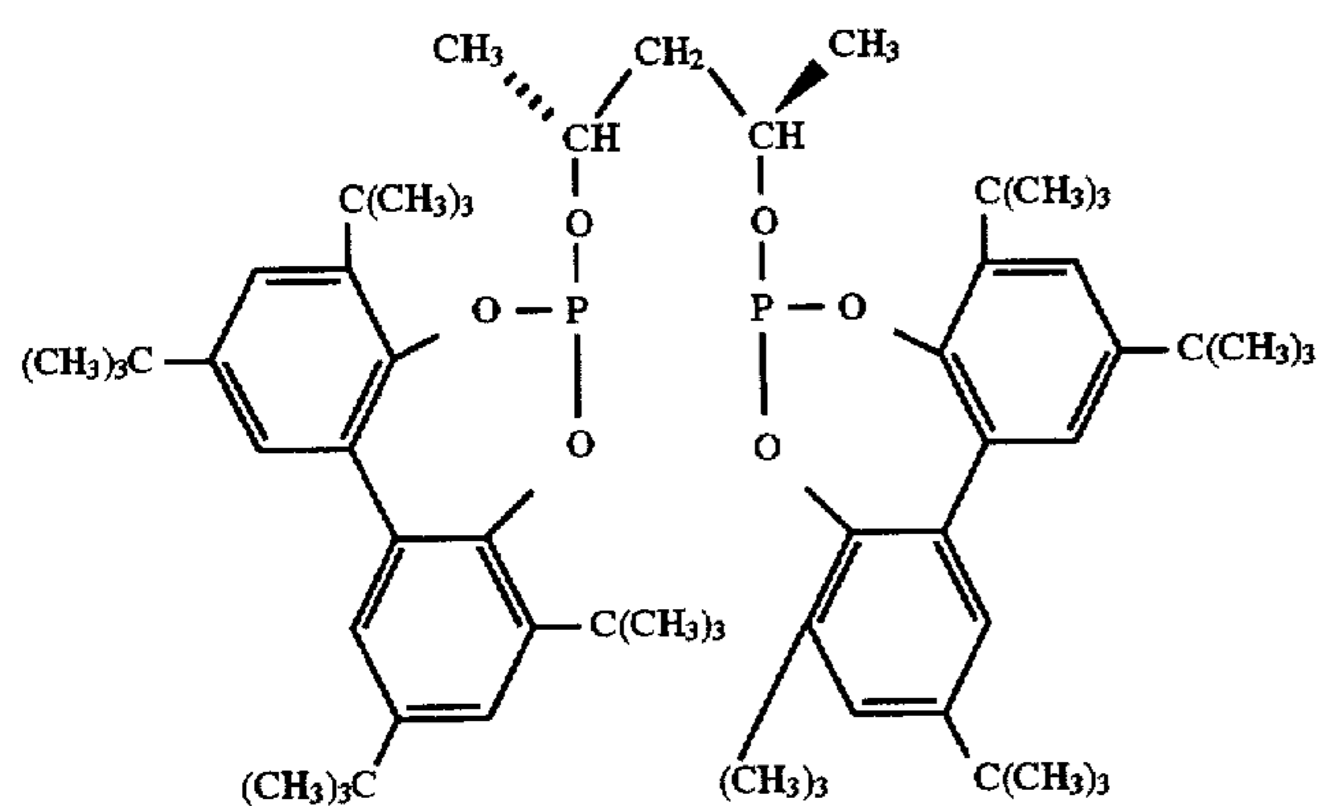
Ligand F
