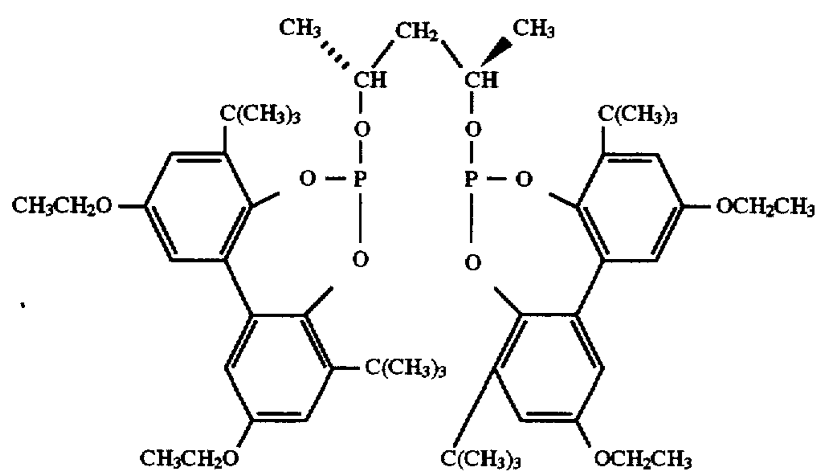
Ligand I
