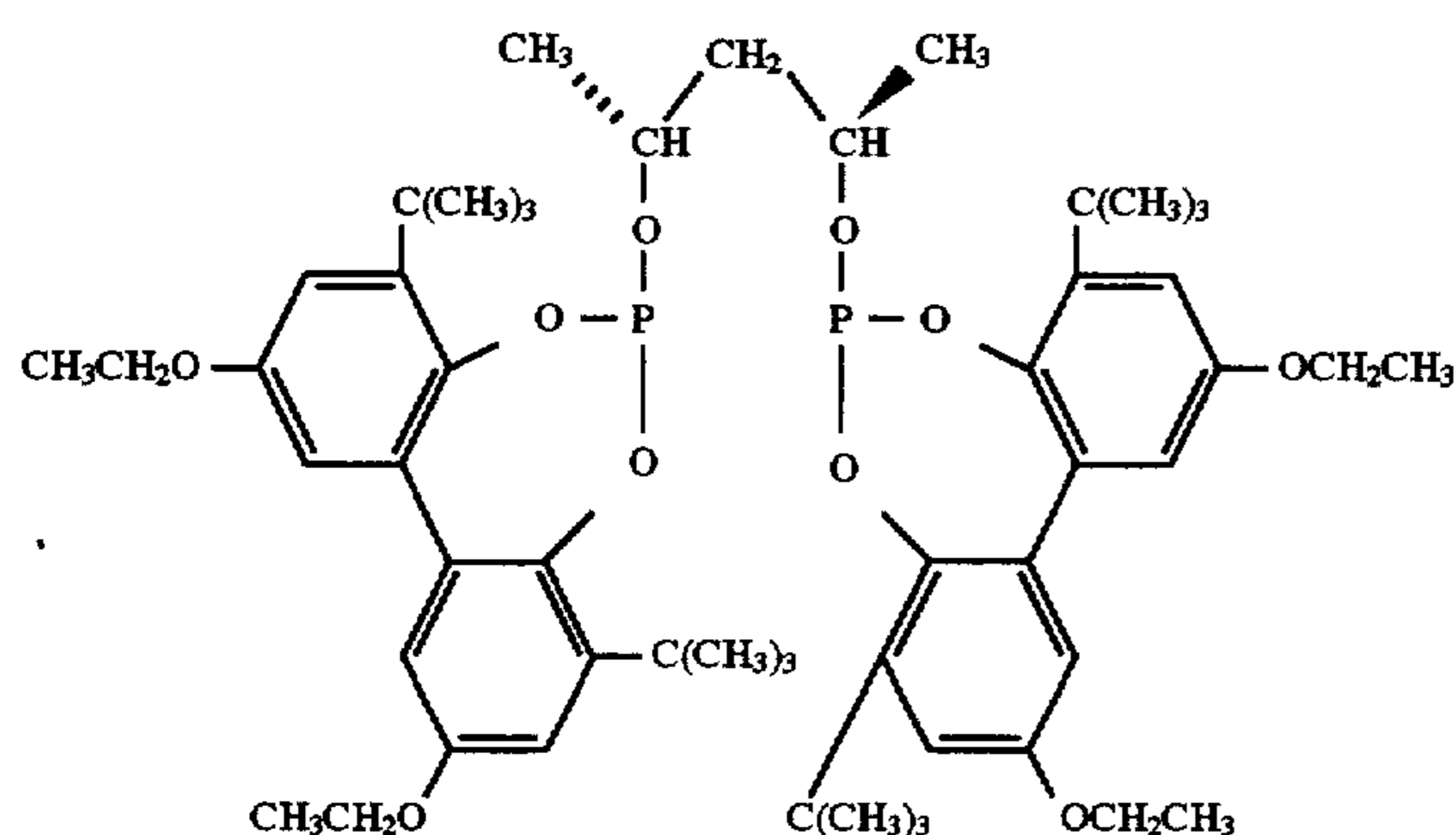
Ligand I
