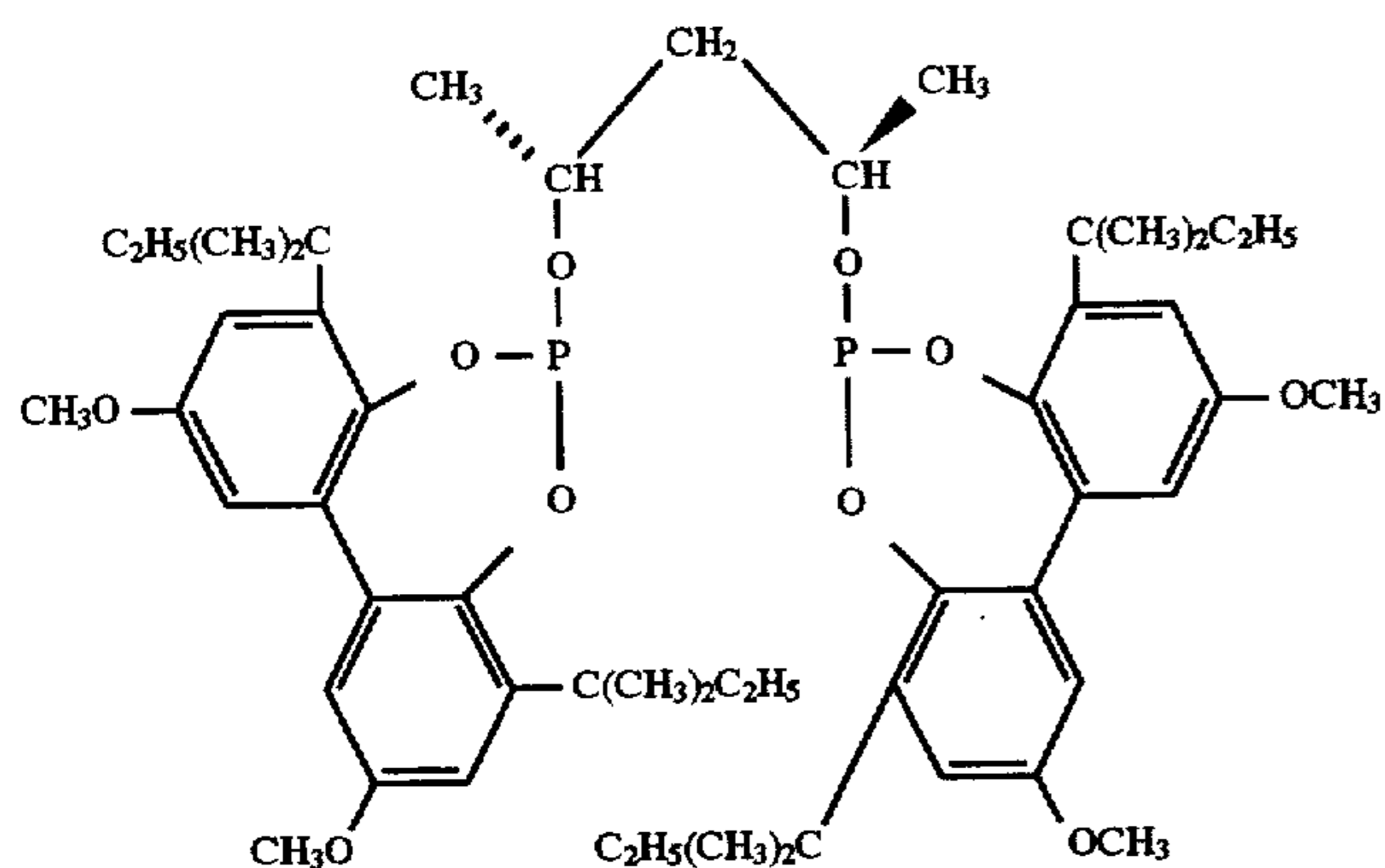
Ligand G
