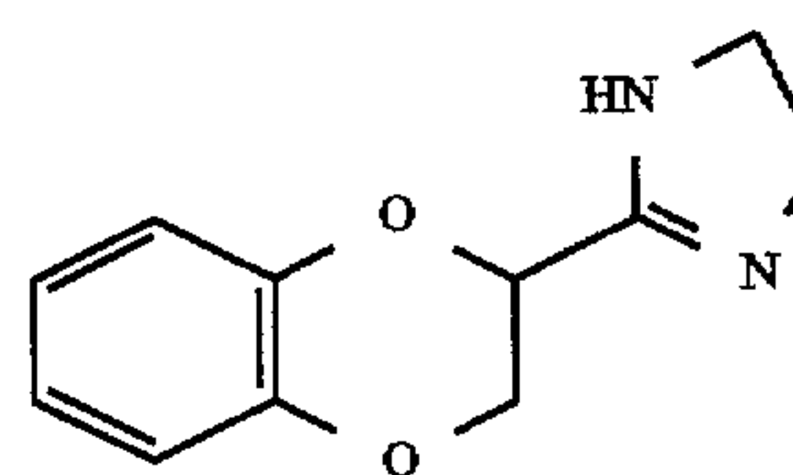
Idazoxan
