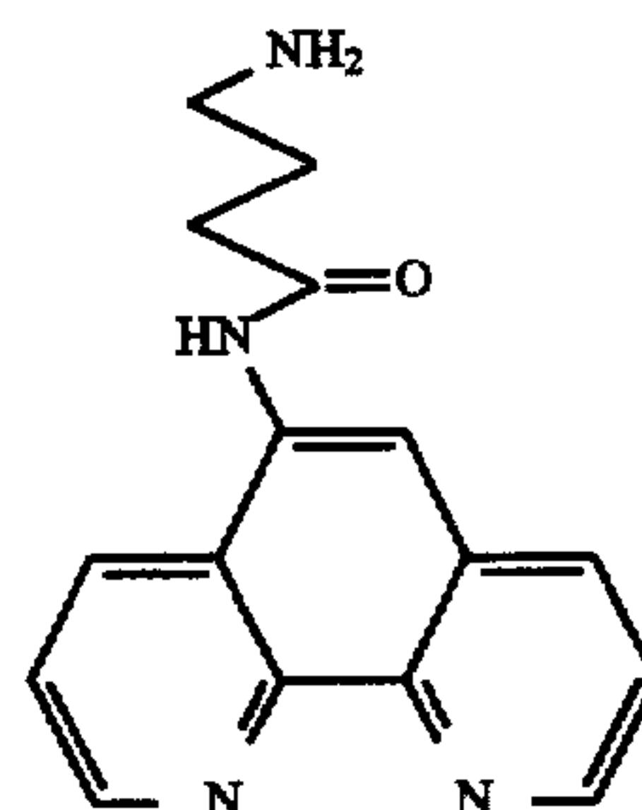
5-(3-aminopropionamido)-1,10-phenanthroline
