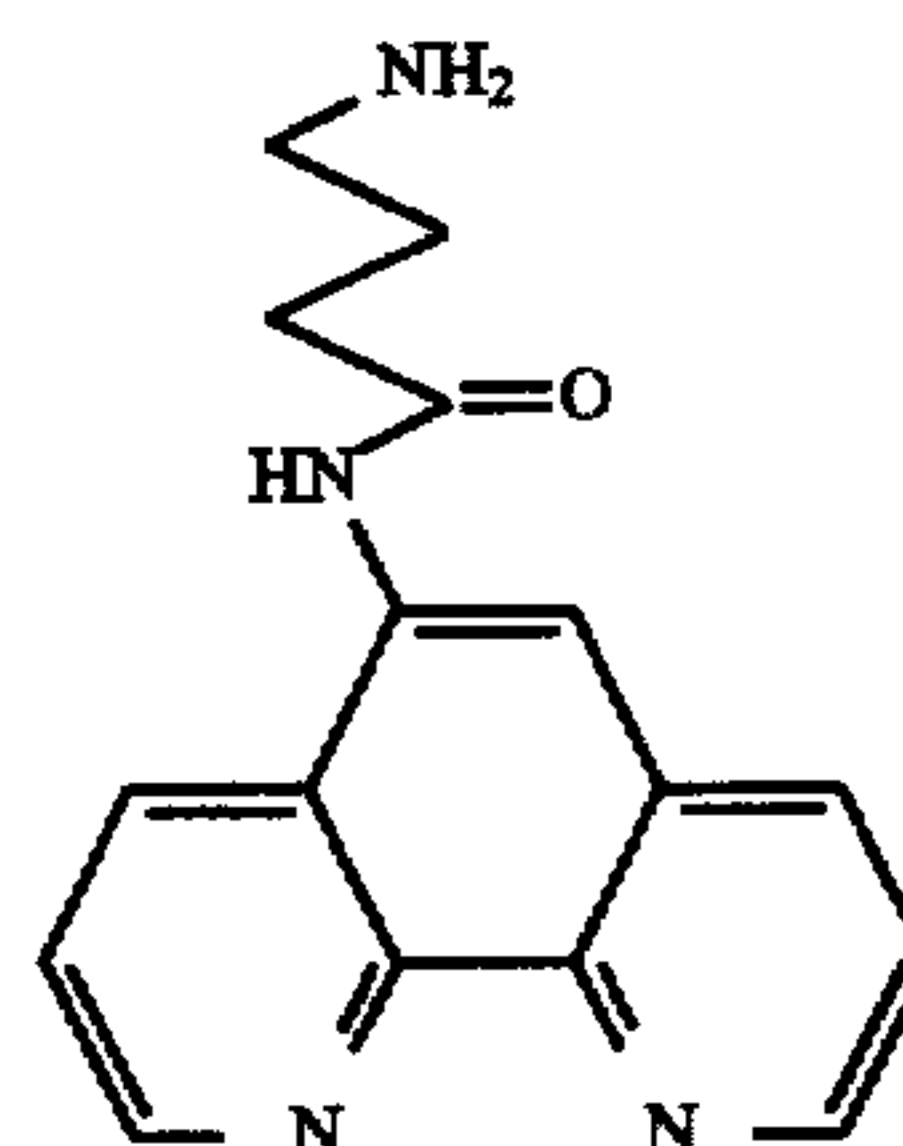
5-(3-aminopropionamido)-1,10-phenanthroline
