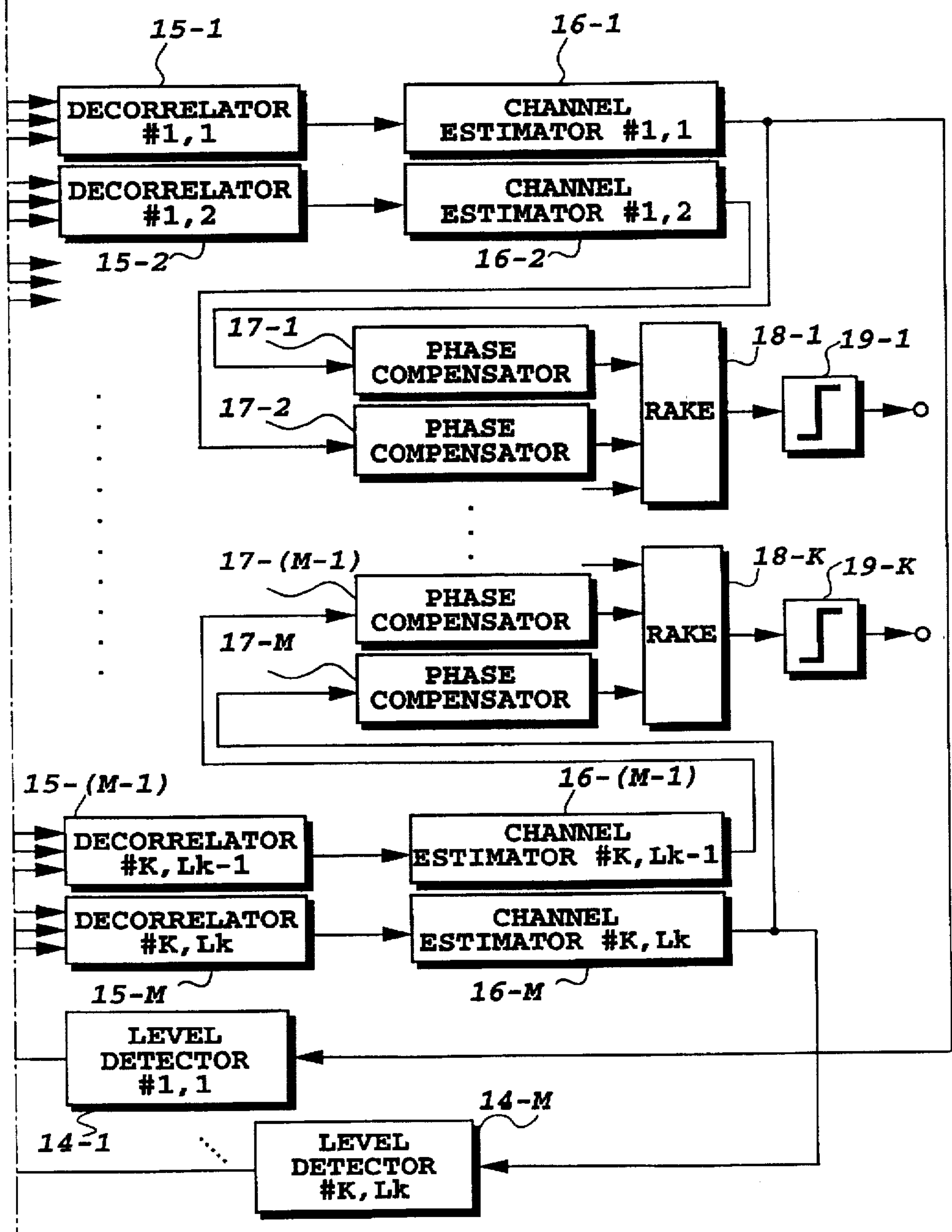
FIG. 14B
