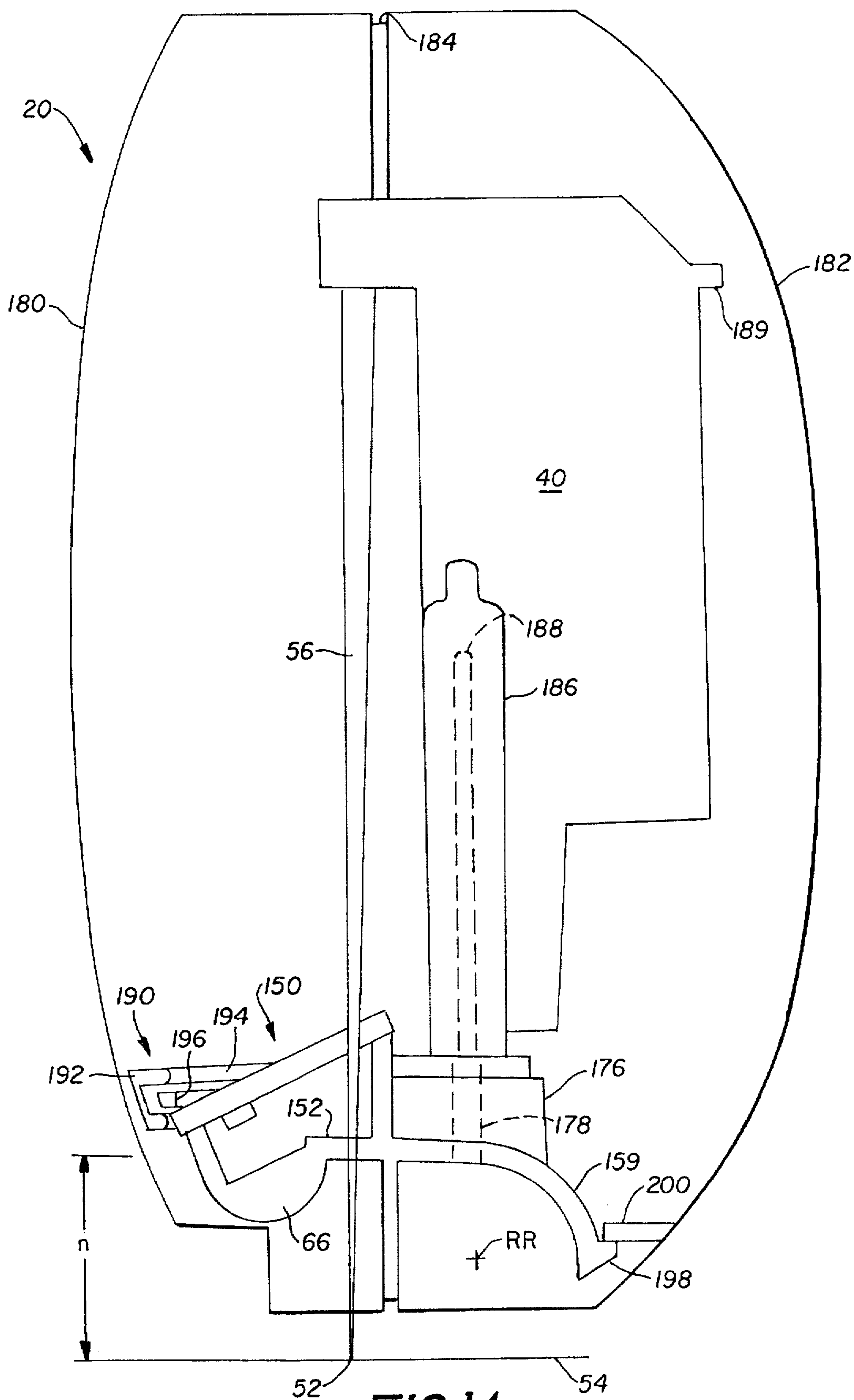
FIG. 14
