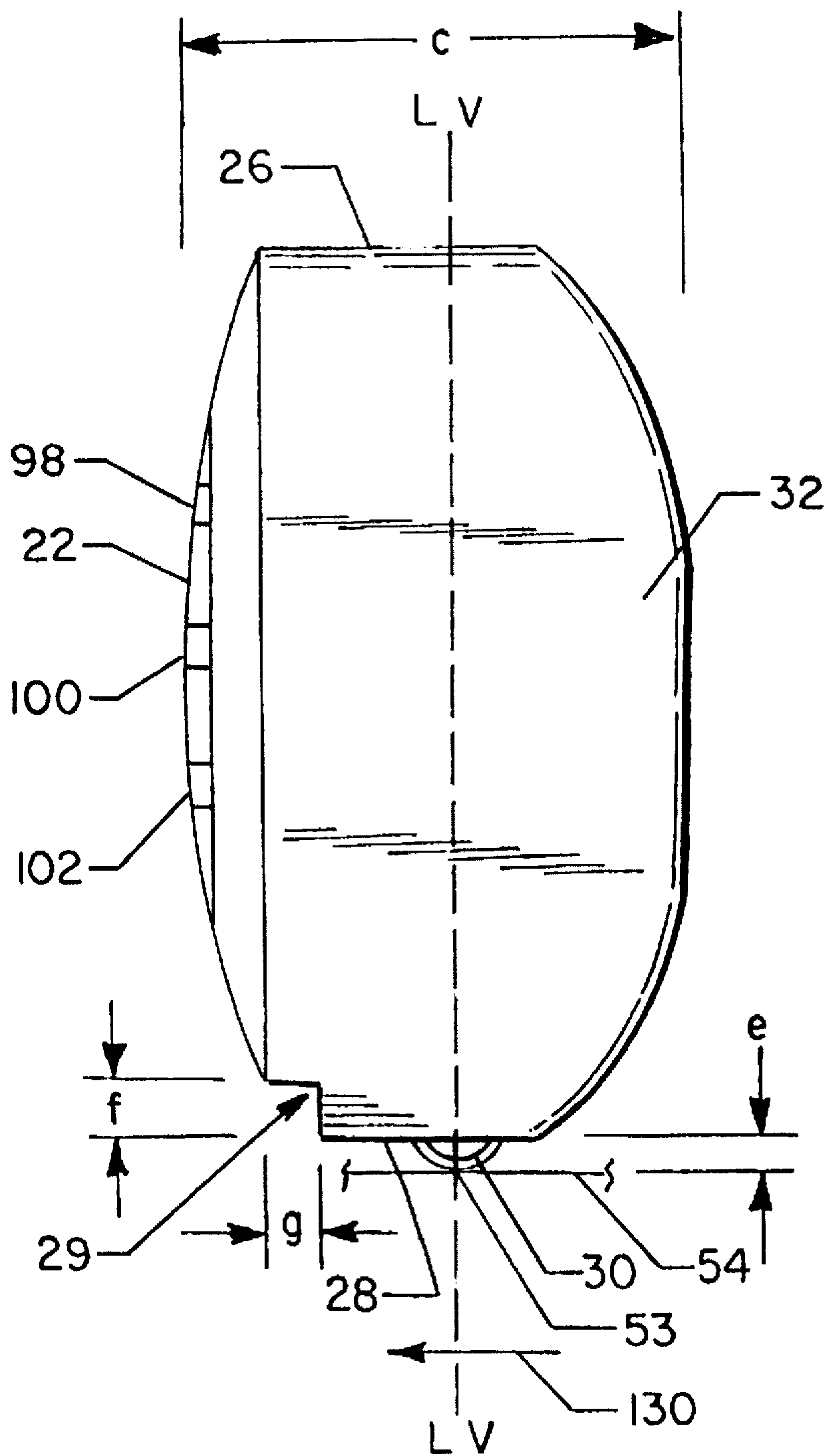
FIG.3
