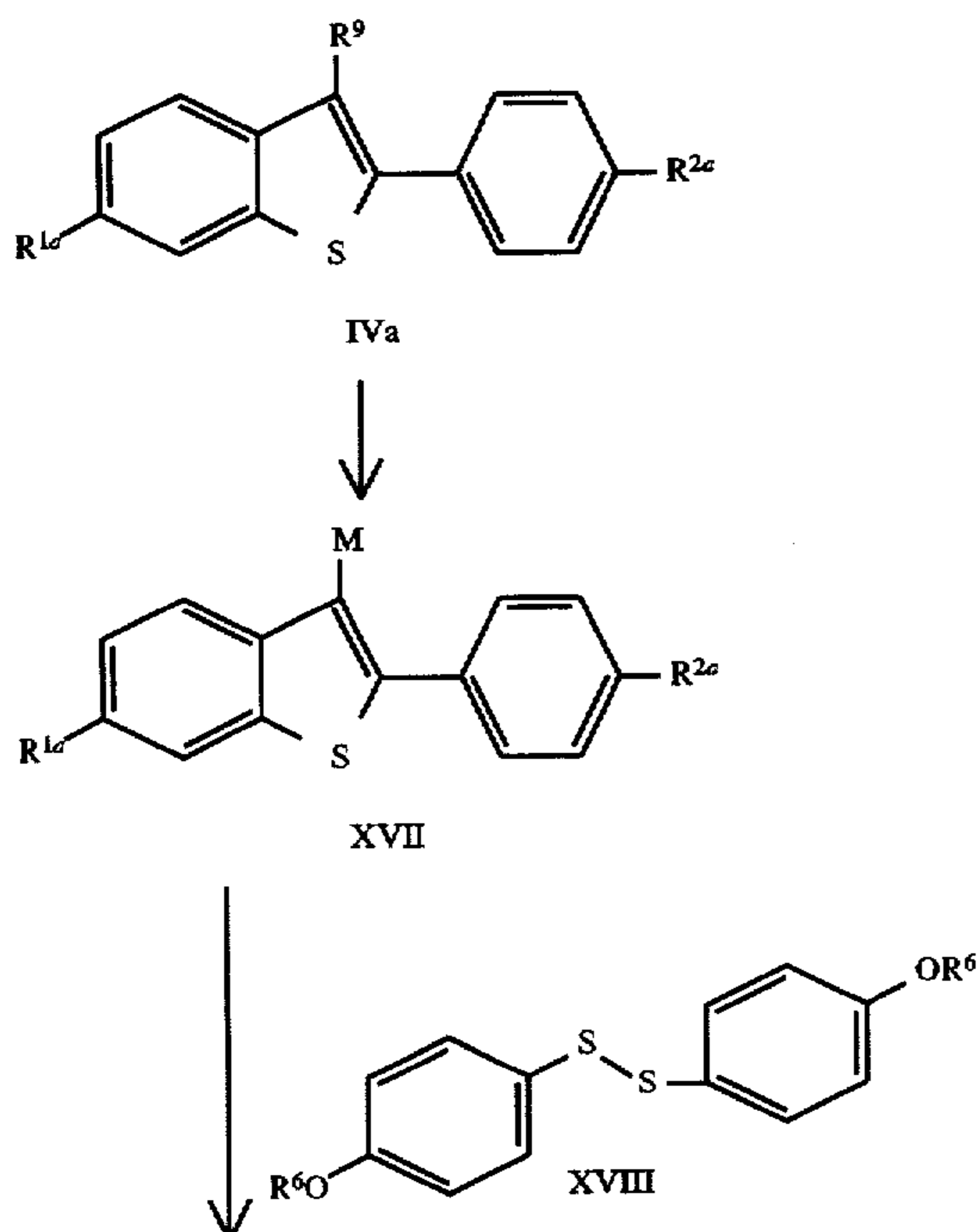
Scheme VI
