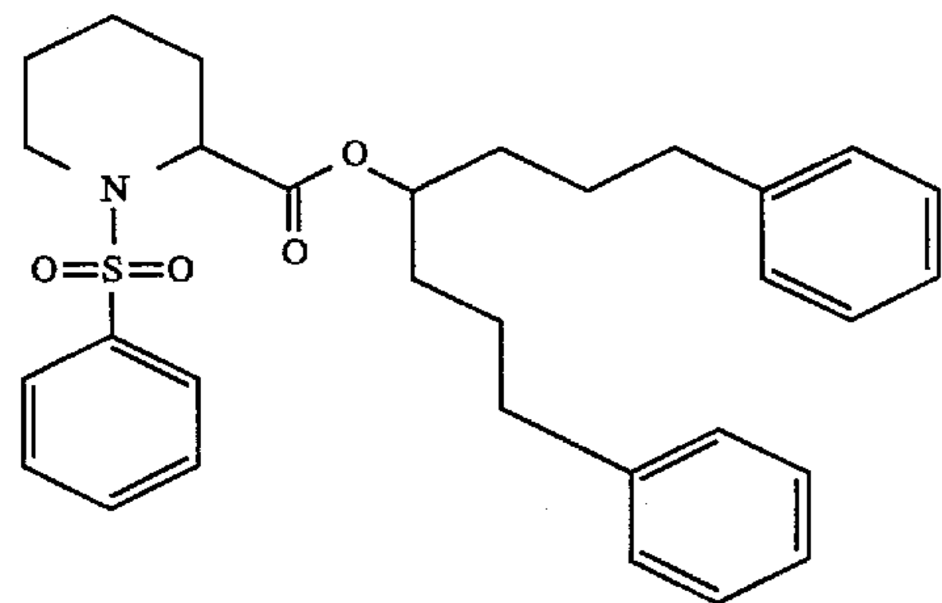
1,7-diphenyl-4-heptyl-N-(para-toluenesulfonyl)pipecolate
