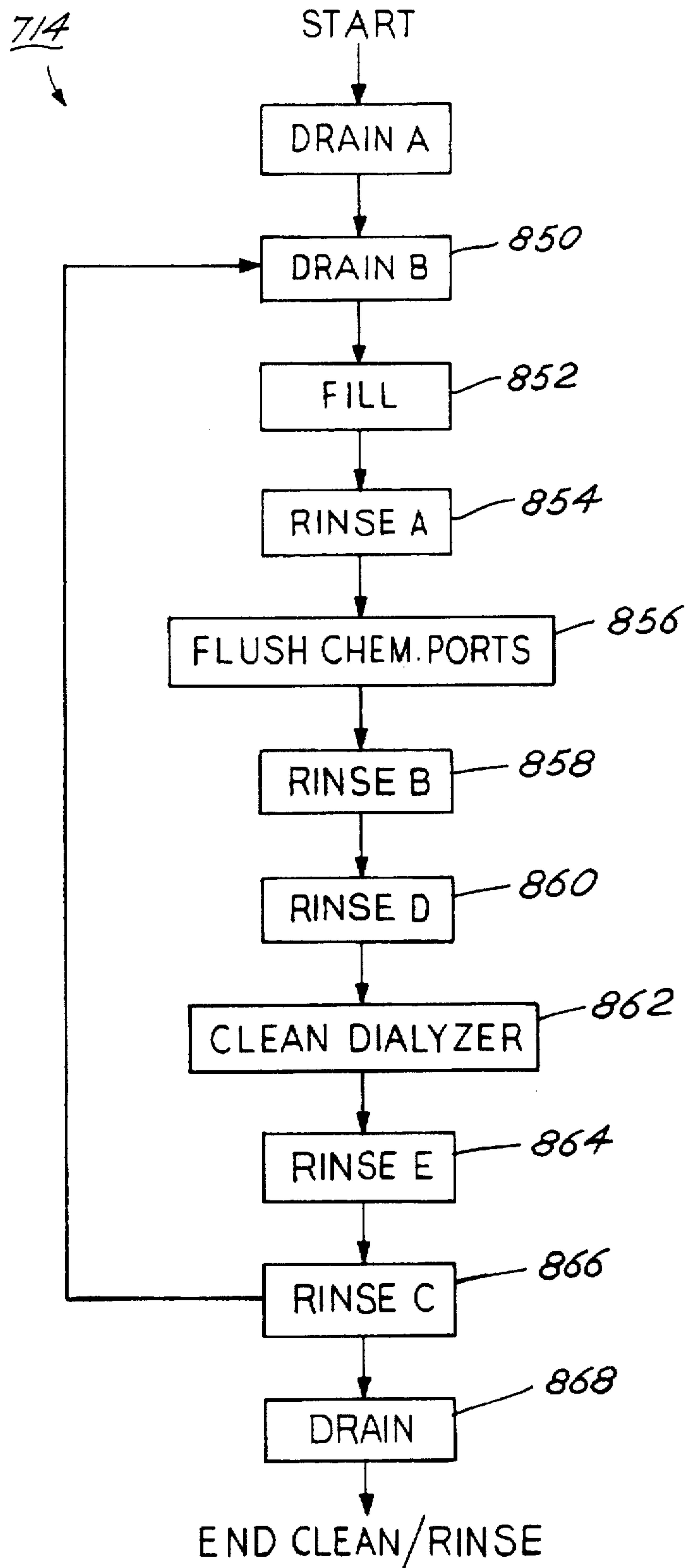
FIG. 23 CLEAN/RINSE
