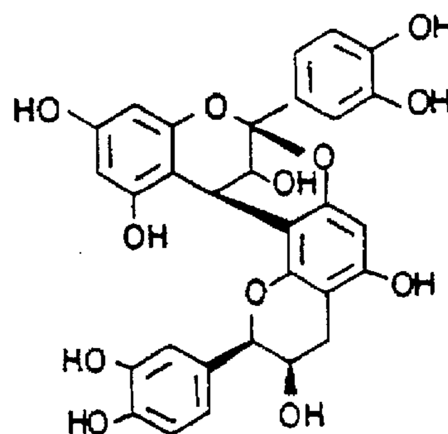
PROCYANIDIN A-2
