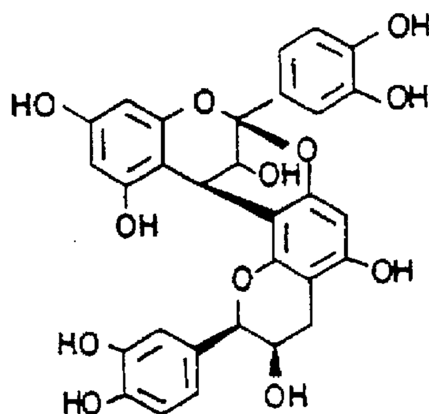
PROCYANIDIN A-2
