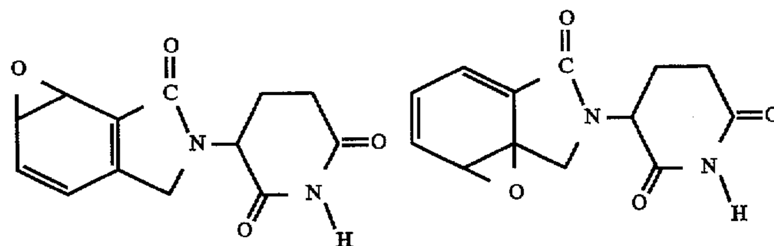
Epoxides of EM 12
