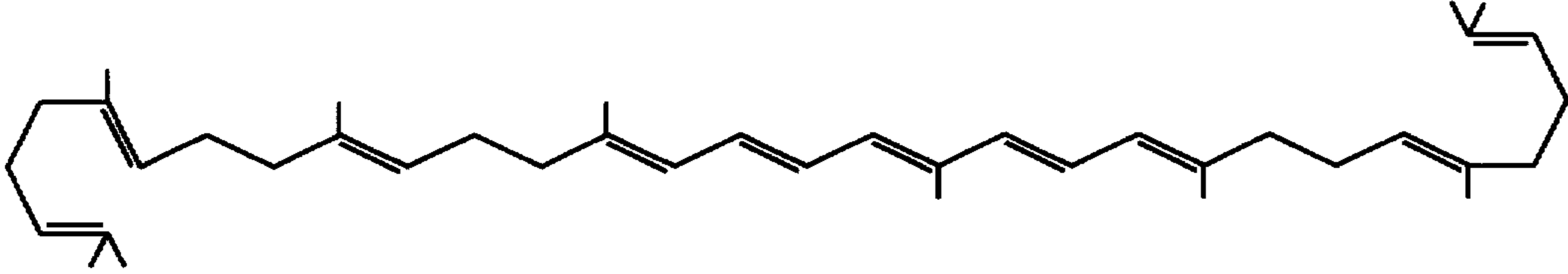
PHYTOFLUENE
