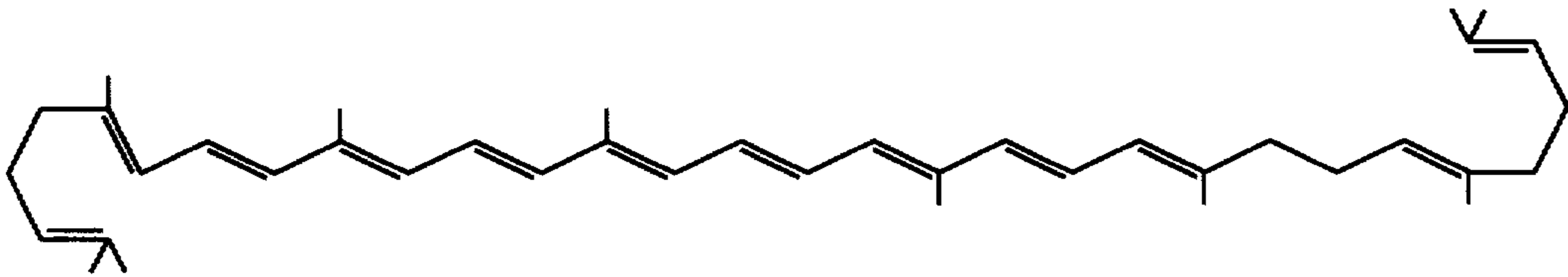
MEUROSPORENE
