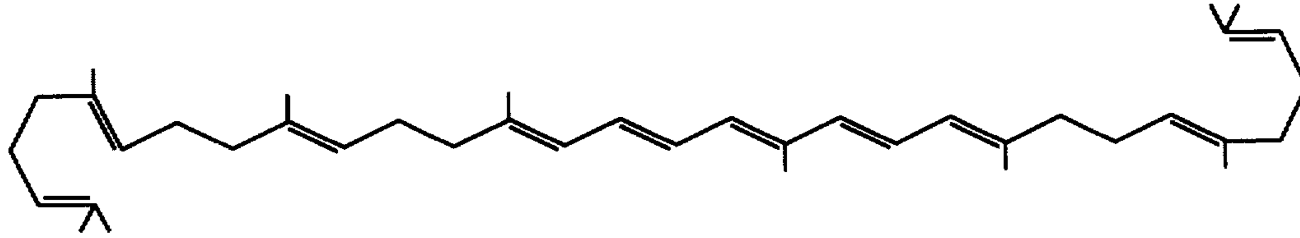
PHYTOFLUENE
