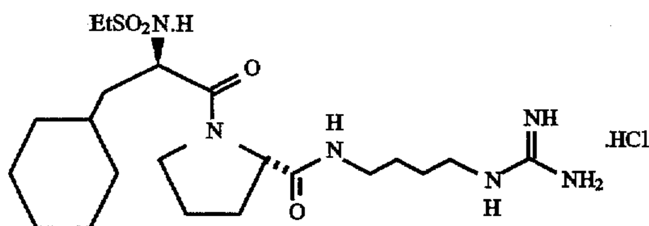
EtSO 2 -D-Cha-Pro-Agm.HCl
