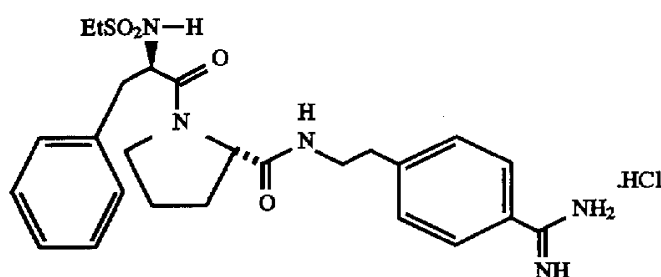
EtSO 2 -D-Phe-Pro-p-NHCH 2 CH 2 -C 6 H 4 C(=NH)NH 2 .HCl
