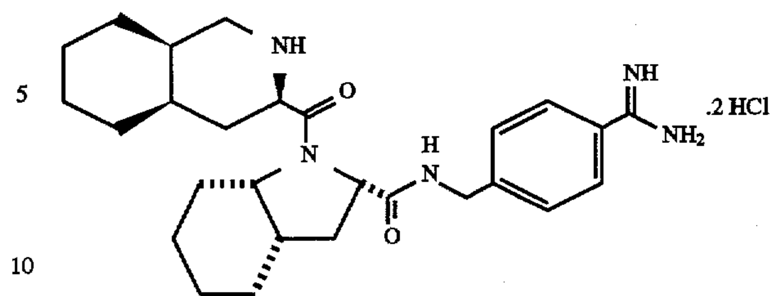
D-3-Piq-cis-Ohi-p-NHCH 2 C 6 H 4 C(NH)NH 2 .2HCl
