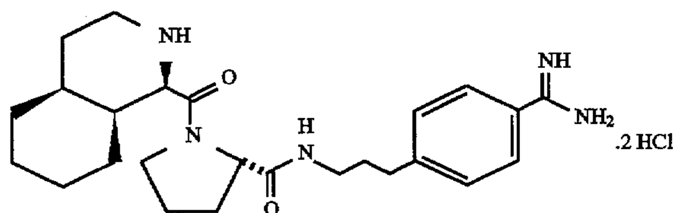
1-Piq-Pro-p-NHCH 2 CH 2 CH 2 -C 6 H 4 C(=NH)NH 2 .2HCl
