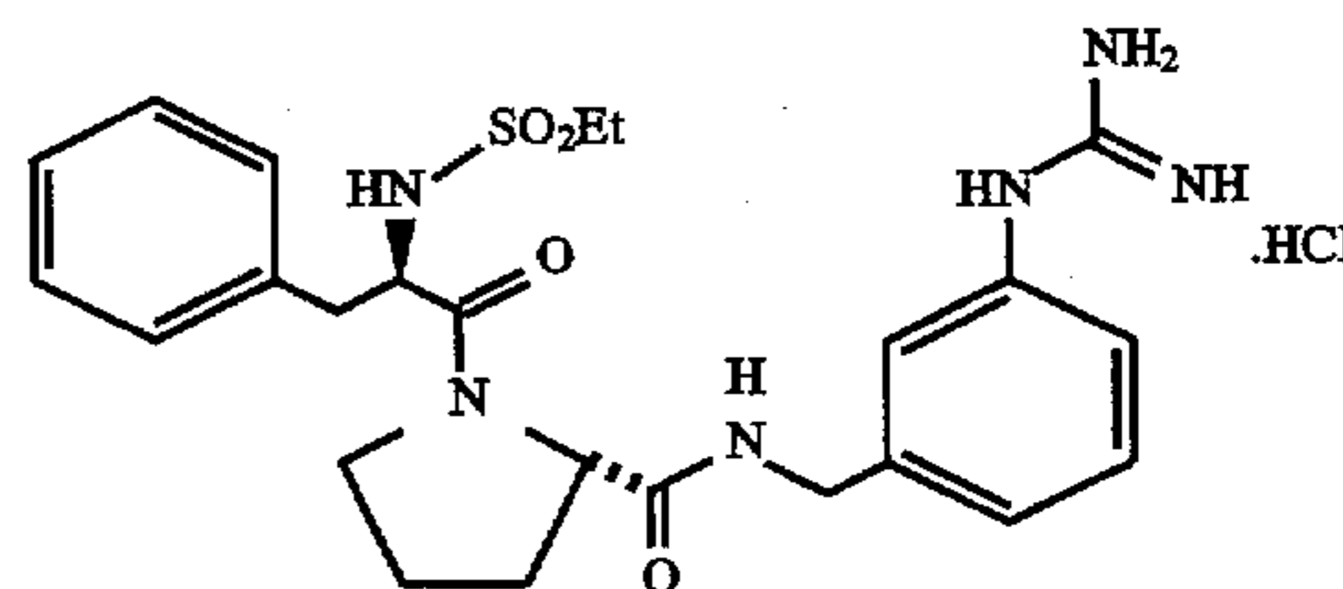
EtSO 2 -D-Phe-Pro-m-NHCH 2 C 6 H 4 NHC(NH)NH 2 ·HCl
