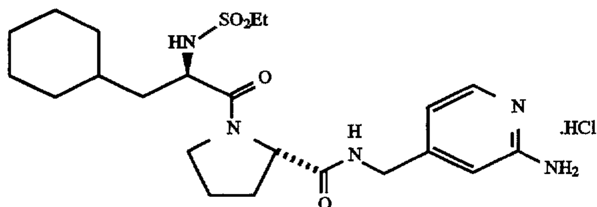
EtSO 2 -D-Cha-Pro-4-NHCH 2 -2-aminopyridine.HCl
