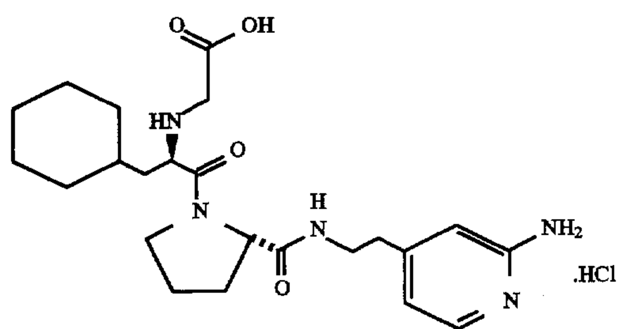
HO 2 CCH 2 -D-Cha-Pro-4-NHCH 2 CH 2 -2-aminopyridine.HCl
