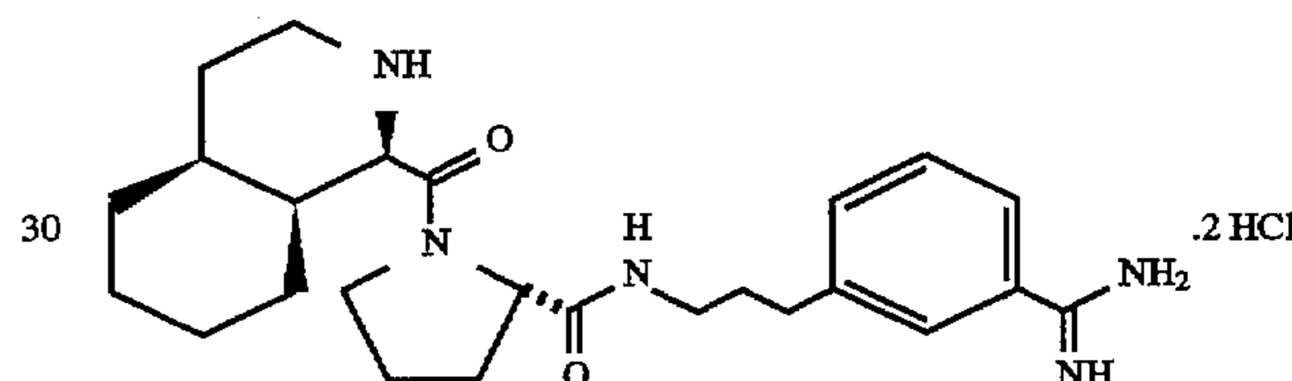
1-Piq-Pro-m-NHCH 2 CH 2 CH 2 -C 6 H 4 C(=NH)NH 2 .2HCl
