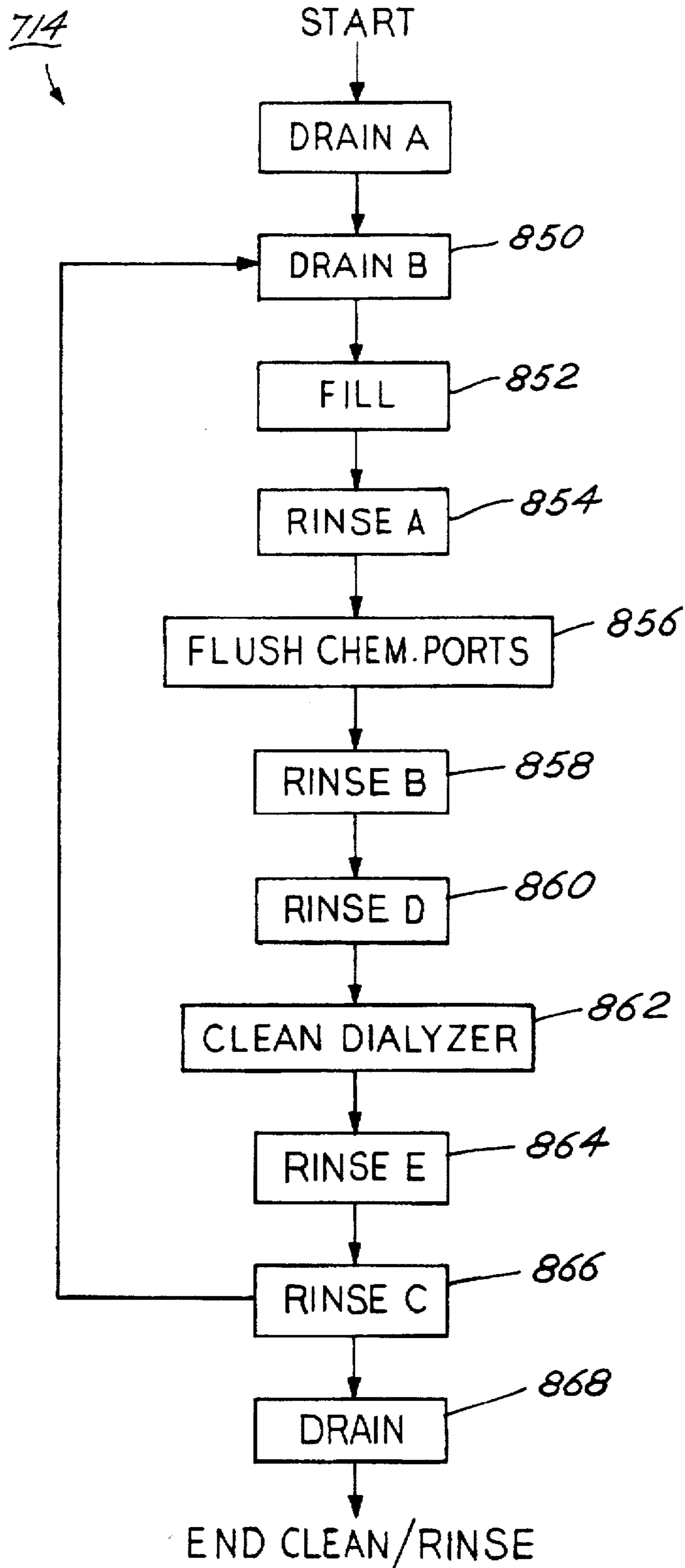
FIG. 23 CLEAN/RINSE
