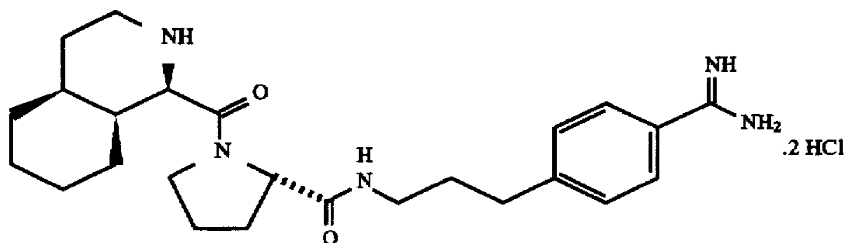
1-Piq-Pro-p-NHCH 2 CH 2 CH 2 -C 6 H 4 C(=NH)NH 2 .2HCl
