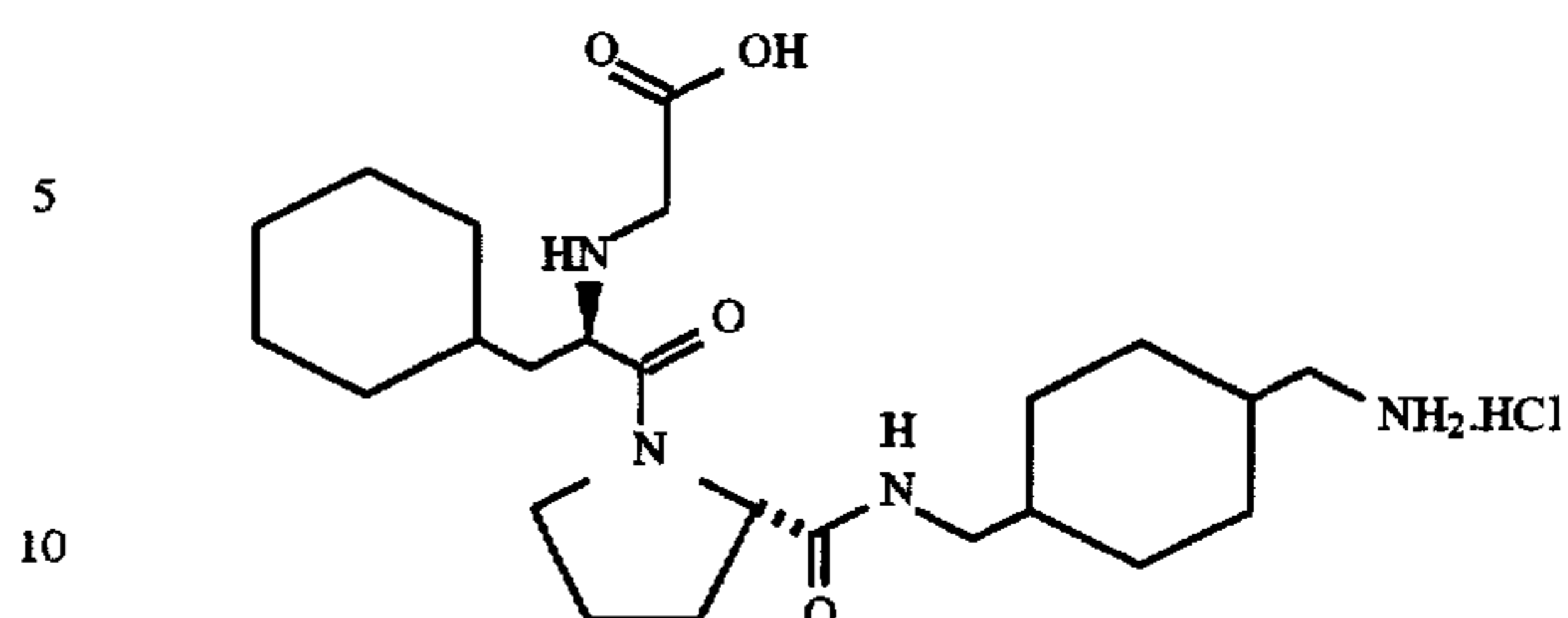
HO 2 CCH 2 -D-Cha-Pro-4-NHCH 2 -C 6 H 10 CH 2 NH 2 .HCl
