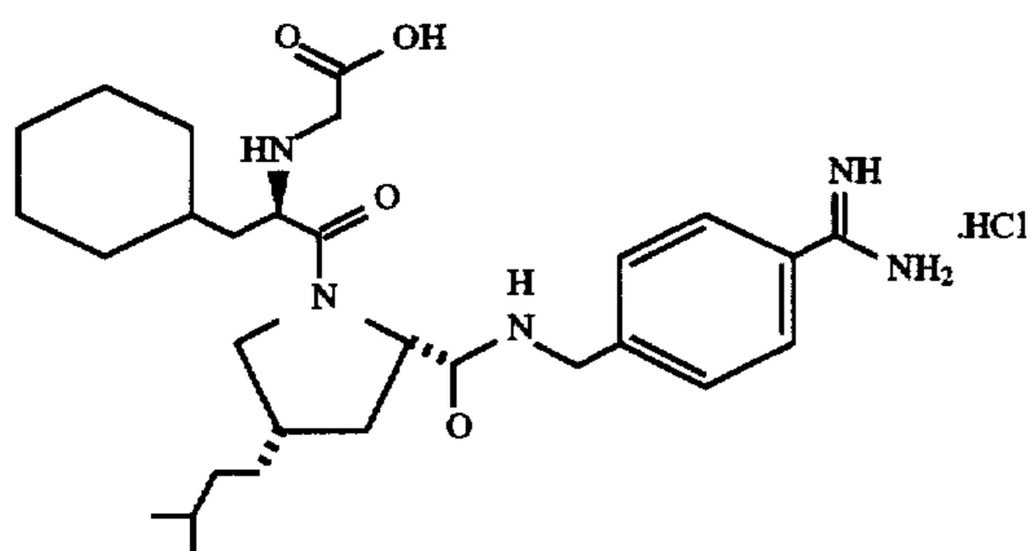
HOOCCH 2 -D-Phe-Pro(4-cis-isoamyl)-p-NHCH 2 C 6 H 4 C(NH)NH 2 .HCl
