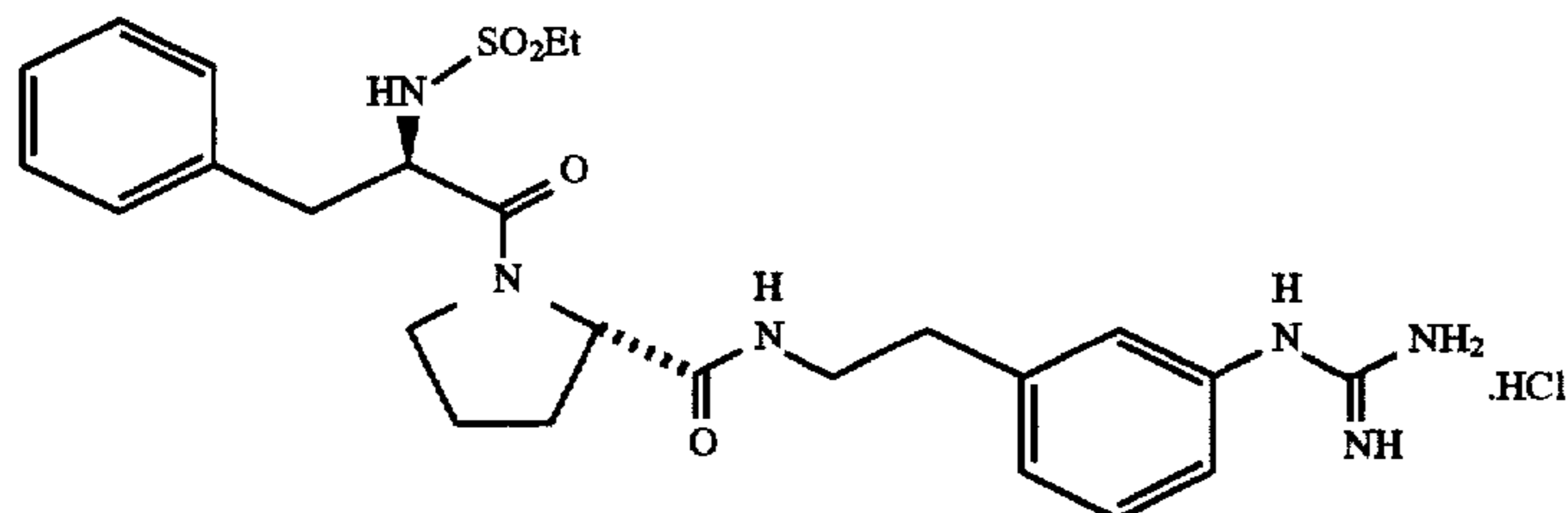
EtSO 2 -D-Phe-Pro-m-NHCH 2 CH 2 C 6 H 4 NHC(NH)NH 2 .HCl
