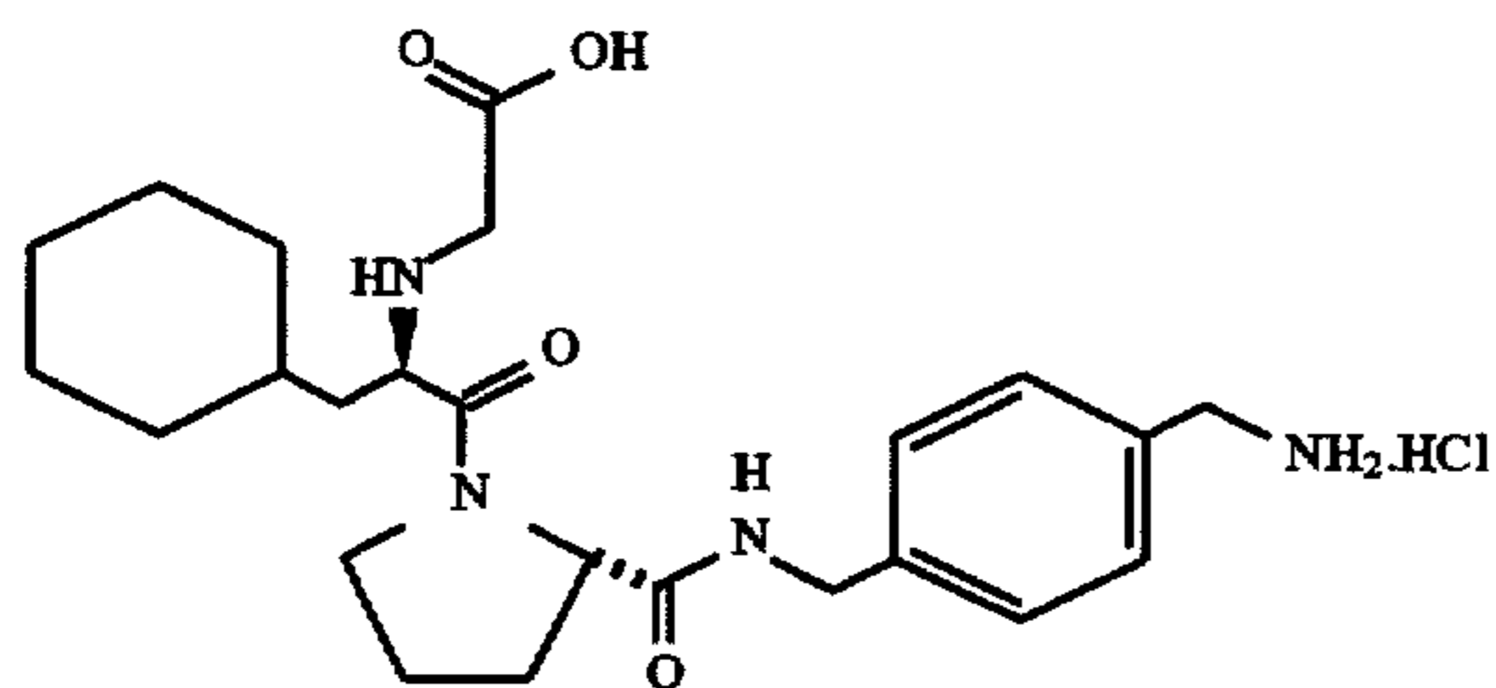
HO 2 CCH 2 -D-Cha-Pro-4-NHCH 2 -C 6 H 4 CH 2 NH 2 .HCl
