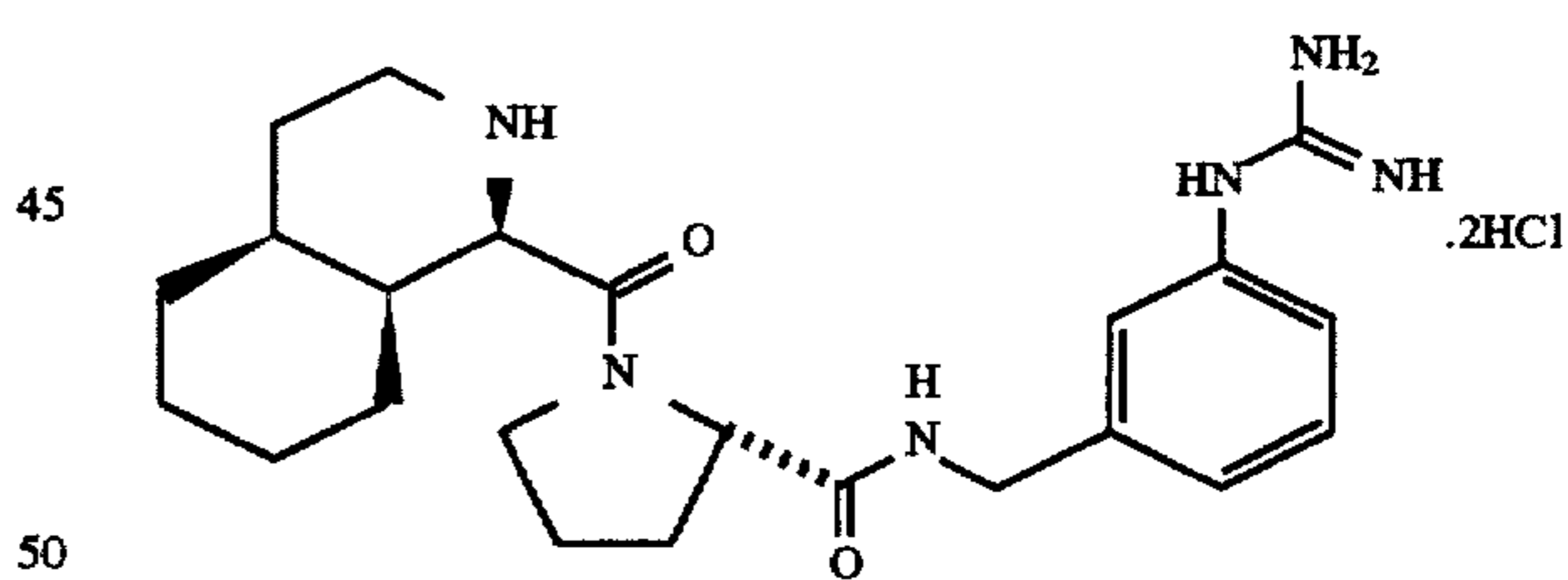
D-1-Piq-Pro-m-NHCH 2 C 6 H 4 NHC(NH)NH 2 .2HCl
