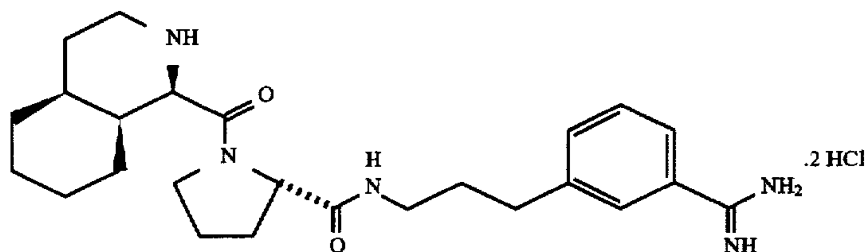
1-Piq-Pro-m-NHCH 2 CH 2 CH 2 -C 6 H 4 C(=NH)NH 2 .2HCl
