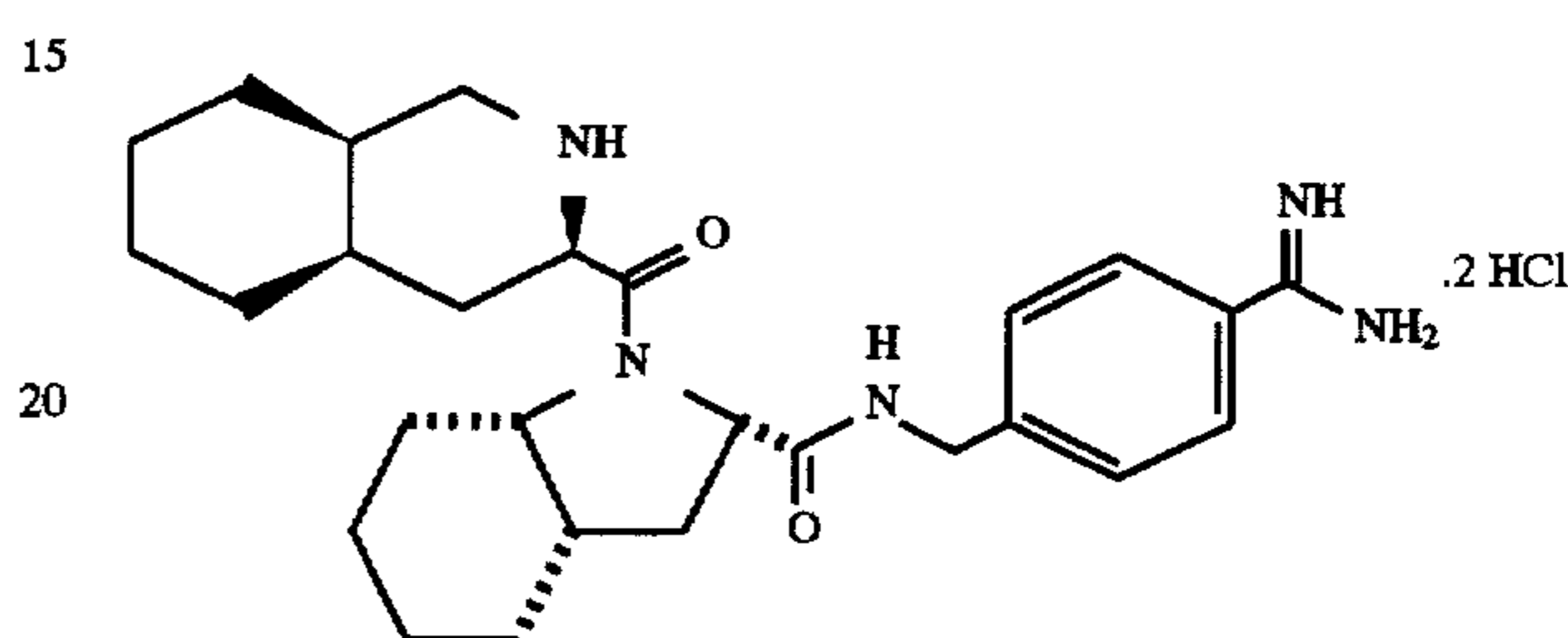
D-3-Piq-cis-Ohi-p-NHCH 2 C 6 H 4 C(NH)NH 2 .2HCl
