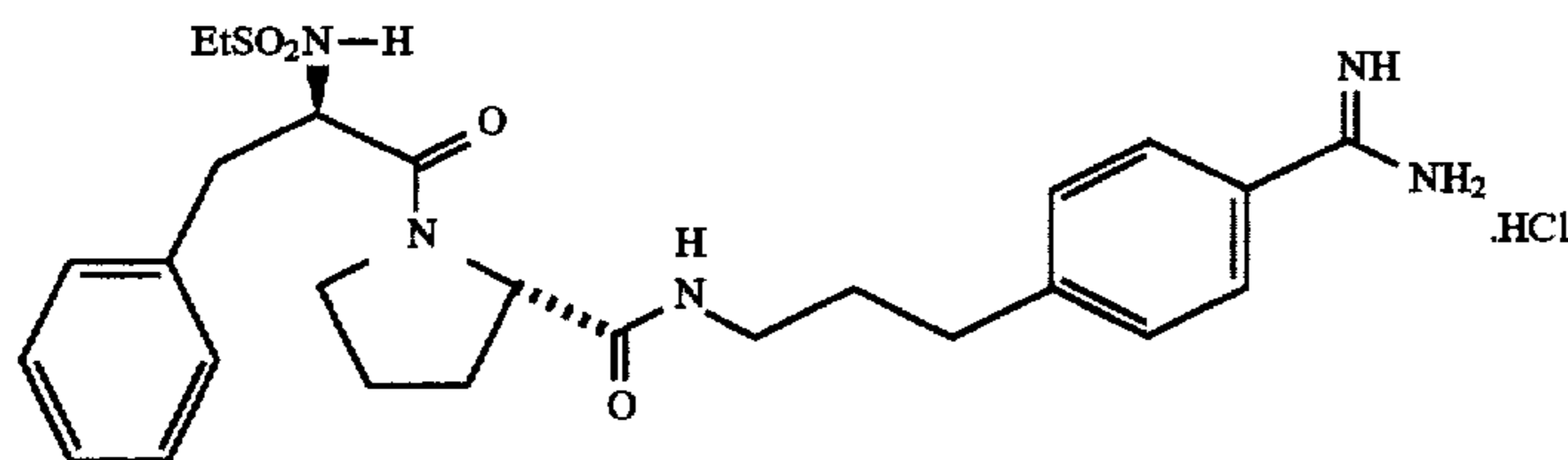
EtSO 2 -D-Phe-Pro-p-NHCH 2 CH 2 CH 2 -C 6 H 4 C(=NH)NH 2 .HCl
