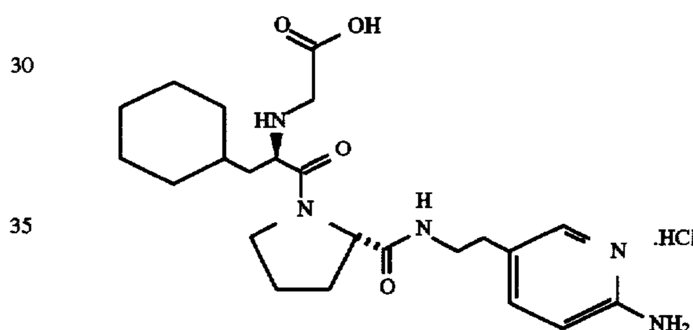
HO 2 CCH 2 -D-Cha-Pro-5-NHCH 2 -2-aminopyridine.HCl
