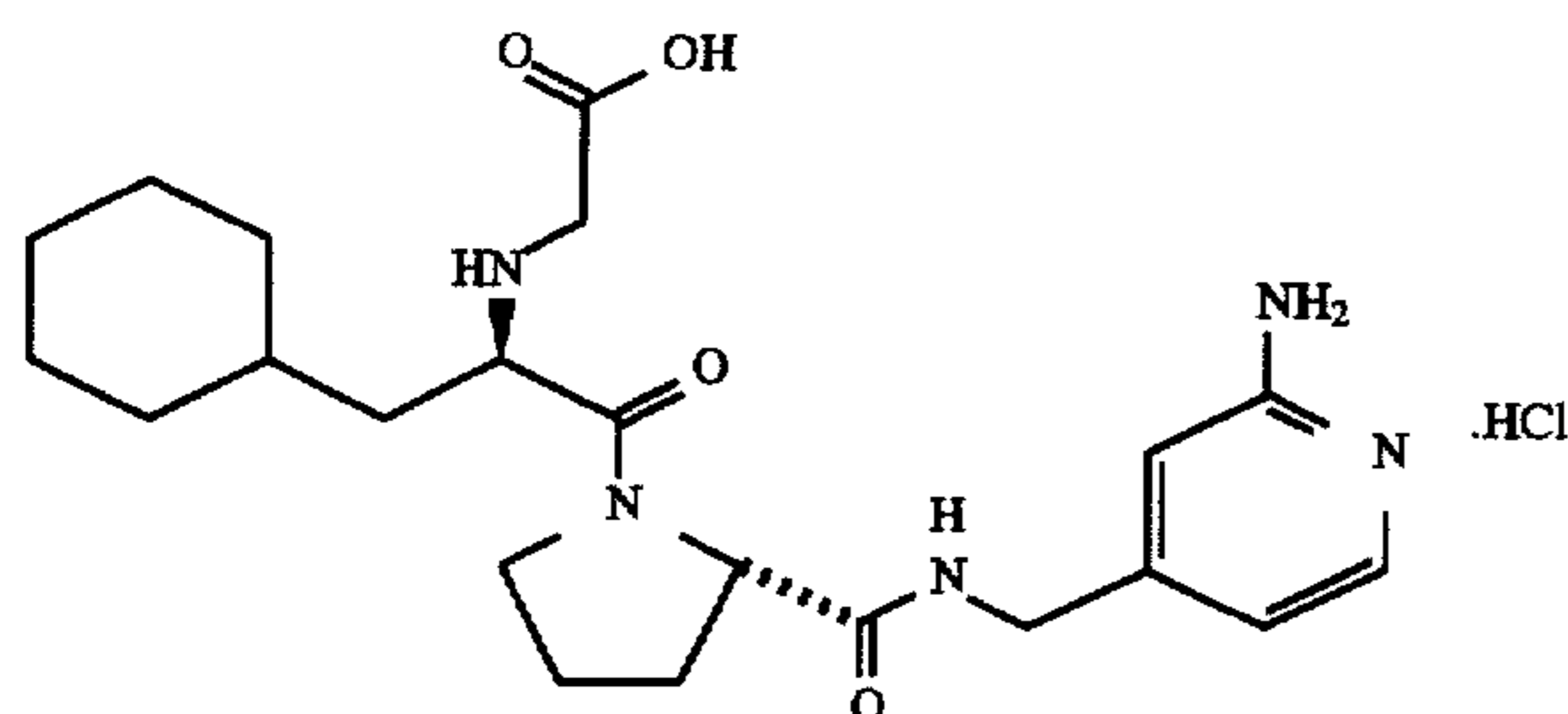
HO 2 CCH 2 -D-Cha-Pro-4-NHCH 2 -2-aminopyridine.HCl
