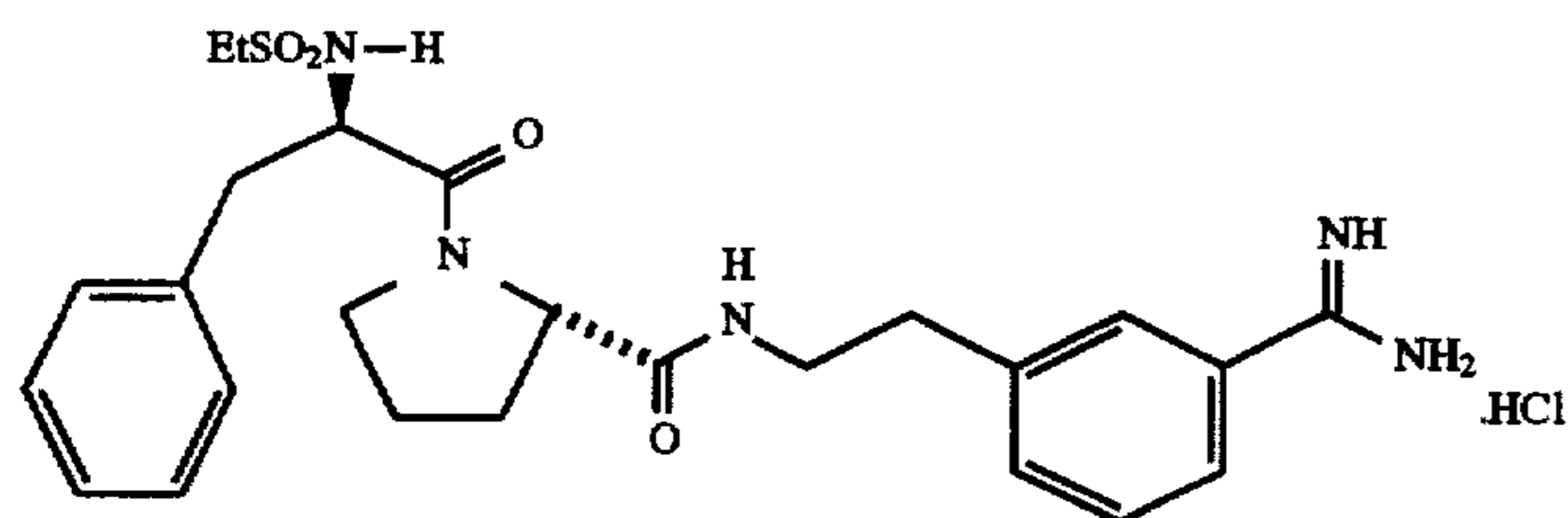
EtSO 2 -D-Phe-Pro-m-NHCH 2 CH 2 -C 6 H 4 C(=NH)NH 2 .HCl
