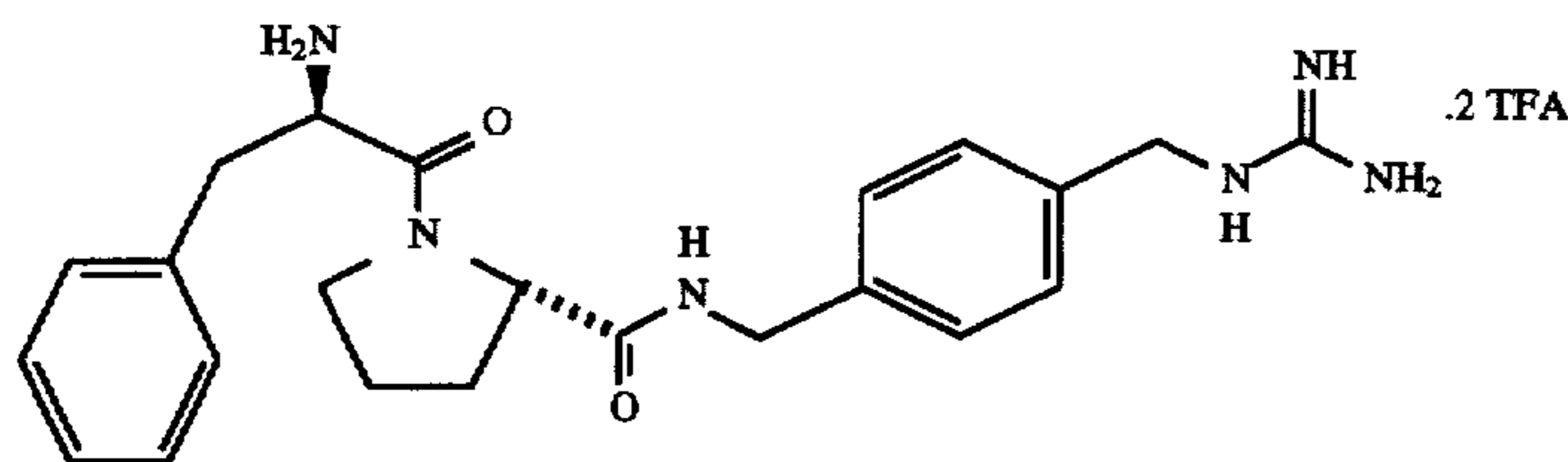
D-Phe-Pro-p-NHCH 2 C 6 H 4 CH 2 NHC(NH)NH 2 .2TFA
