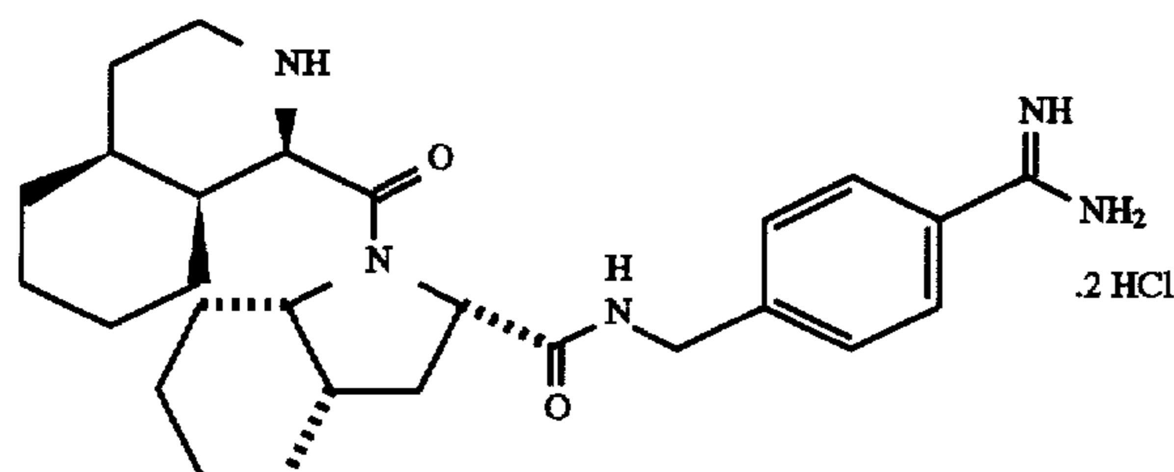
D-1-Piq-cis-Ohi-p-NHCH 2 C 6 H 4 C(NH)NH 2 .2HCl
