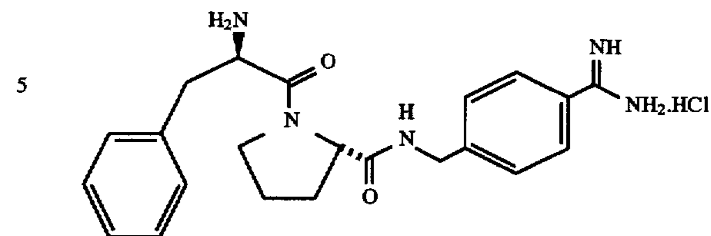
D-Phe-Pro-p-NHCH 2 C 6 H 4 C(NH)NH 2 .HCl
