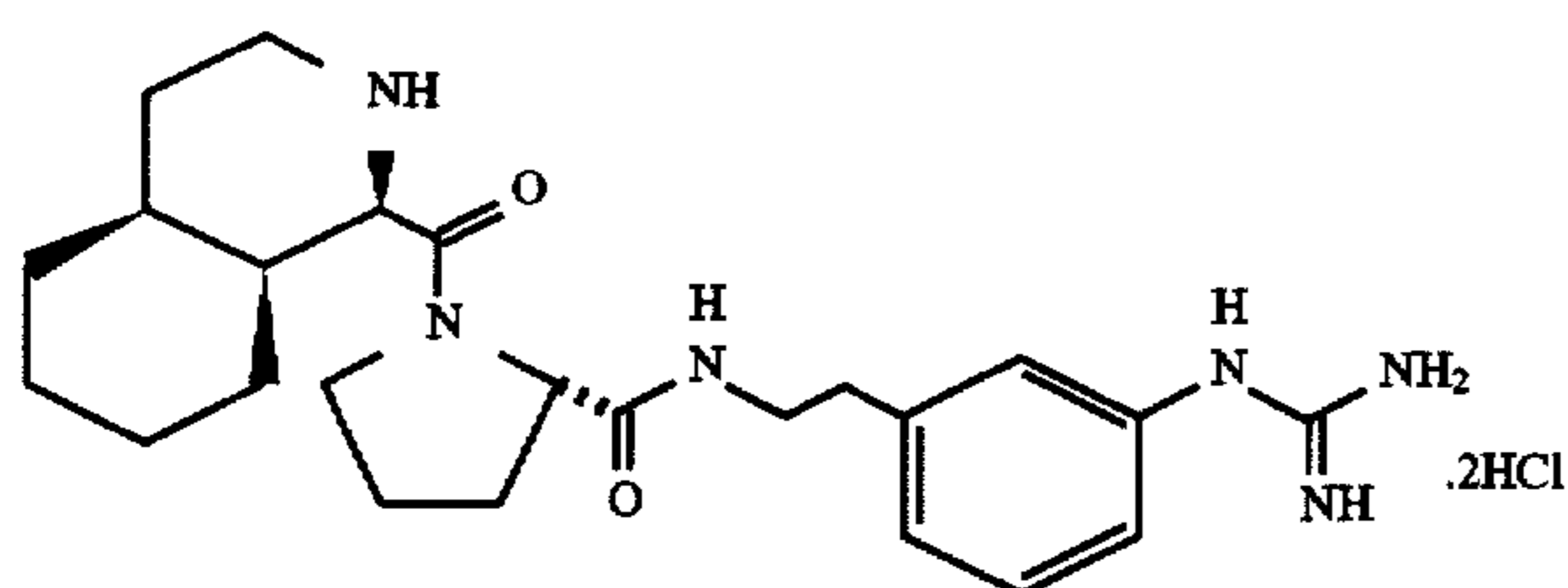
D-1-Piq-Pro-m-NHCH 2 CH 2 C 6 H 4 NHC(NH)NH 2 .2HCl
