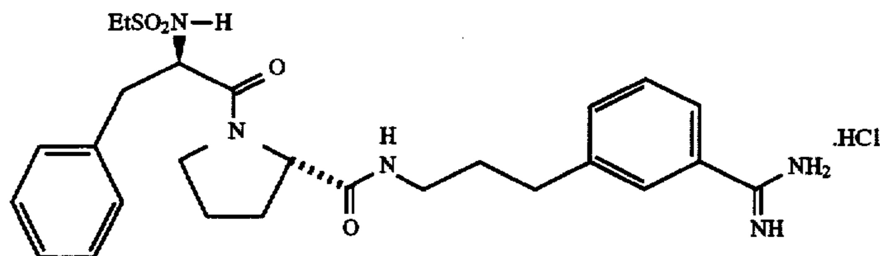
EtSO 2 -D-Phe-Pro-m-NHCH 2 CH 2 CH 2 -C 6 H 4 C(=NH)NH 2 .HCl
