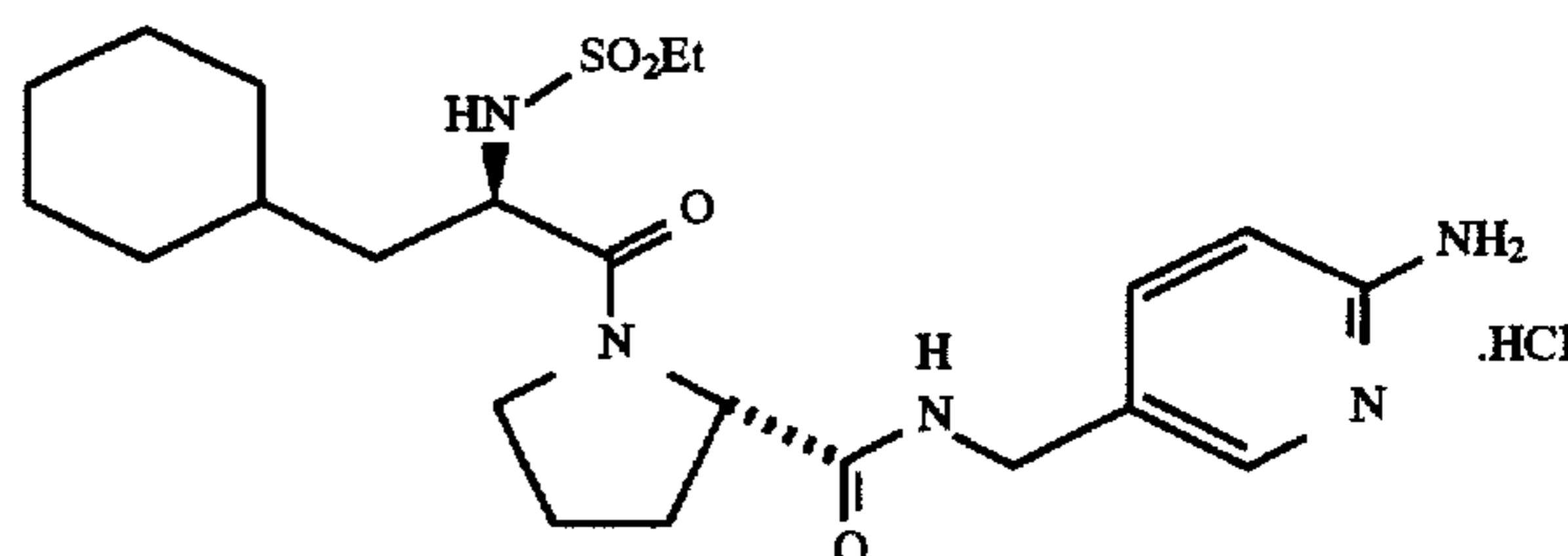
EtSO 2 -D-Cha-Pro-5-NHCH 2 -2-aminopyridine.HCl
