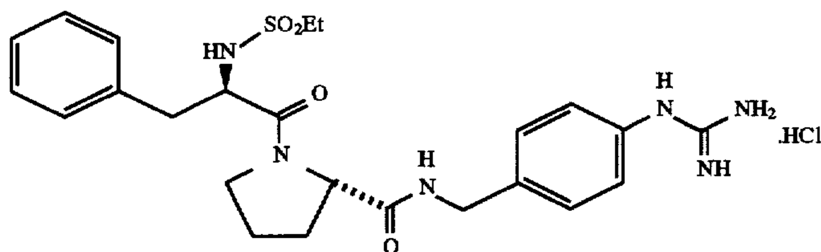
EtSO 2 -D-Phe-Pro-p-NHCH 2 C 6 H 4 NHC(NH)NH 2 .HCl
