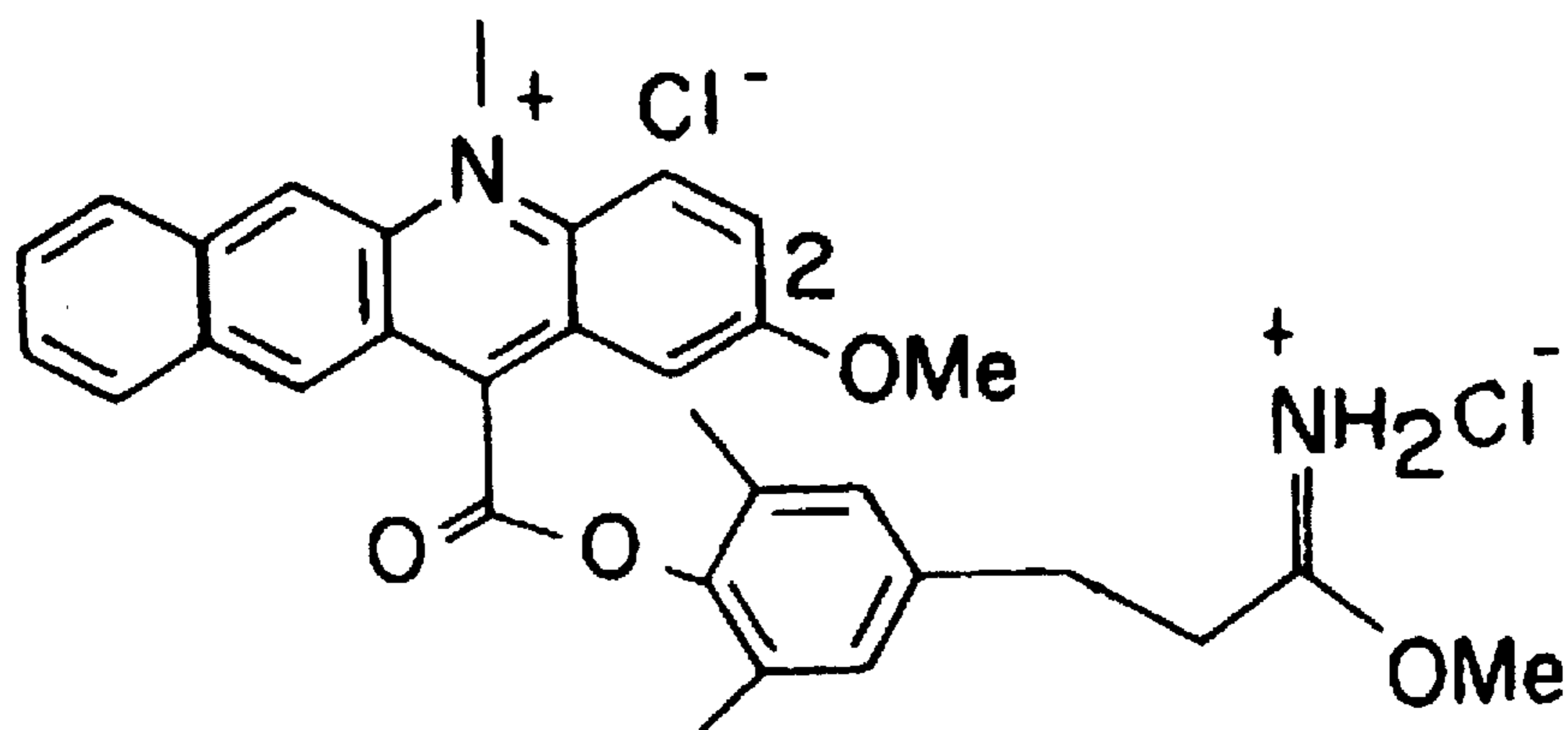
2-MeO-LEAE-Imidate
