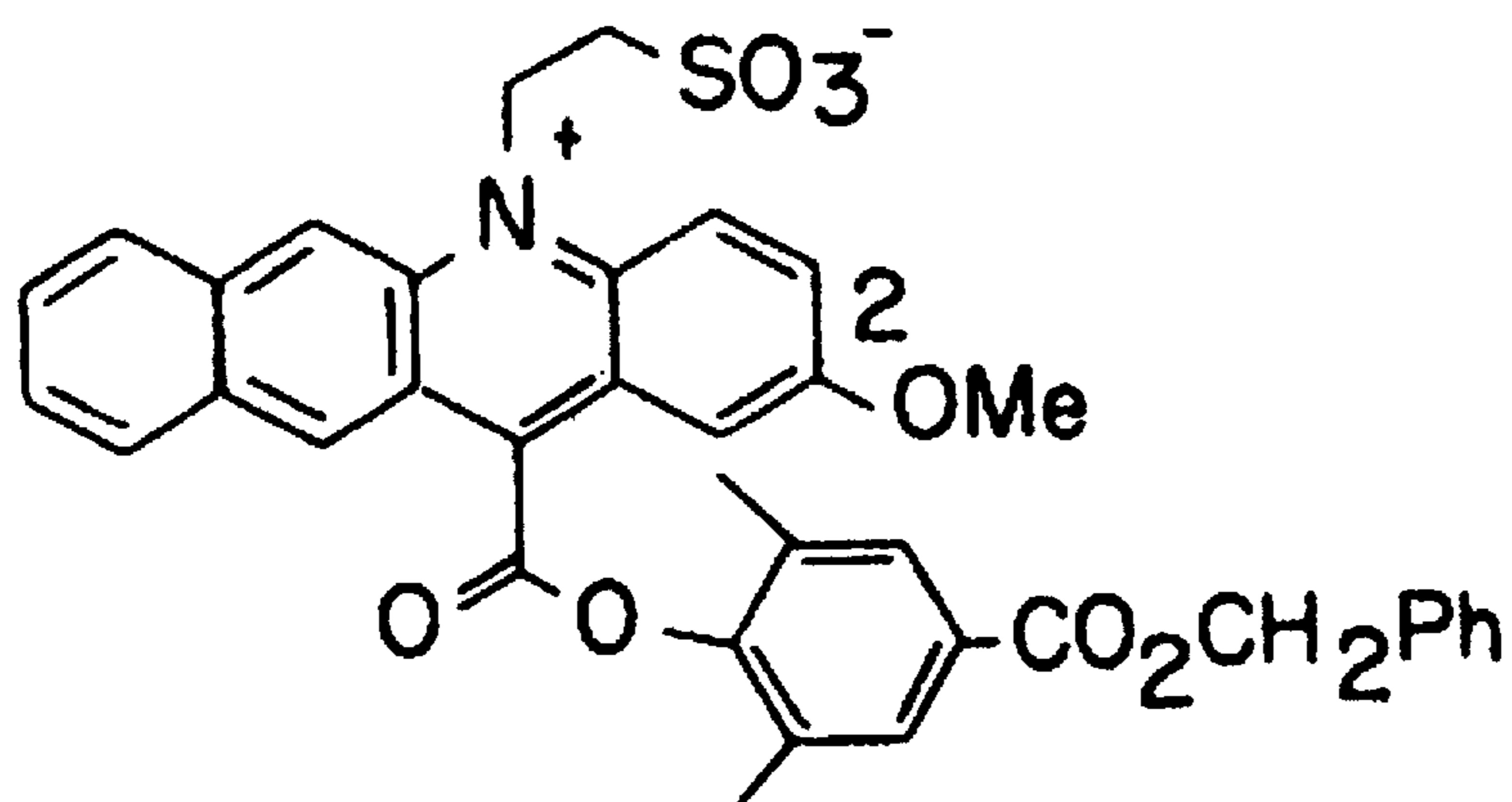
2-MeO-NSE-LEAE-NHS
