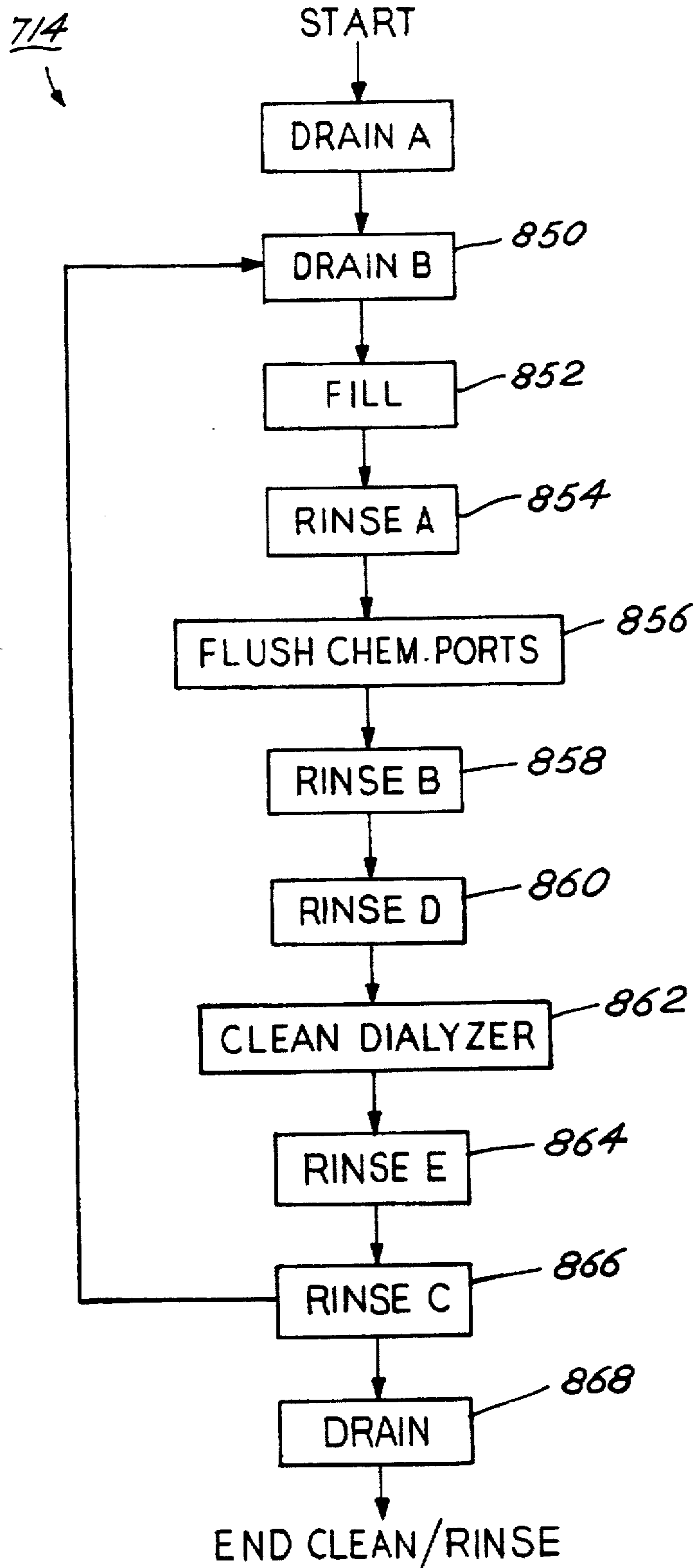
FIG. 23 CLEAN/RINSE
